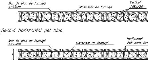
Secció horitzontal per la junta
