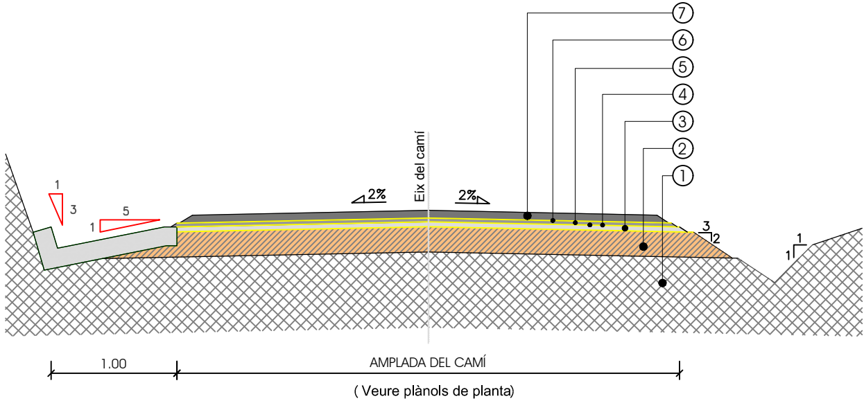
SECCIÓ TIPUS 2.- REFORÇ I REGULARITZACIÓ DE PAVIMENT
