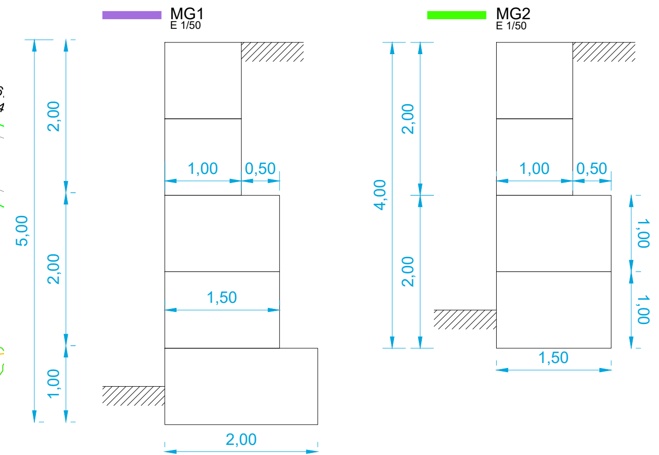
DETALL TIPUS MUR GABIONS E 1/50
