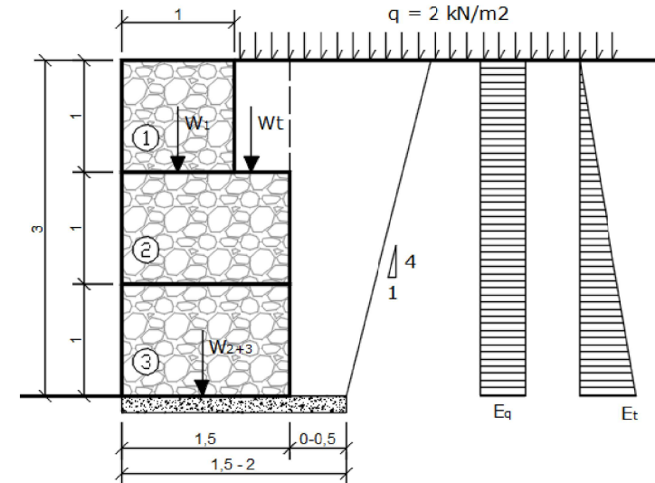
Figura 6.1. Esquema del mur de gabions de 3,0m d'alçada.
