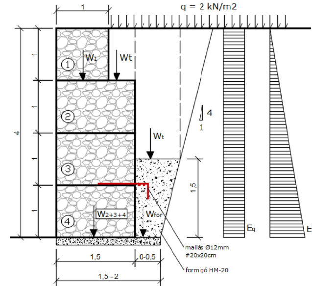
Figura 5.1. Esquema del mur de gabions de 4,0m d'alçada.
