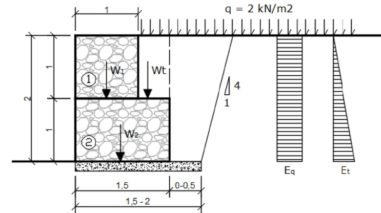
Figura 7.1. Esquema del mur de gabions de 2,0m d'alçada.
