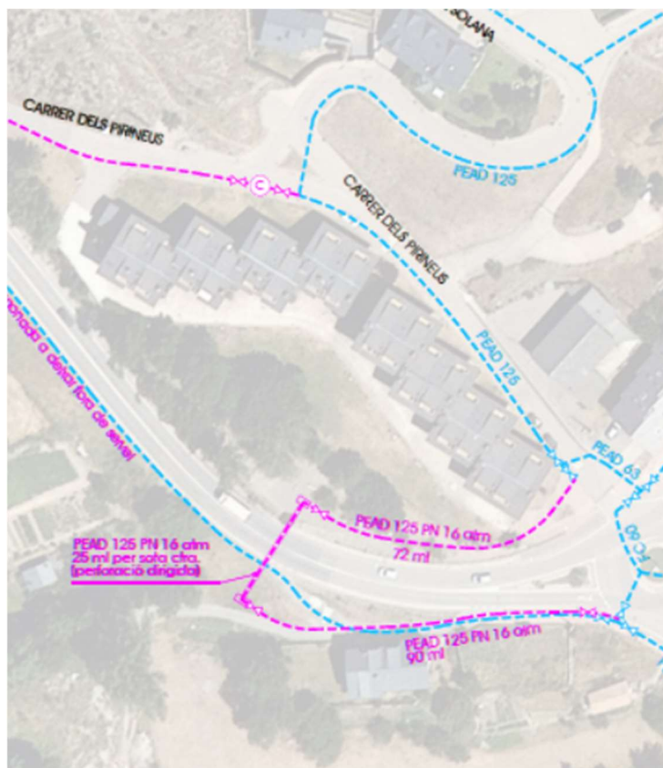
Traçat definitiu a la zona on s'ha platejat dos traçats alternatius per a la canonada
