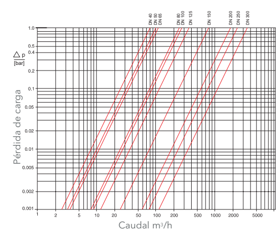
Ábaco tipo de pérdida de carga
