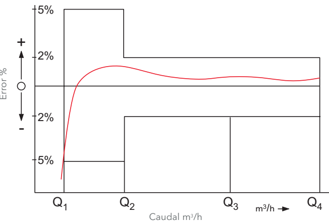
Curva tipo de precisión
