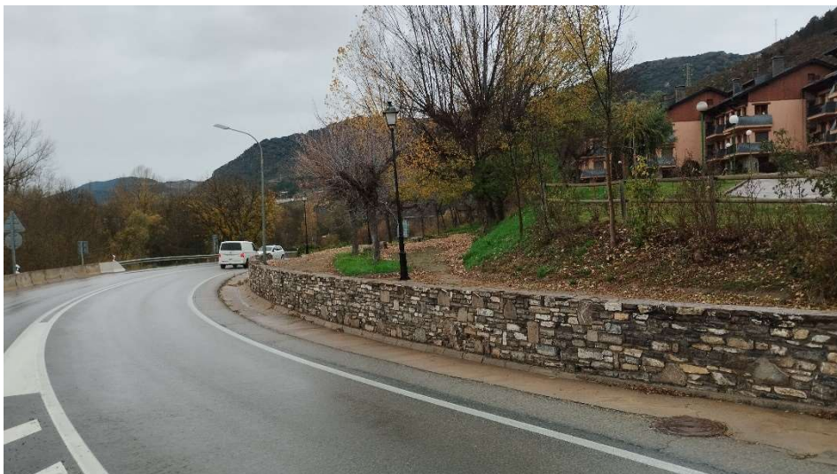
Zona del pas sota la carretera N-260 per perforació horitzontal (mirant a ponent)
