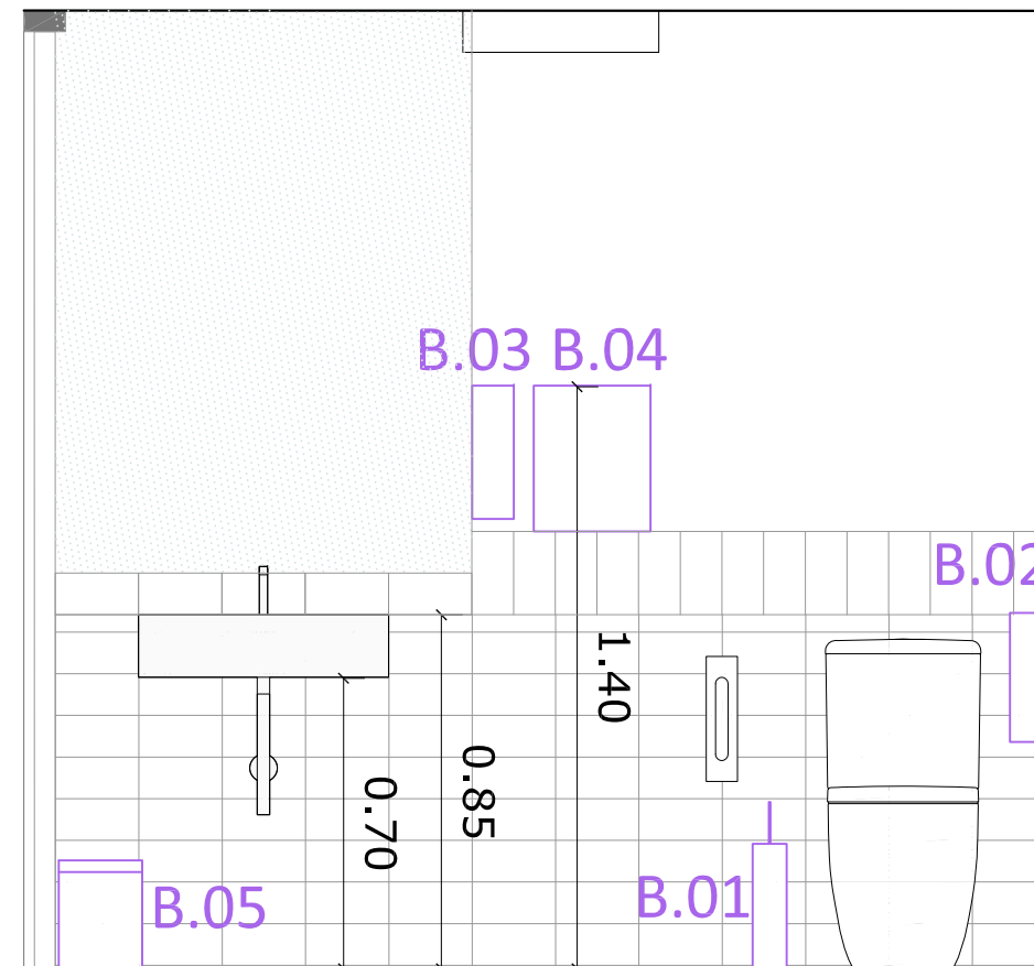
SECCIÓ-ALÇAT S4
