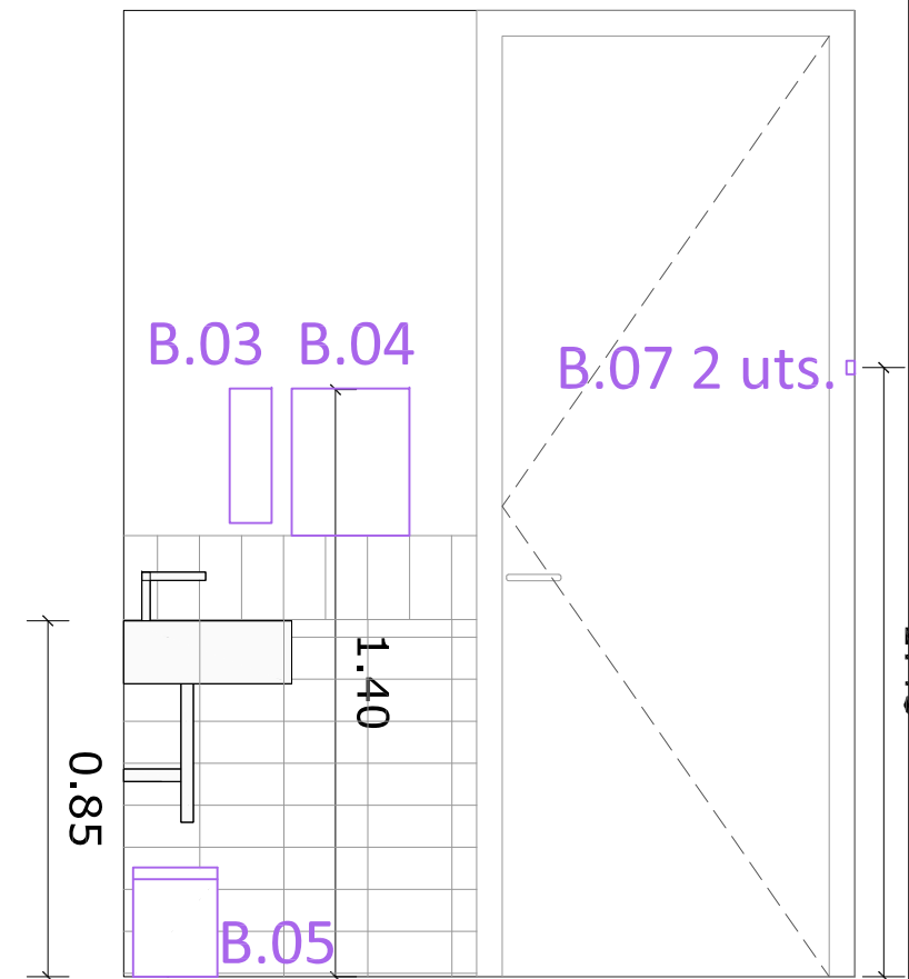
SECCIÓ-ALÇAT S4
