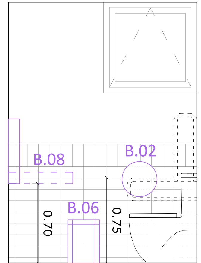
SECCIÓ-ALÇAT S1
