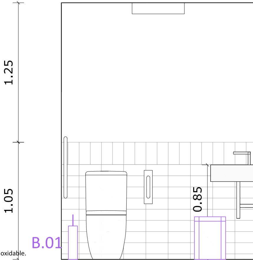
SECCIÓ-ALÇAT S3
