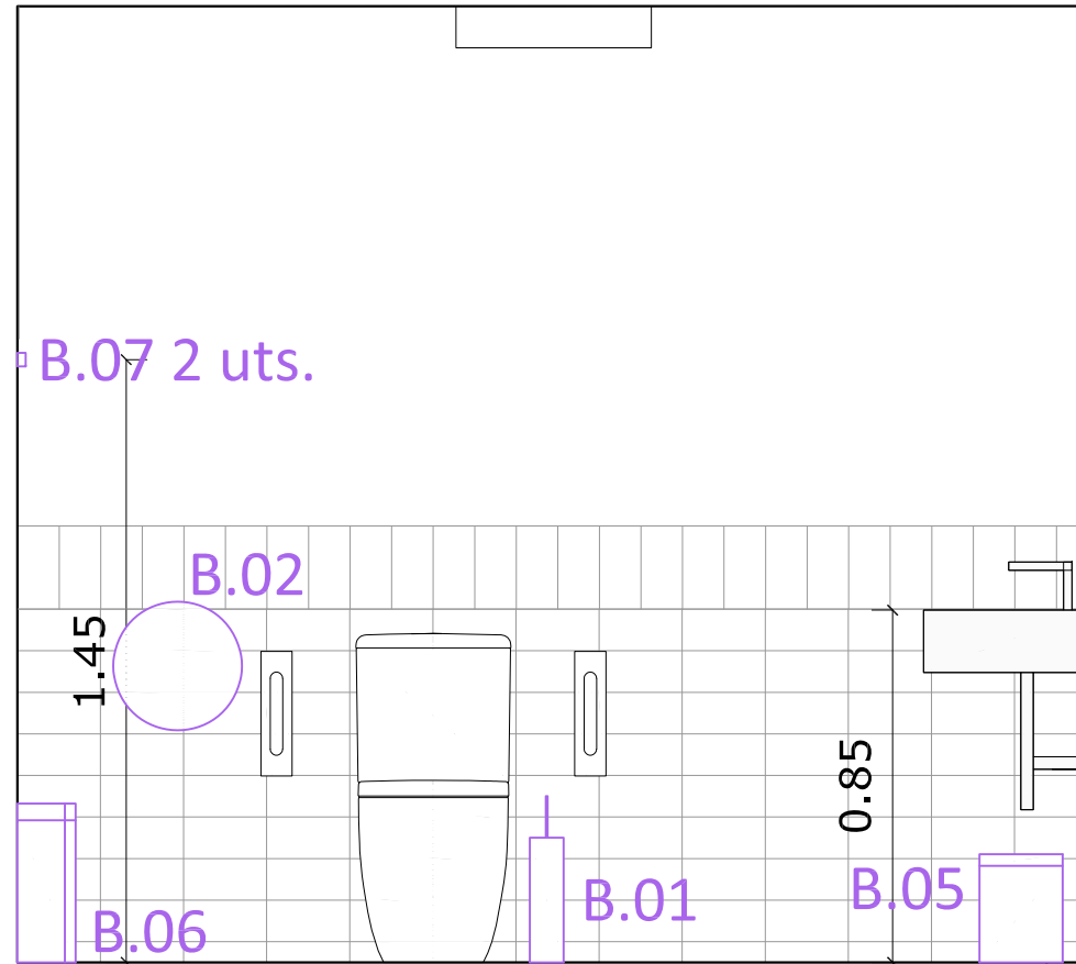
SECCIÓ-ALÇAT S3
