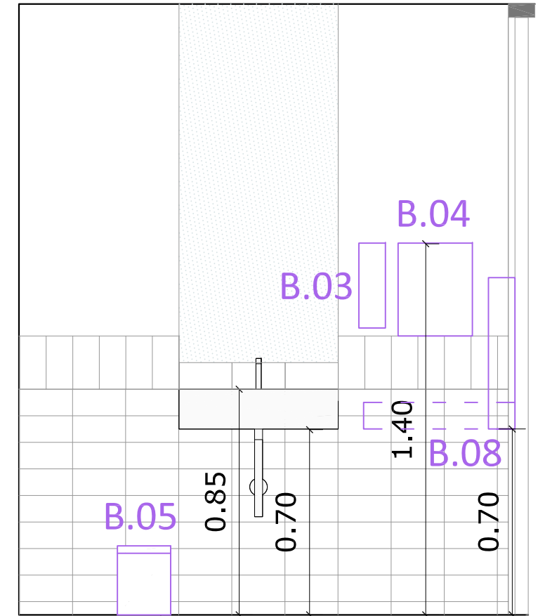
SECCIÓ-ALÇAT S2
