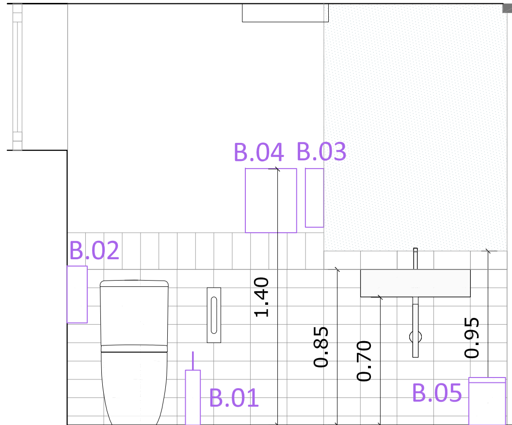
SECCIÓ-ALÇAT S3
