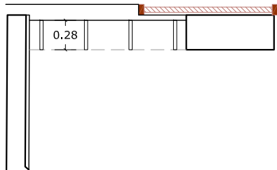
LLEIXES D'EMMAGATZEMATGE 1 (M.03) Dimensions: 148 x 28 cm Unitats: 1 Lleixes en tauler contraxapat de bedoll (e=18mm) i xapades en fòrmica. Color a decidir per DO.
