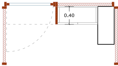
ARMARI AMB CLAU 2 (M.02) Dimensions: 230 x 89 x 40 cm Unitats: 1 Armari (amb clau) en tauler contraxapat de bedoll (e=18mm). Lleixes xapades en fòrmica (<0,7mm.) per seva cara superior. Color a decidir per DO. Tiradors en acer inox mat, panys i ferratges inclosos.
