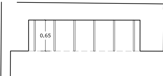
LLEIXES D'EMMAGATZEMATGE 2 (M.04) Dimensions: 236 x 65 cm Lleixes en tauler carrosser de 30mm. (tauler contraxapat) Disposades sobre carteles ancorades a carrils verticals d'acer collats al mur. 1 unitat - conté 3 lleixes Dimensions de cada lleixa: 236 x 65cm.
