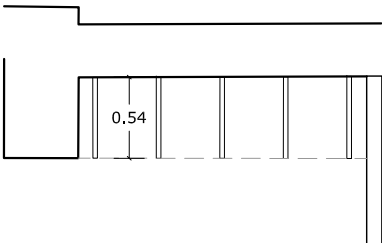
LLEIXES D'EMMAGATZEMATGE 3 (M.05) Dimensions: 190 x 54 cm Lleixes en tauler carrosser de 30mm. (tauler contraxapat) Disposades sobre carteles ancorades a carrils verticals d'acer collats al mur. 1 unitat - conté 3 lleixes Dimensions de cada lleixa: 190 x 54cm.
