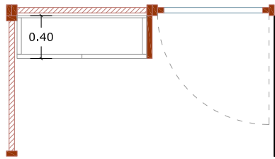
ARMARI AMB CLAU 1 (M.01) Dimensions: 230 x 121 x 40 cm Unitats: 1 Armari (amb clau) en tauler contraxapat de bedoll (e=18mm). Lleixes xapades en fòrmica (<0,7mm.) per seva cara superior. Color a decidir per DO. Tiradors en acer inox mat, panys i ferratges inclosos.
