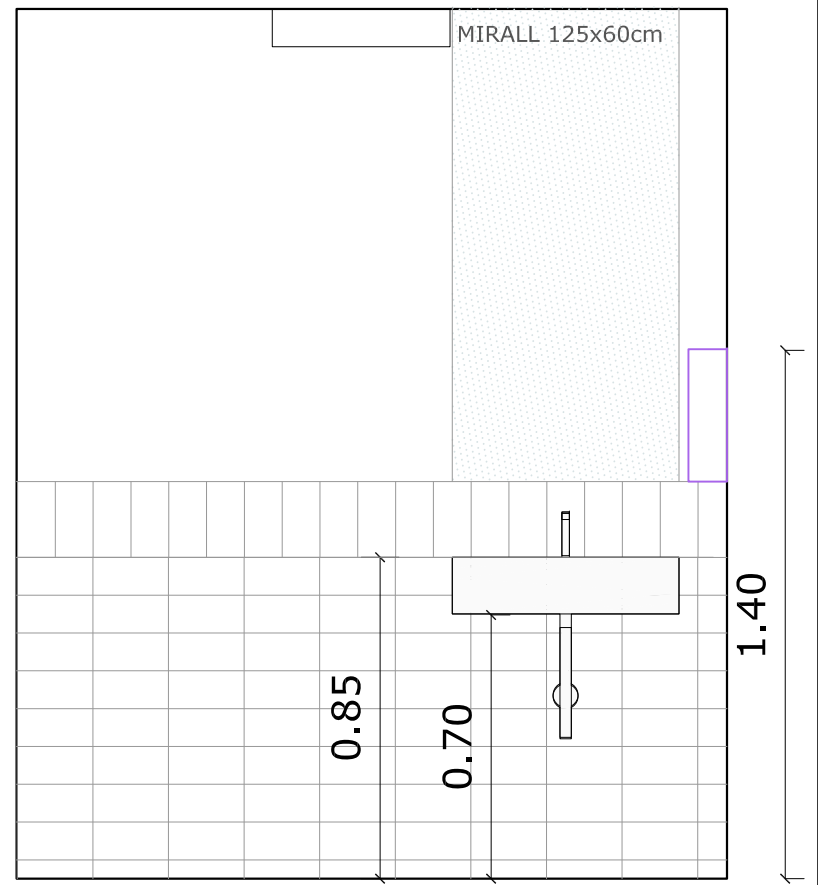
SECCIÓ-ALÇAT S2
