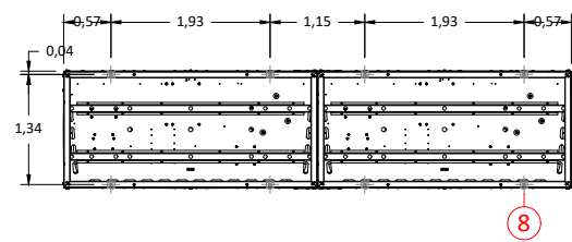
DISPOSICIÓ DE FORATS DE MUNTATGE
