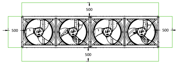
ESPAI MÍNIM DE MANTENIMENT
