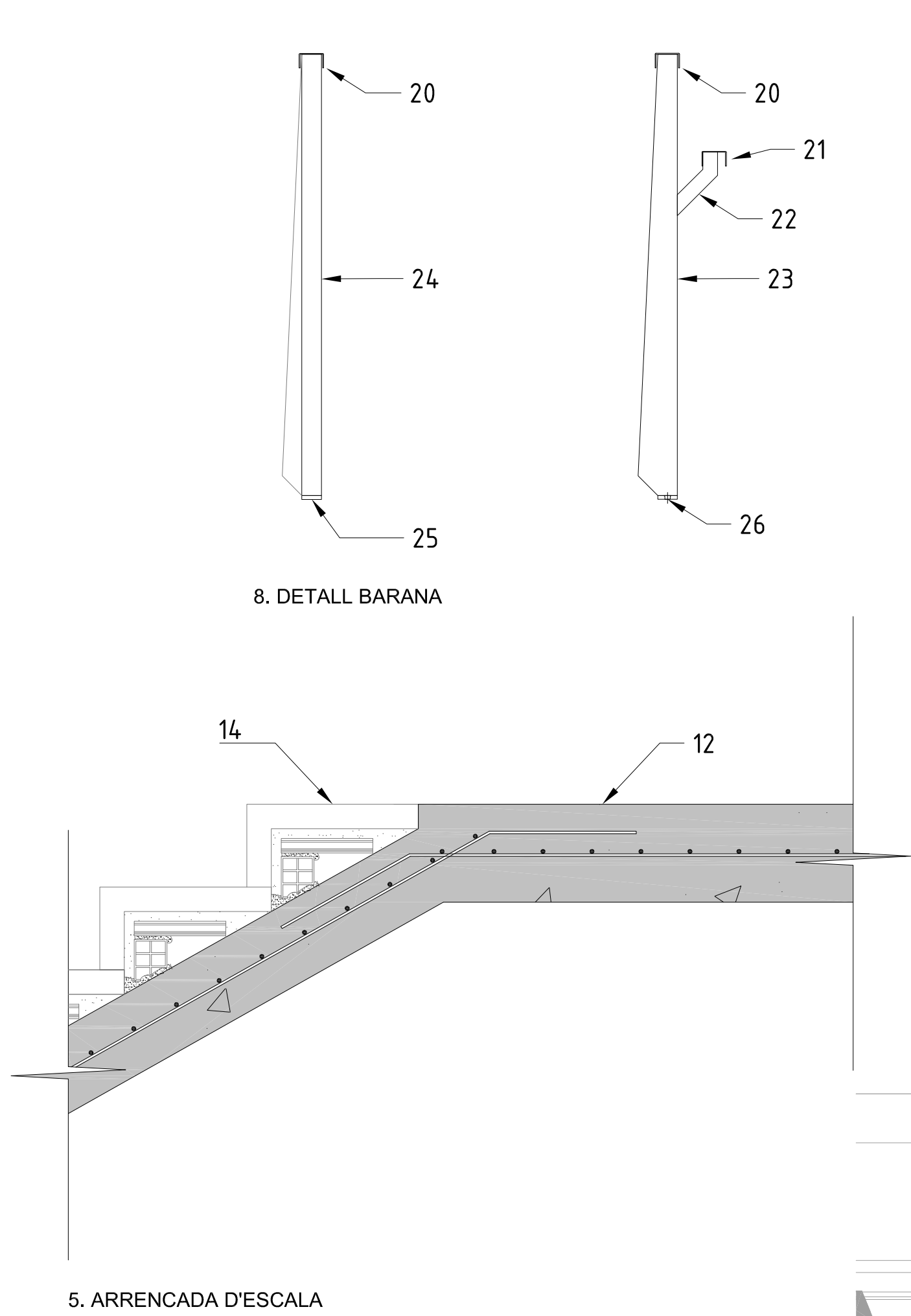
5. ARRENCADA D'ESCALA
