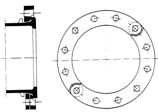
Brida orientable
