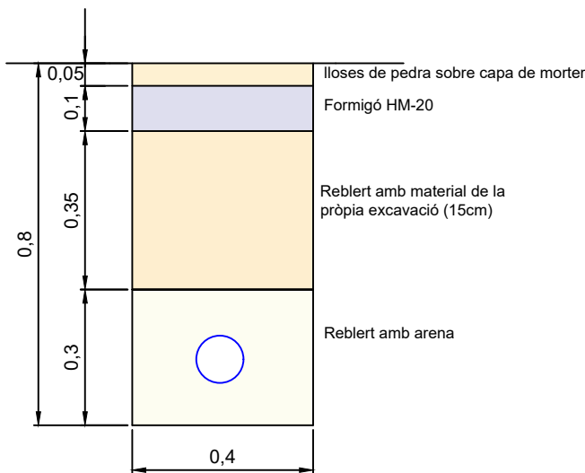
Detall rasa aigua potable en paviment de lloses de pedra
