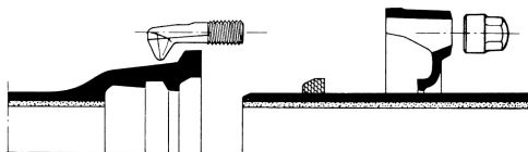
Junta mecànica
