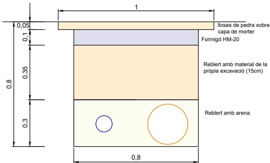
Detall rasa aigua potable i clavegueram en paviment de lloses de pedra
