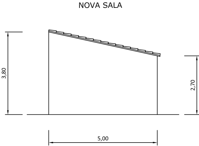
ALÇAT LATERAL DRET
