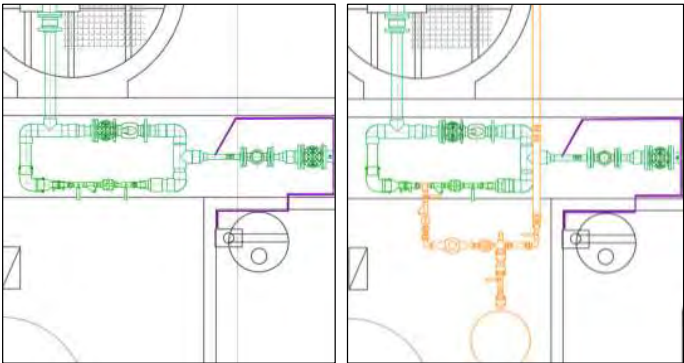
Figura 10. Estat actual (esquerra) i proposta (dreta) del pou Palaudàries.
