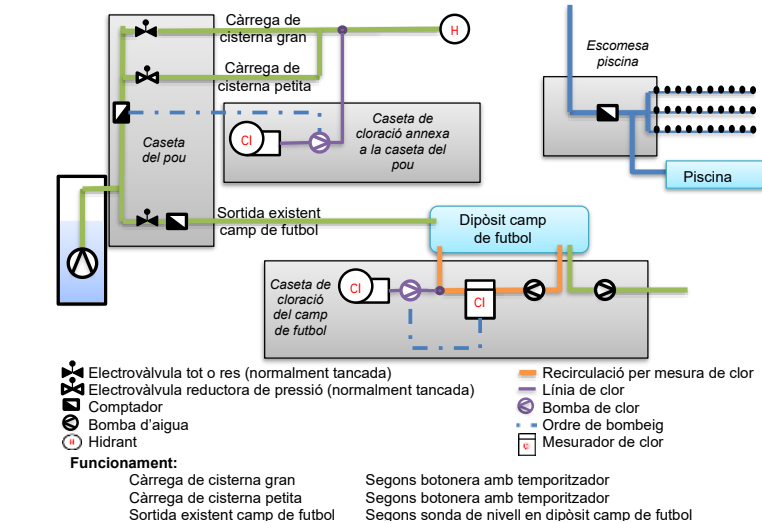
Figura 6. Esquema de funcionament actual del pou Piscines.
