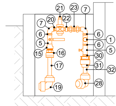
SECCIÓ B-B'
