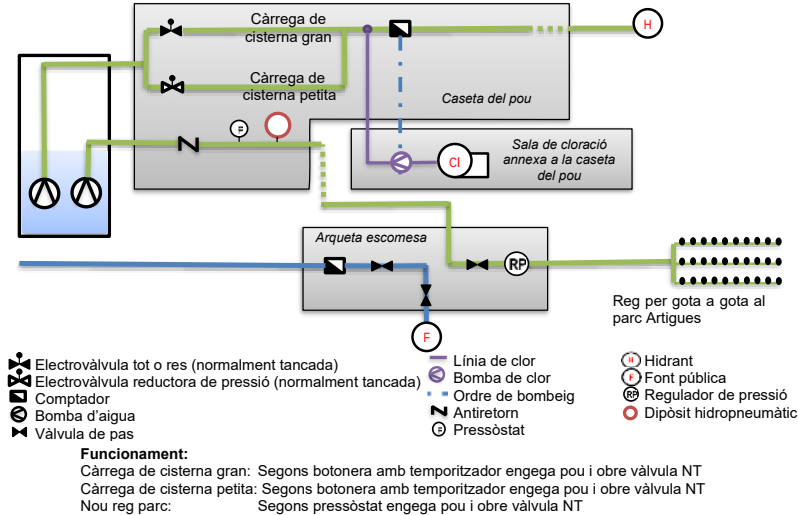
Figura 8. Esquema de funcionament proposat del pou Artigues.
