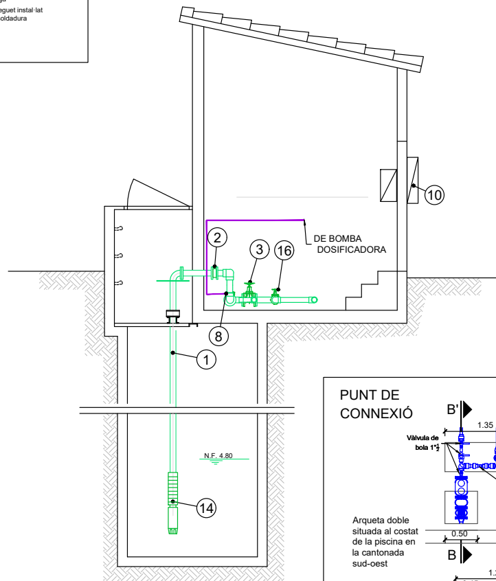
SECCIÓ B-B'
