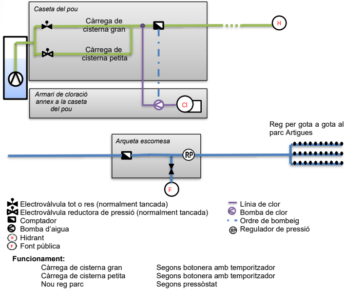
Figura 1. Esquema de funcionament actual del pou Artigues.
