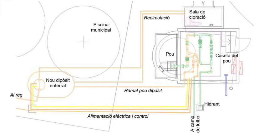
Figura 15. Esquema pou piscines dipòsit enterrat.
