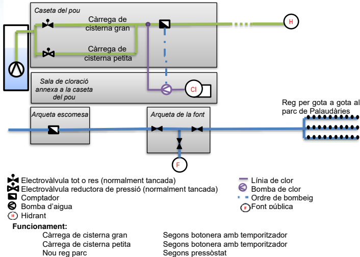
Figura 4. Esquema de funcionament actual del pou Palaudàries.
