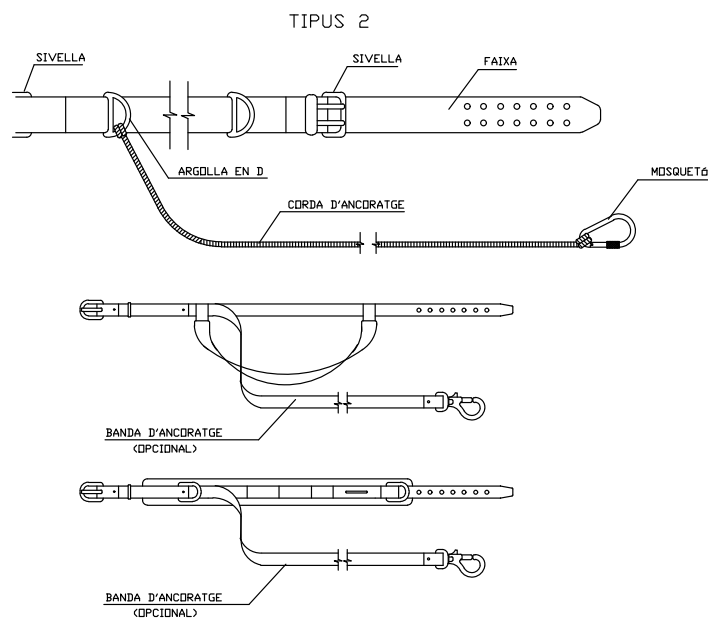
CINTURONS D'ANCORATGE
