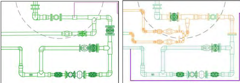
Figura 14. Estat actual (esquerra) i proposta (dreta) dels ramals de l'interior de la caseta del pou Piscines.
