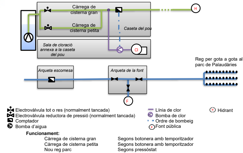
Figura 4. Esquema de funcionament actual del pou Palaudàries.
