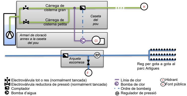
Figura 2. Esquema de funcionament actual del pou Artigues.
