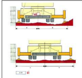
Urbanisme: maquinària d'obra. Grues: col·locació estabilitzadors
