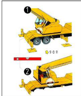
Urbanisme: maquinària d'obra. Grues: control de nivell
