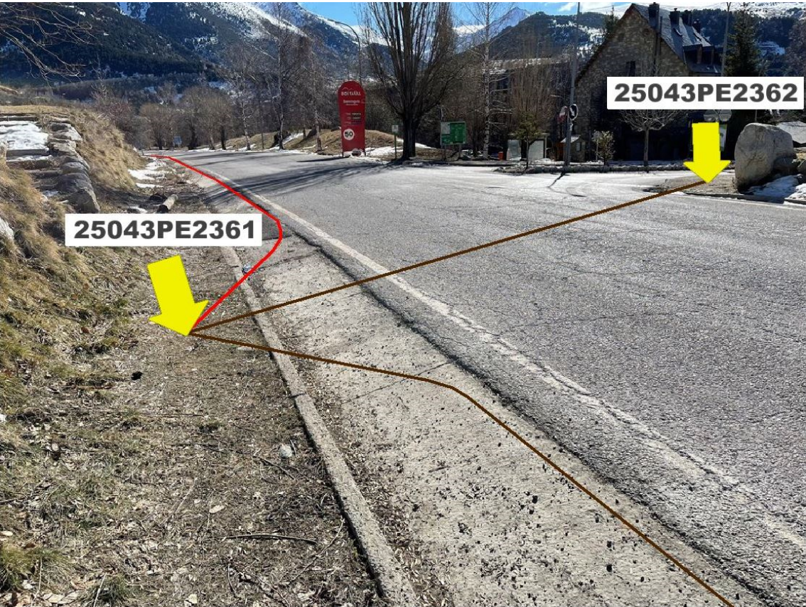
Fig 1.2.4.2.1. Inici de l'estesa de FO al pericó projectat 25043PE2362 i inici de l'obra civil al pericó projectat 25043PE2361.
