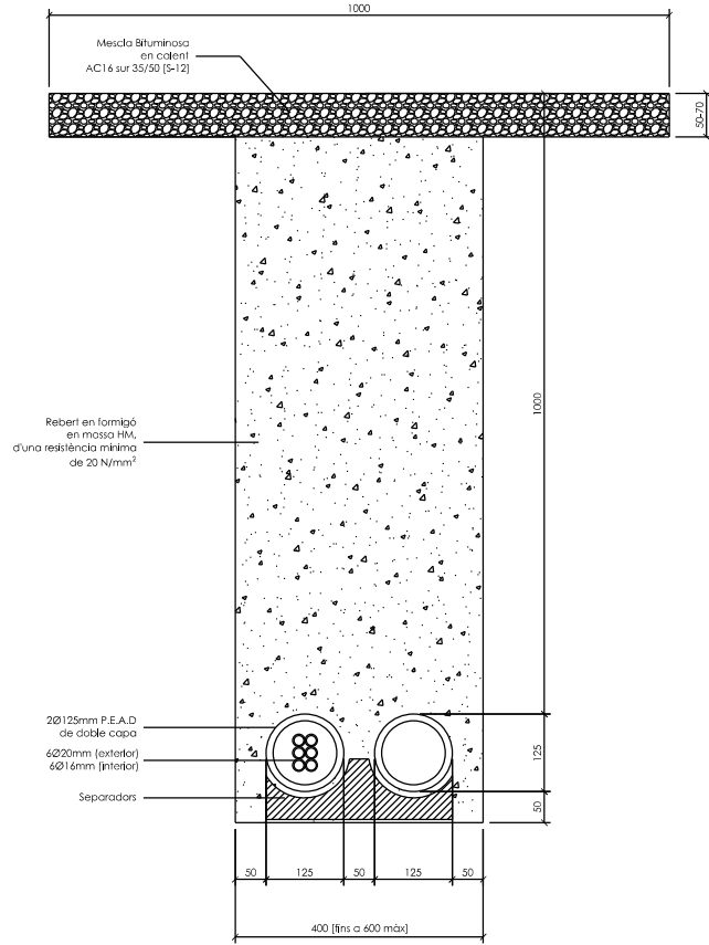
CANALITZACIÓ CONVENCIONAL DE 2Ø125mm EN BASE 2 EN CREUAMENTS DE CARRETERES [ST-6]
