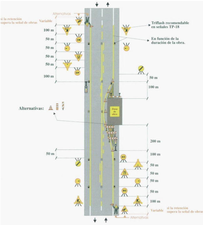
Fig 1.2.3.5.c. Exemple de senyalització.
