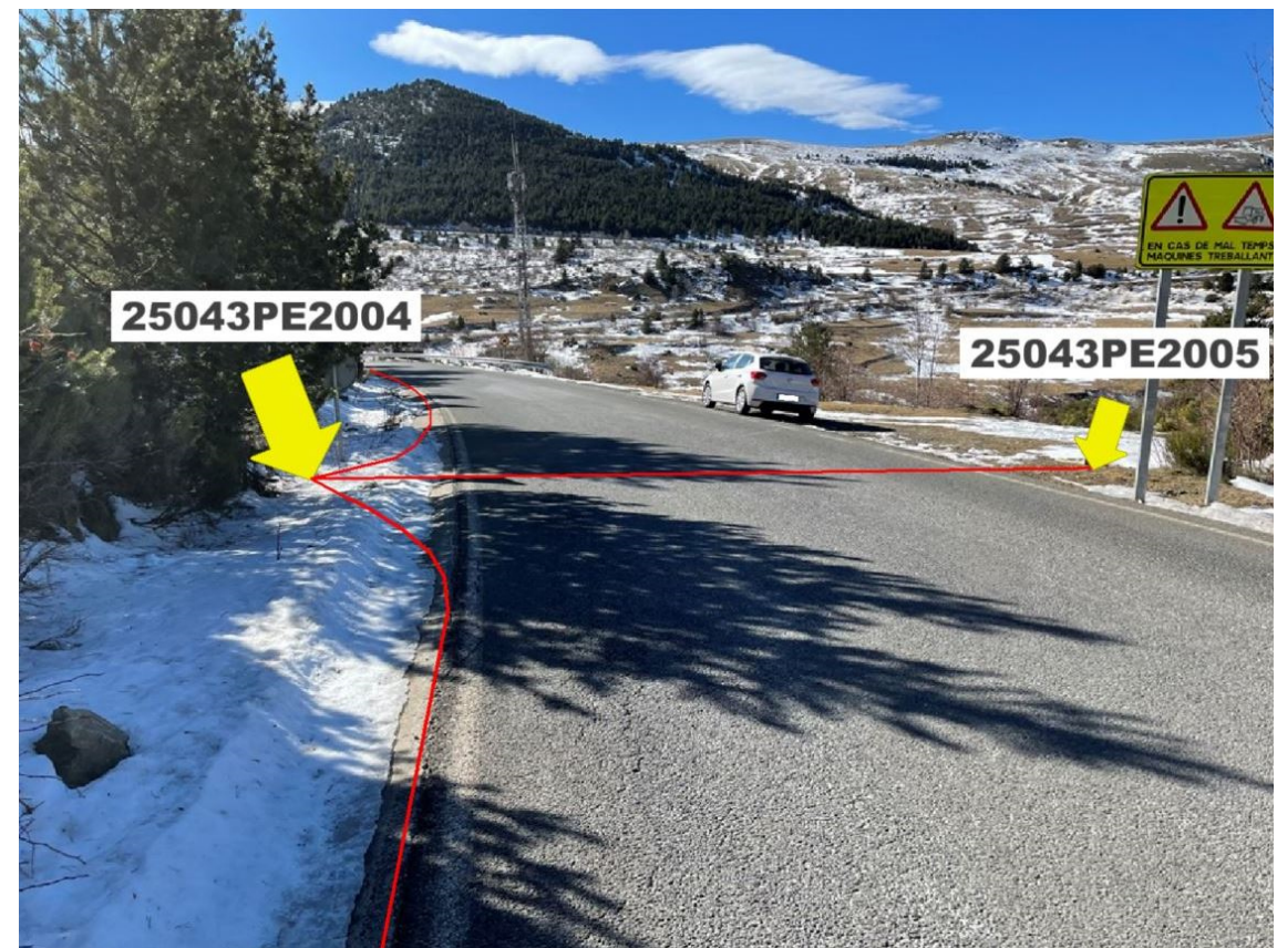
Fig 1.2.4.2.13. Ubicació dels nous pericons 25043PE2004 i 25043PE2005. Encreuament.
