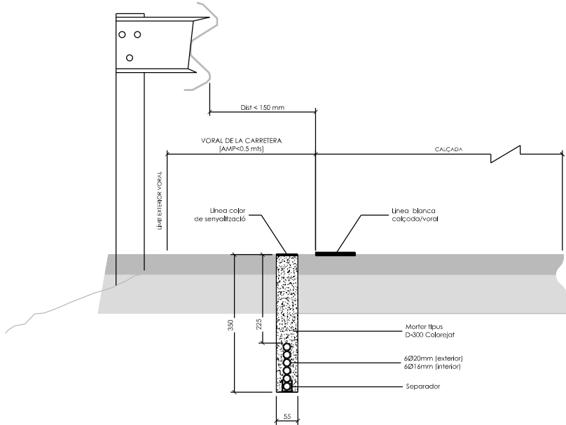
CANALITZACIÓ EN MICRORASA DE 6Ø20mm BASE 1 EN CALÇADA AMB BIONA [ST4]
