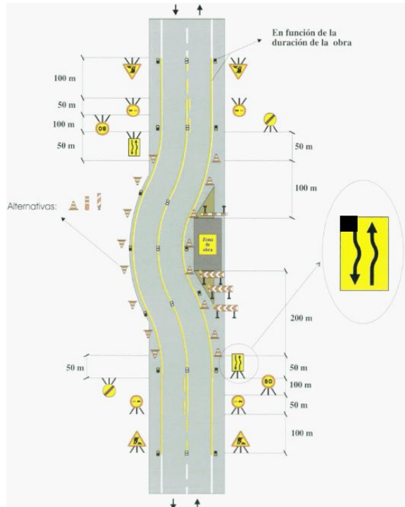
Fig 1.2.3.5.b. Exemple de senyalització.
