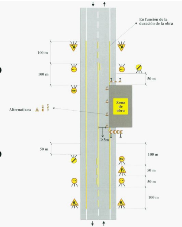
Fig 1.2.3.5.a. Exemple de senyalització.
