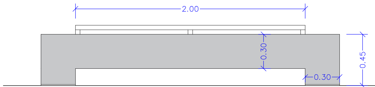
ALÇAT FRONTAL
