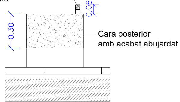
SECCIÓ 2
