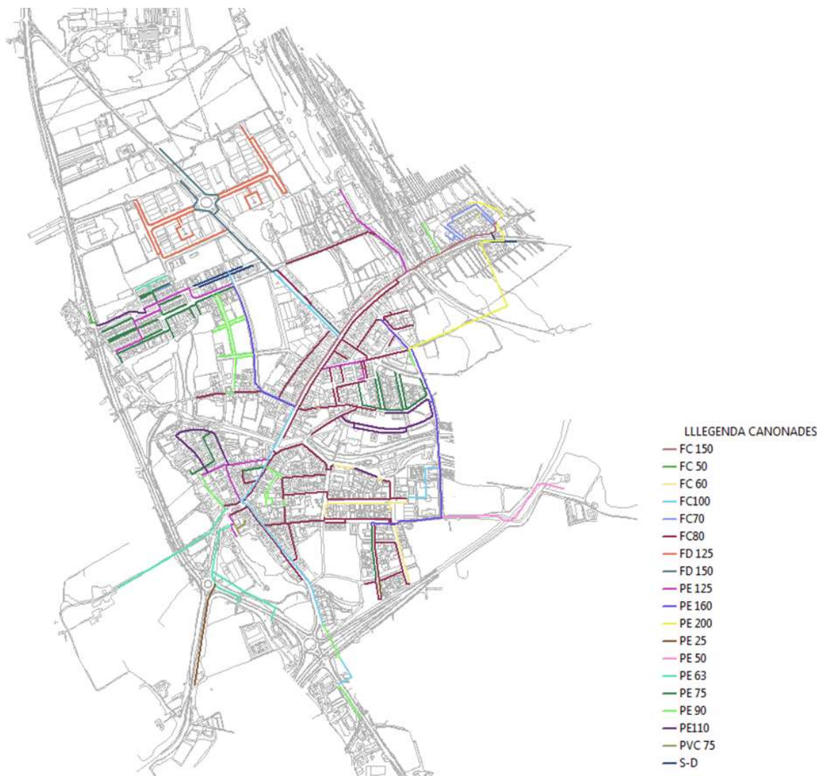
Figura núm.2 Xarxa de distribució d'abastament de Móra la Nova (font: Pla Director Abastament 2019)
