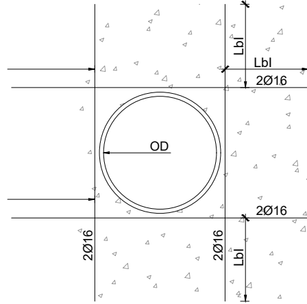
DETALL 1. REFORÇ ARMAT EN MUR -BUILT CANONADA-
