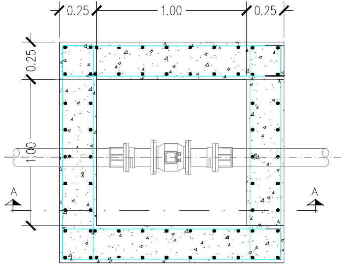
PLANTA ESCALA 1:25
