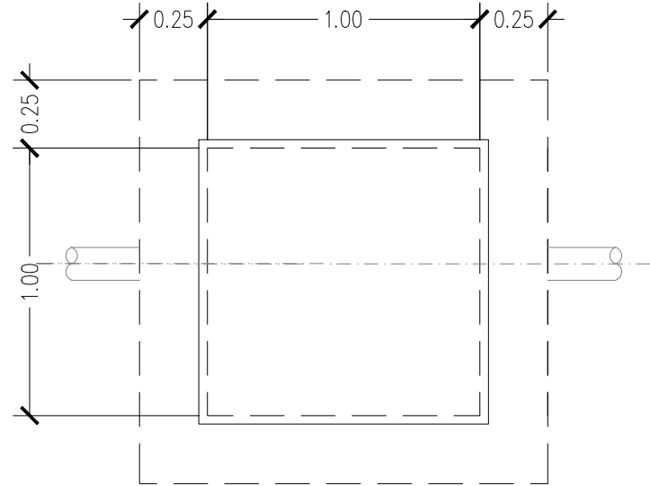
PLANTA COBERTA ESCALA 1:25
