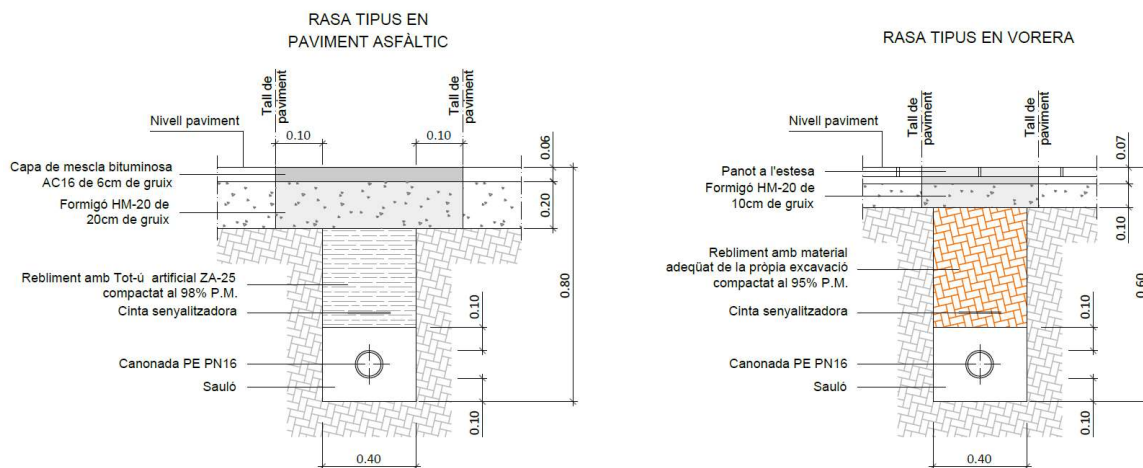
Figura 7. Secció tipus en vorera i calçada
