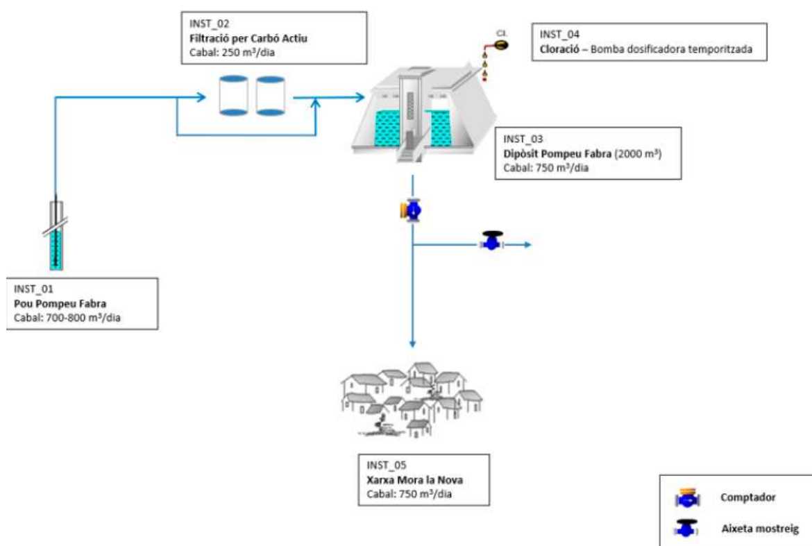
Figura núm.1 Esquema hidràulic de l'abastament a Móra la Nova
