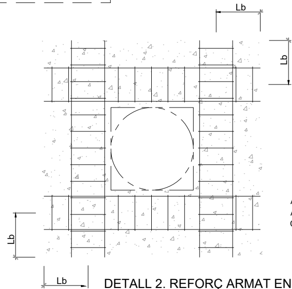
DETALL 2. REFORÇ ARMAT EN SOSTRE -BUILT TAPA ACCÉS-
