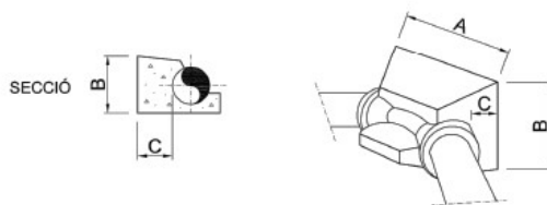
Figura 9. Massissos d'ancoratge per a colzes
