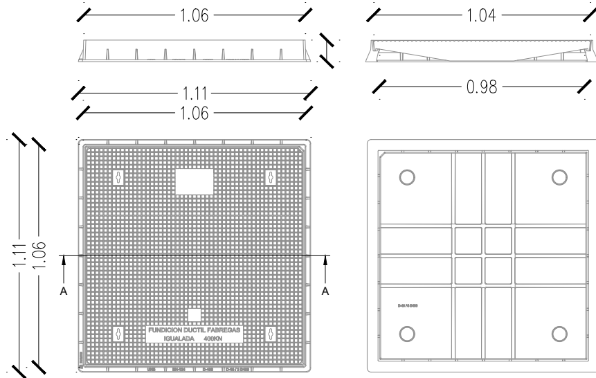
DETALL 3. TAPA
