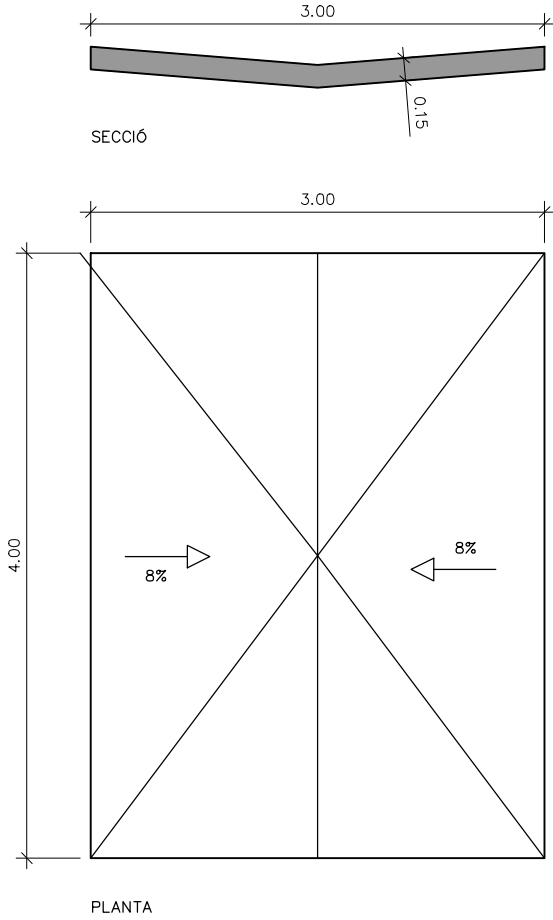
TRECANT D'AIGÜES DE FORMIGÓ E:1/50
