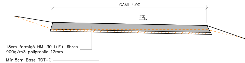
SECCIÓ TIPUS CAMÍ (formigó)
