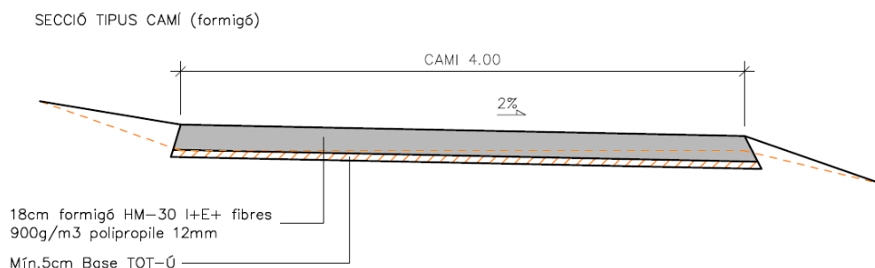
Il·lustració 13. vista secció tipus tram 1.1.
