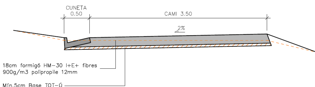
Il·lustració 14. vista secció tipus tram 1.1 amb cuneta.
