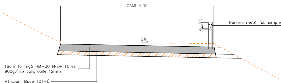
Il·lustració 15. vista secció tipus, tram 1.1 amb biona
