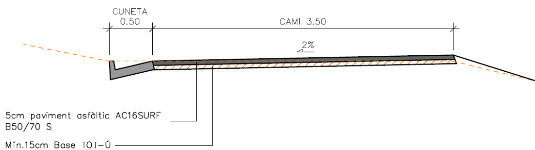
Il·lustració 6. vista secció tipus tram 1.2. amb cuneta
