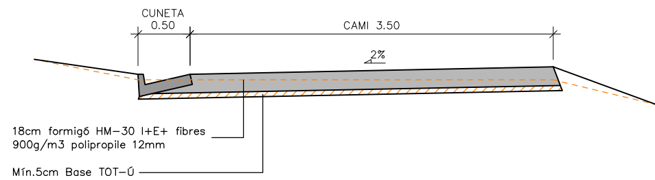
SECCIÓ TIPUS CAMÍ + CUNETA TTR-50 (formigó)
