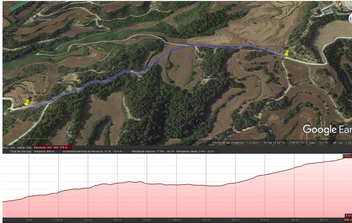
Il·lustració 6. vista secció 0+600.
