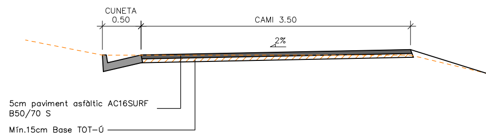
SECCIÓ TIPUS CAMÍ + CUNETA TTR-50 (asfalt)
