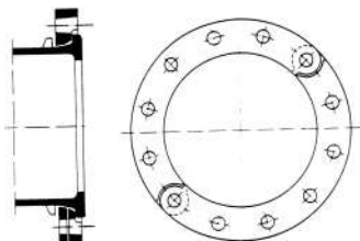
Brida orientable
