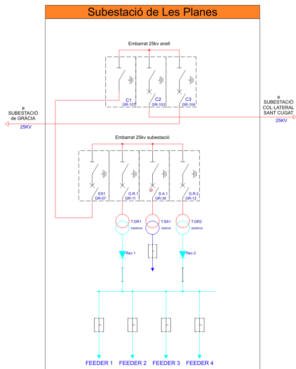
Fig 3 Nou esquema unifilar simplificat de la subestació.
