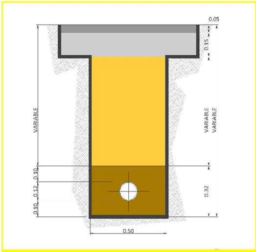
Detall de secció tipus
