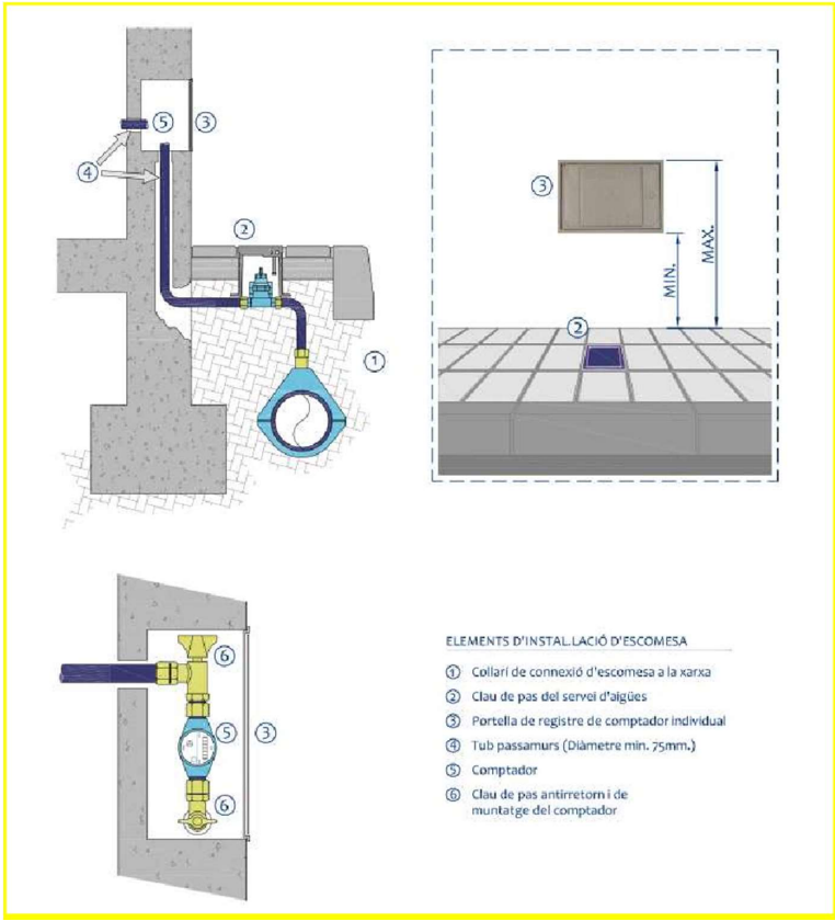
Detall d'escamesa tipus
