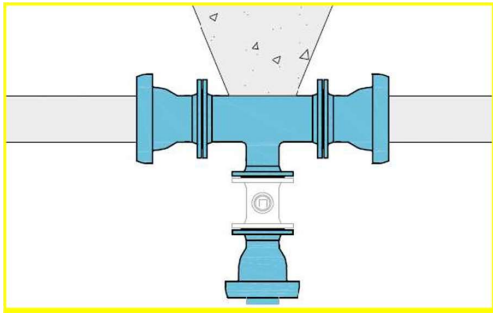
Detall de connexió tipus
