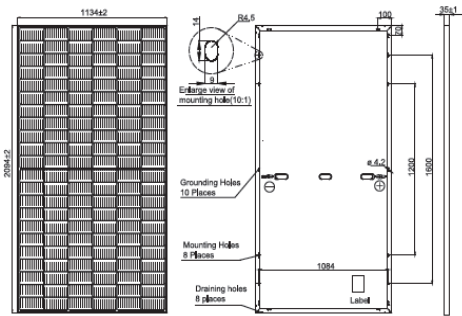
Figura 3. Panell fotovoltaic
