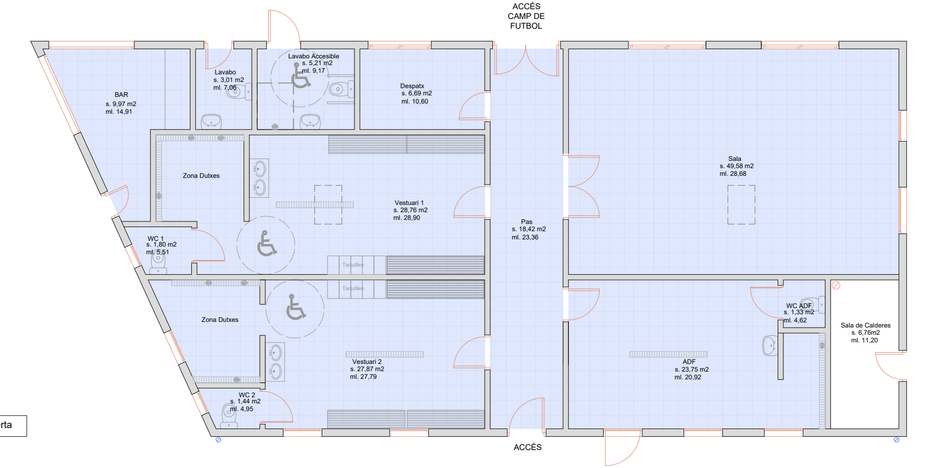
ESTAT REFORMAT - PLANTA BAIXA
