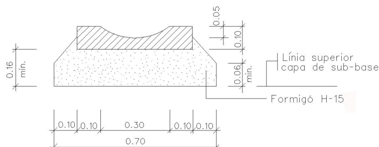
Canaleta prefabricada de formigó
