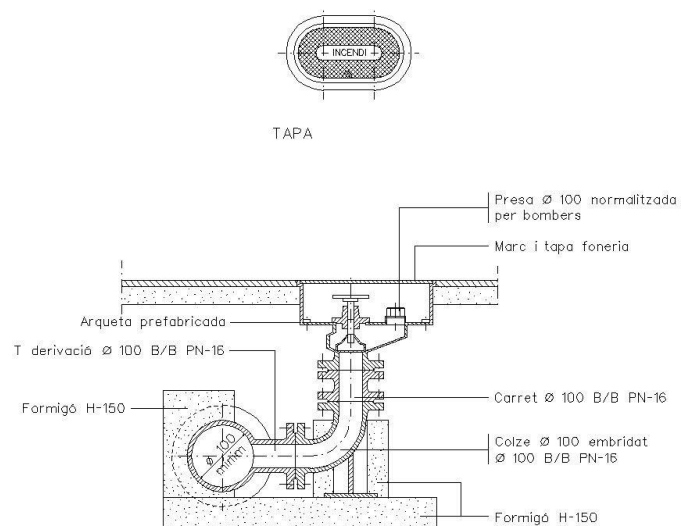
Hidrant soterrat
