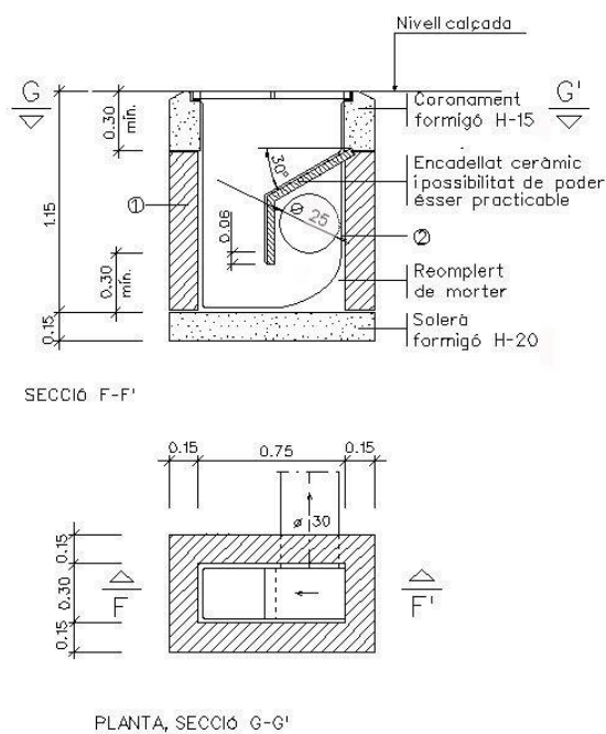
Embornal sifònic " in situ "
