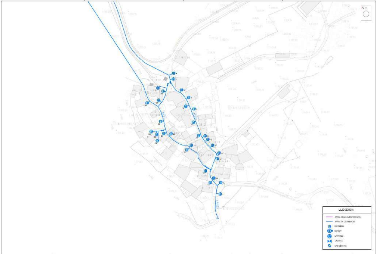
Figura 13. Detall del nucli de Travesseres a partir de l’inventari efectuat durant el treball de camp
