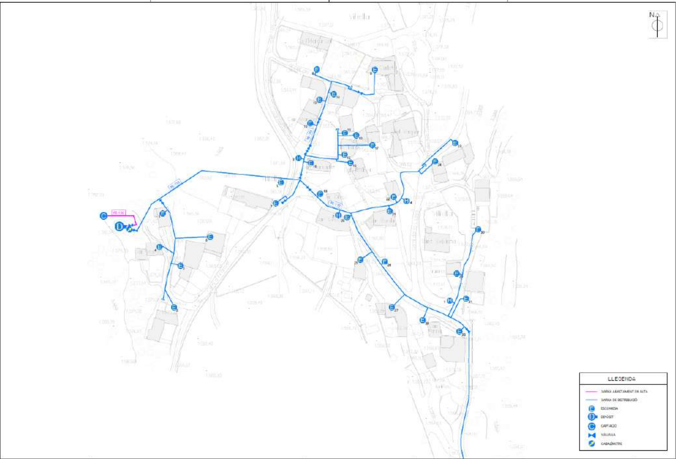
Figura 17. Distribució dels materials per a Viliella
