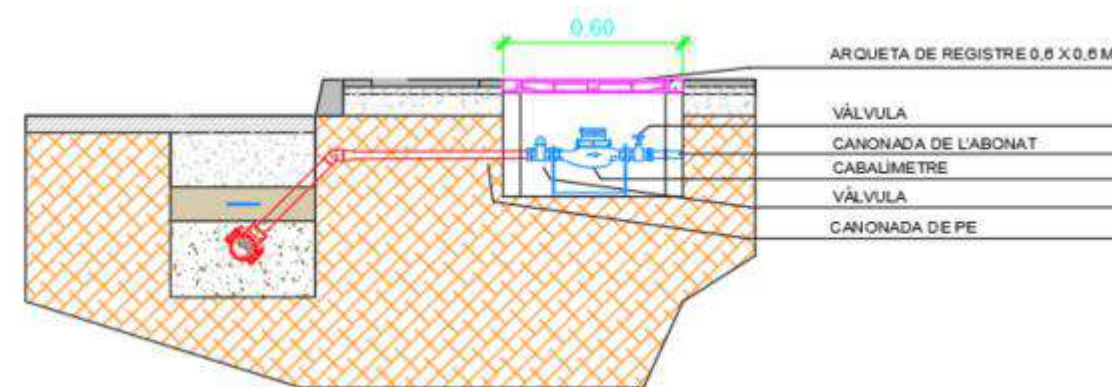
Figura 19. Detall constructiu tipus de l'arqueta de registre
