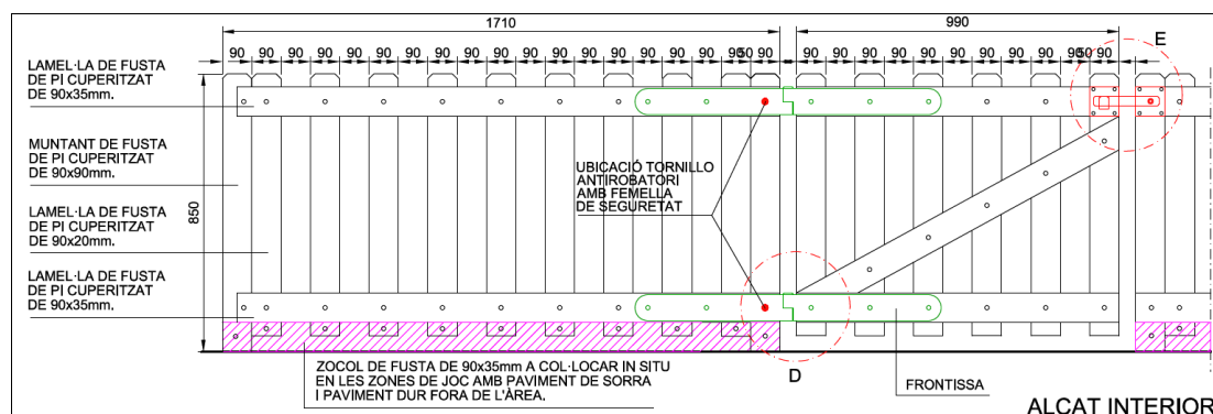
Perfil longitudinal tanca tipus Anglès
