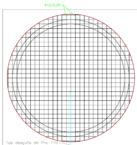
Imatge 33: Esquema de l'armat de la sabata.
