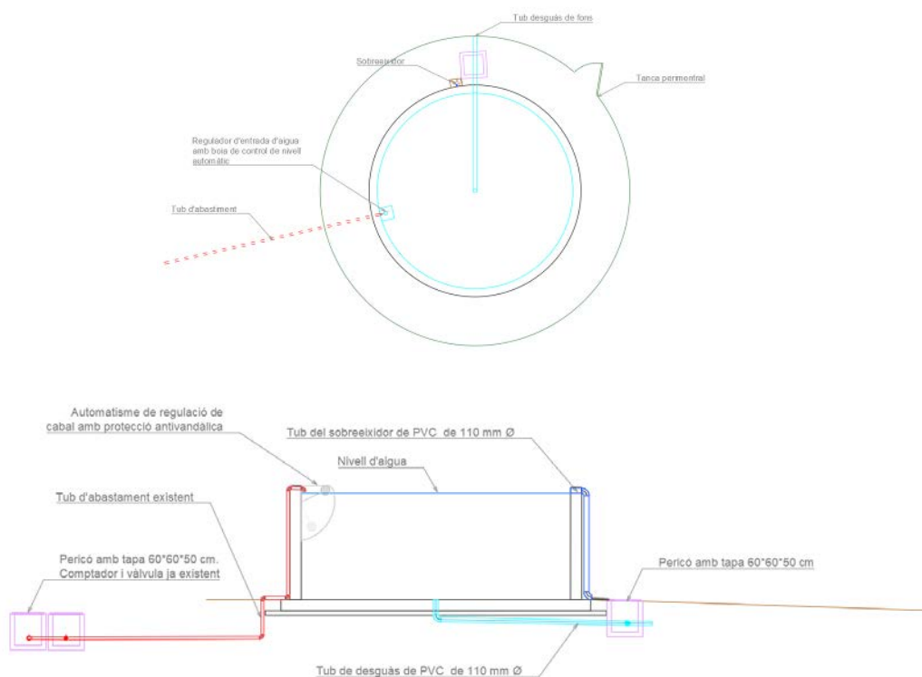
Imatge 44: Elements hidràulics dels punts d'aigua.
