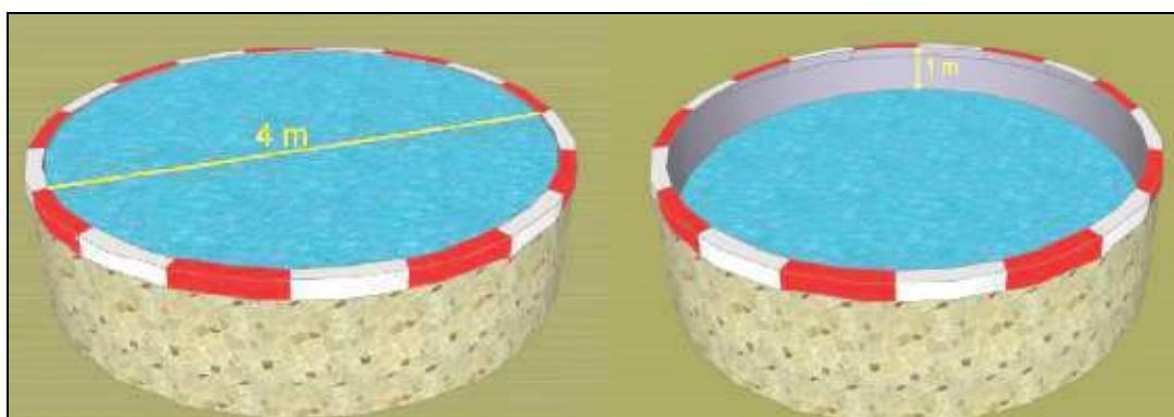
Imatge 31: Dimensió mínima de la làmina d'aigua i requeriment mínim de fondària de la làmina d'aigua per a la càrrega de mitjans aeris.
