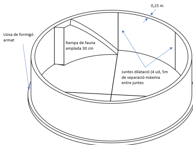
Imatge 32: Esquema del nou punt d'aigua proposat
