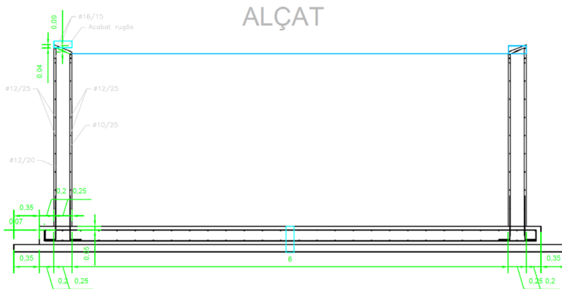
Imatge 35: Esquema de l'armat de les parets del punt d'aigua.
