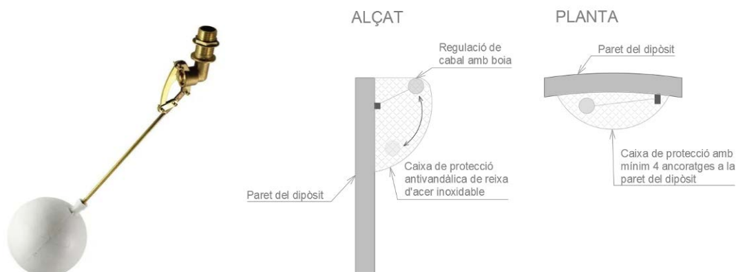
Imatge 43: Automatismes de regulació de cabal i esquema orientatiu de la caixa de protecció.
