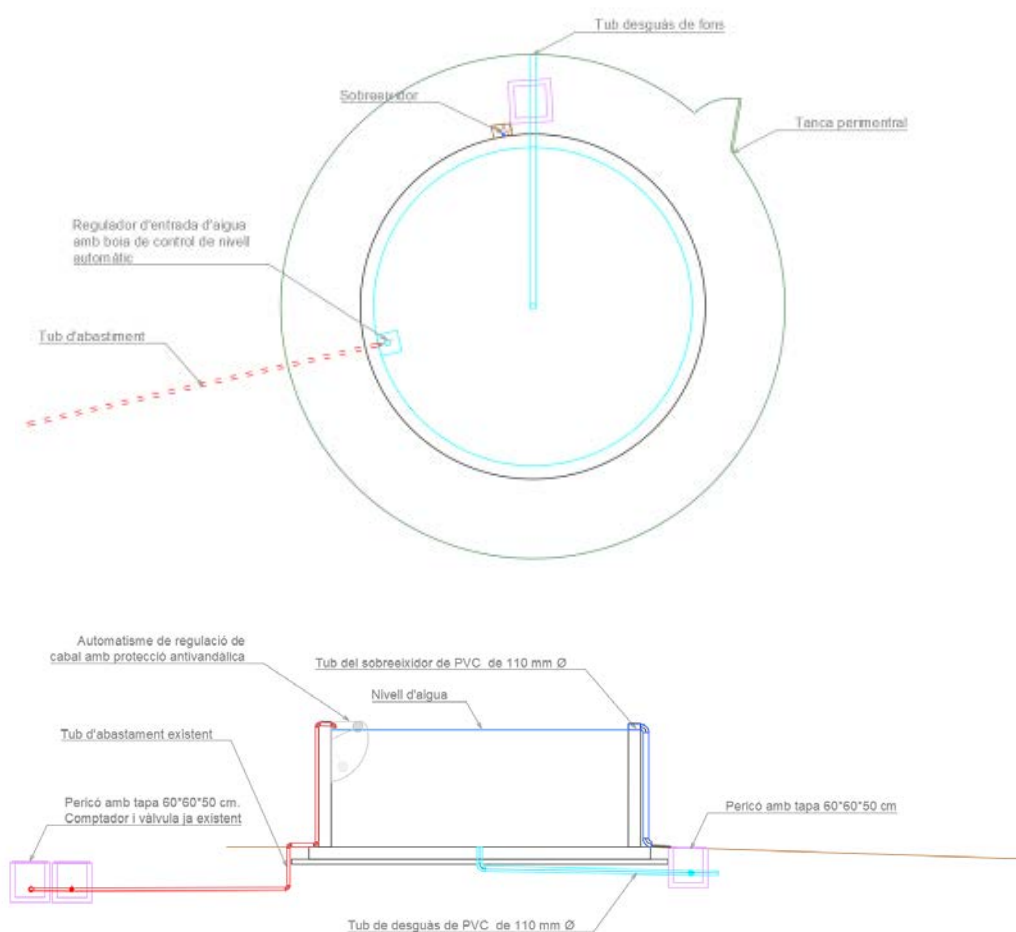
Elements hidràulics dels punts d'aigua
