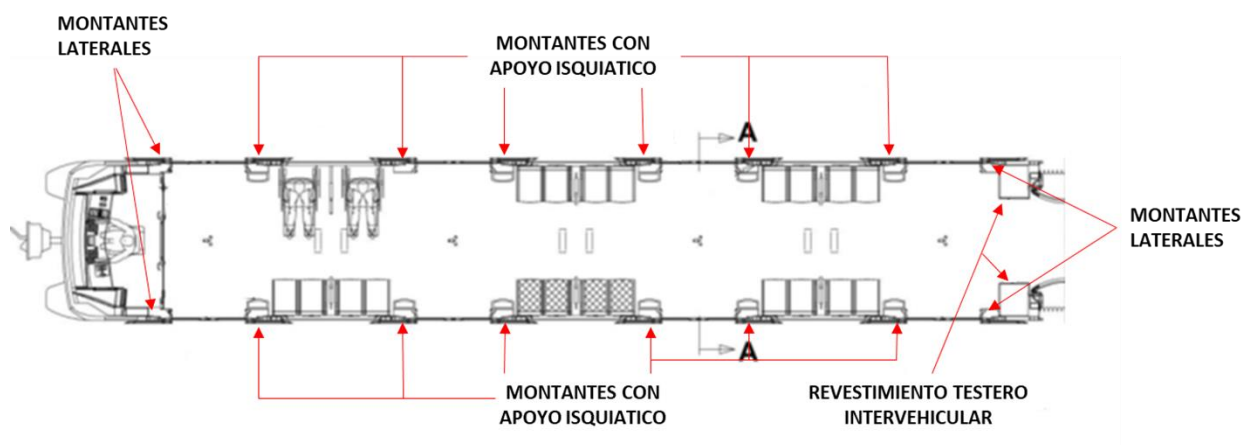
Figura 3.1 Exemple d'ubicació en MA1 dels elements S/5000 i S/6000
