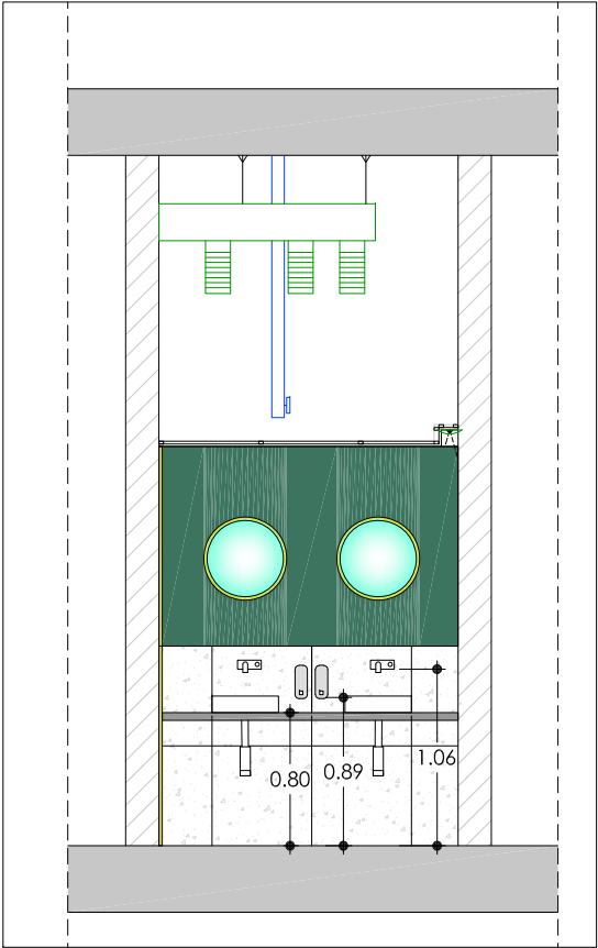
Secció cc' e: 1/50
