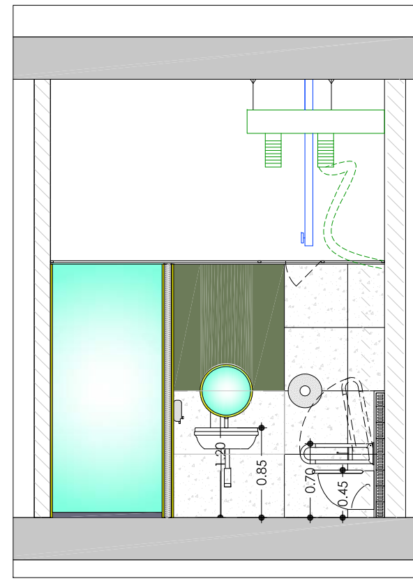
Secció cc' e: 1/50
