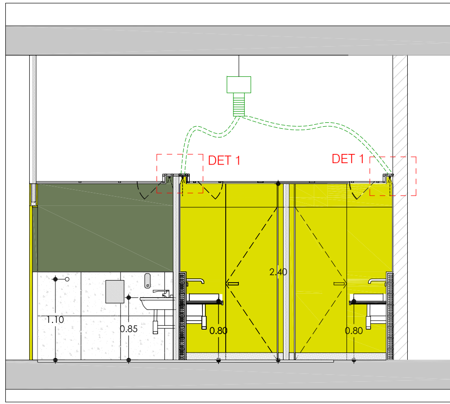
Secció aa' e: 1/50
