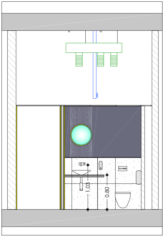
Secció cc' e: 1/50
