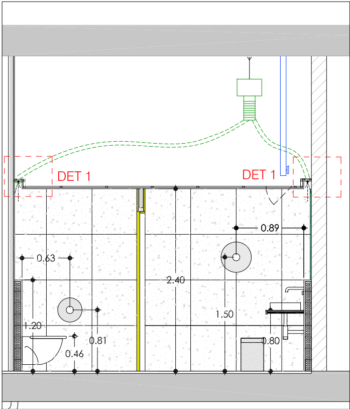
Secció bb' e: 1/50
