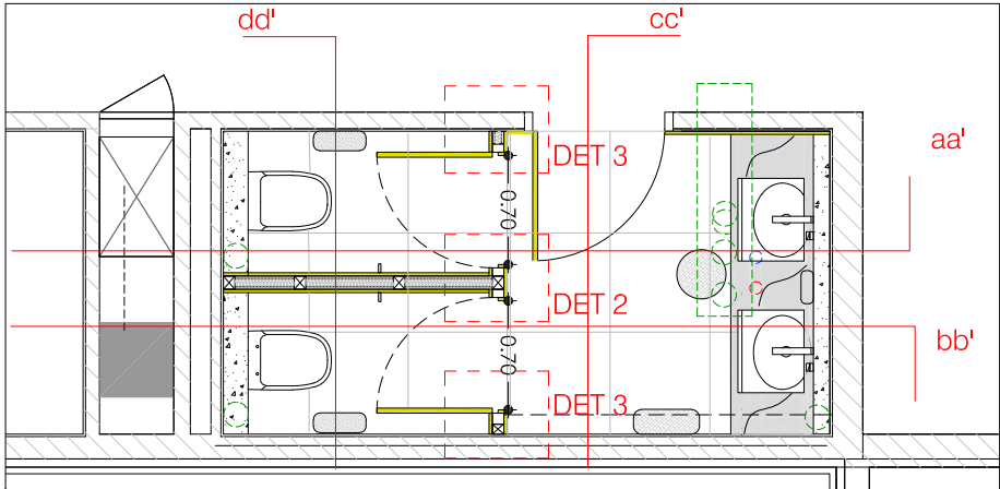
Planta Servei Higènic CL01BC71 e: 1/50
