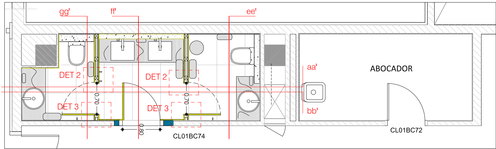
Planta Servei Higienic CL01BC74 e: 1/50
