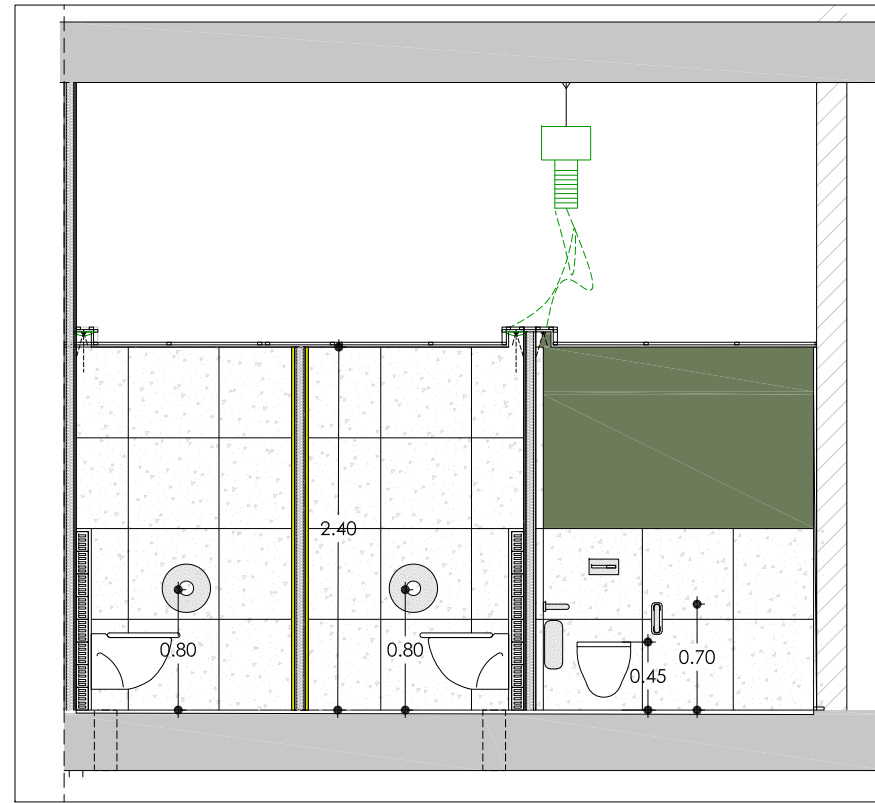
Secció bb' e: 1/50
