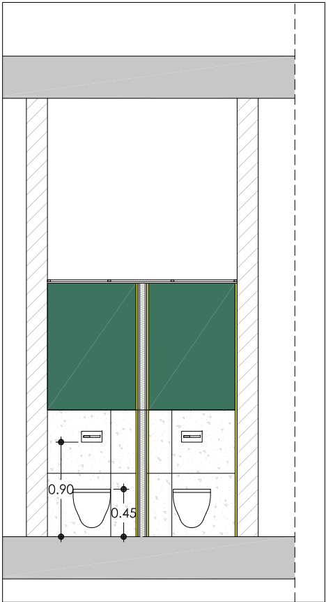
Secció dd' e: 1/50
