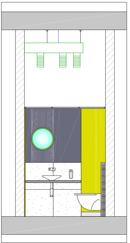
Secció gg' e: 1/50
