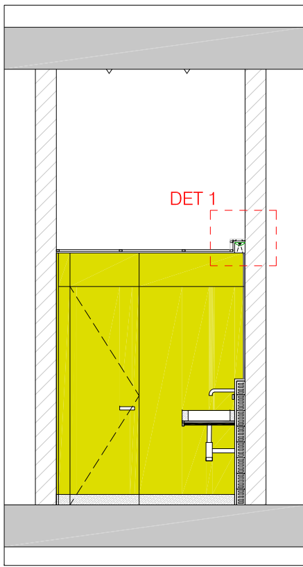
Secció ff' e: 1/50
