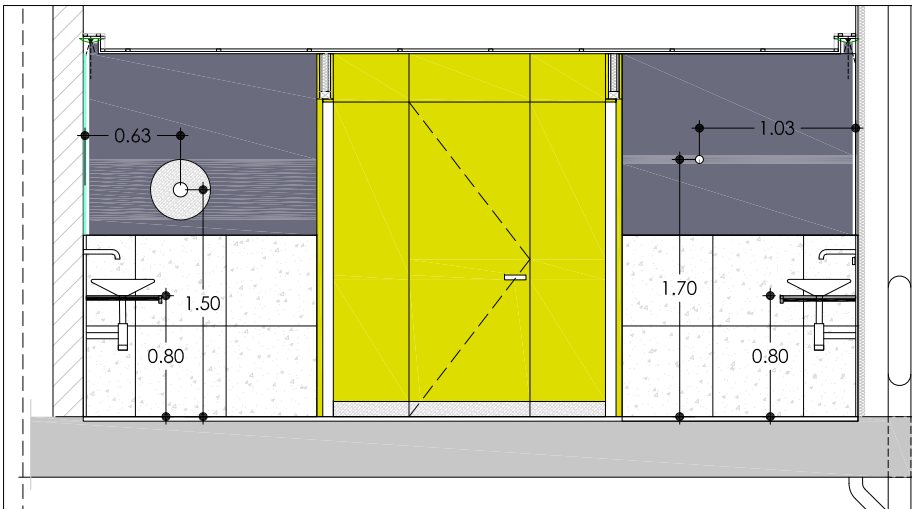
Secció bb' e: 1/50
