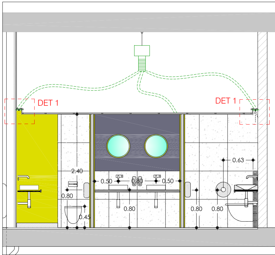
Secció aa' e: 1/50
