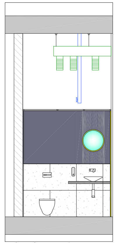
Secció dd' e: 1/50
