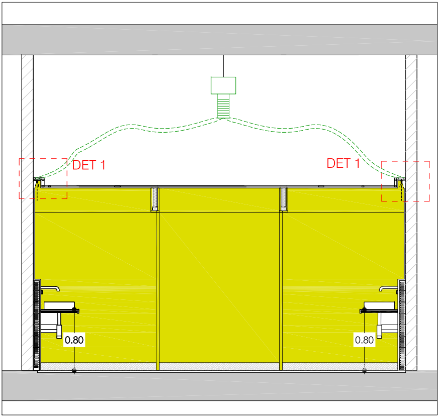
Secció aa' e: 1/50
