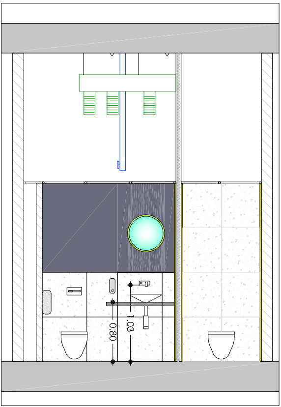
Secció dd' e: 1/50
