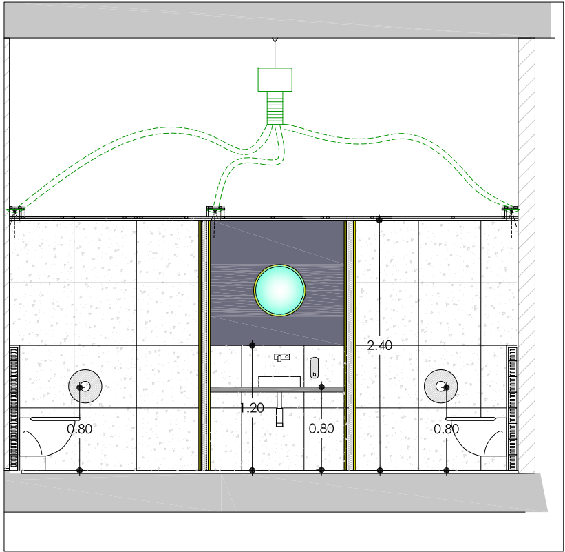
Secció bb' e: 1/50
