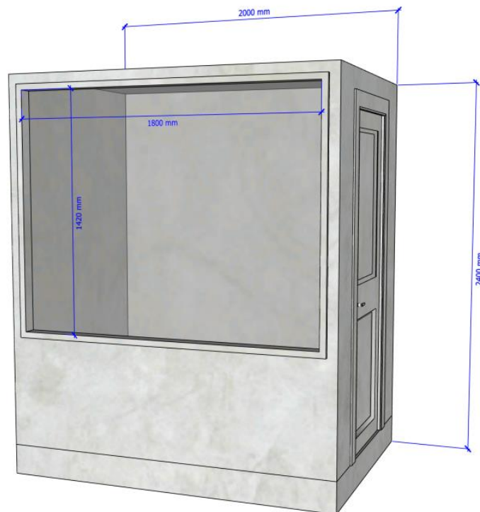
Detall cabina
