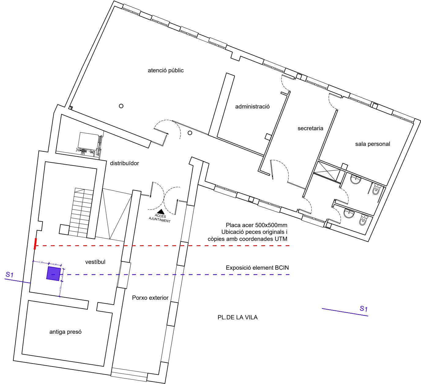
PLANTA PROPOSTA EXPOSICIÓ BCIN - PLANTA BAIXA EDIFICI AJUNTAMENT D'ALMENAR E1:150
