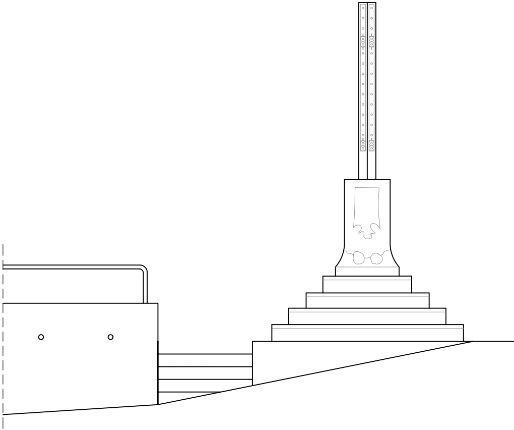
ALÇAT A1 - ESTAT ACTUAL E1:50
