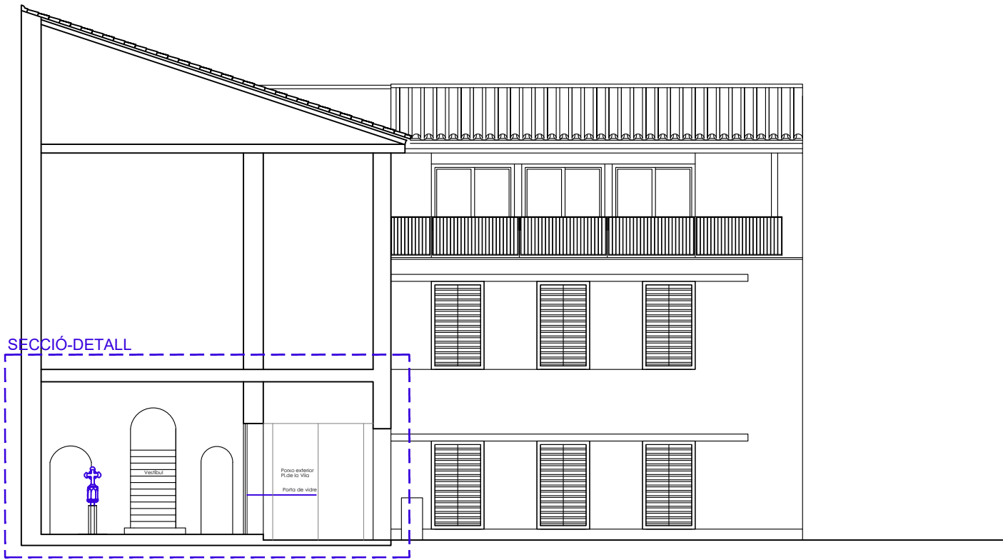
SECCIÓ S1 EDIFICI PROPOSTA EXPOSICIÓ BCIN - AJUNTAMENT D'ALMENAR E1:150
