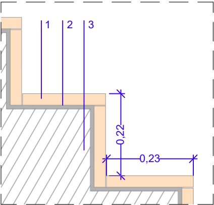
DETALL ESCALA E1:10
