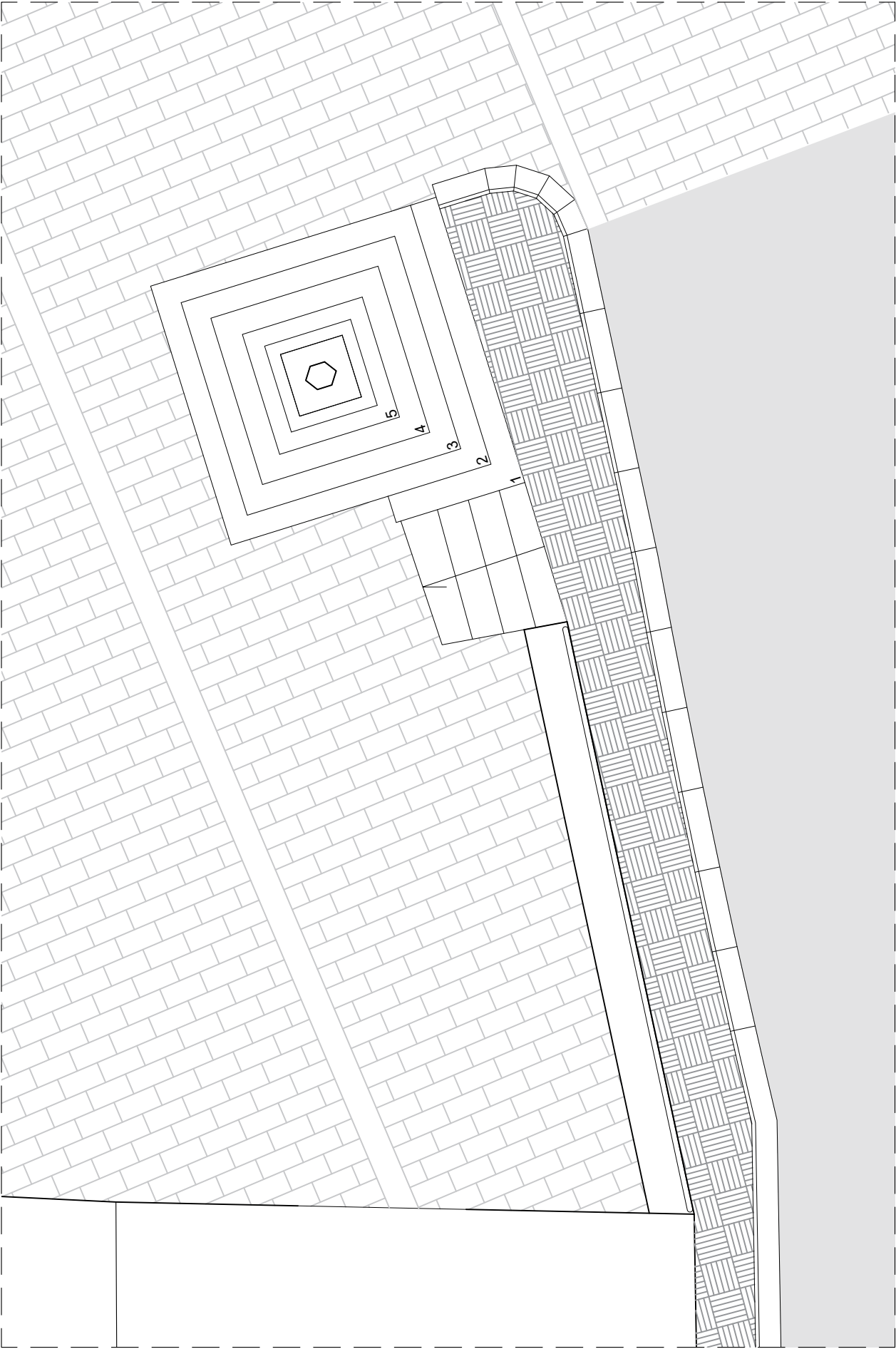
PLANTA ESTAT ACTUAL - PLAÇA SOLDEVILA E1:50
