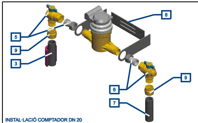
INSTAL·LACIÓ COMPTADOR DN 20
