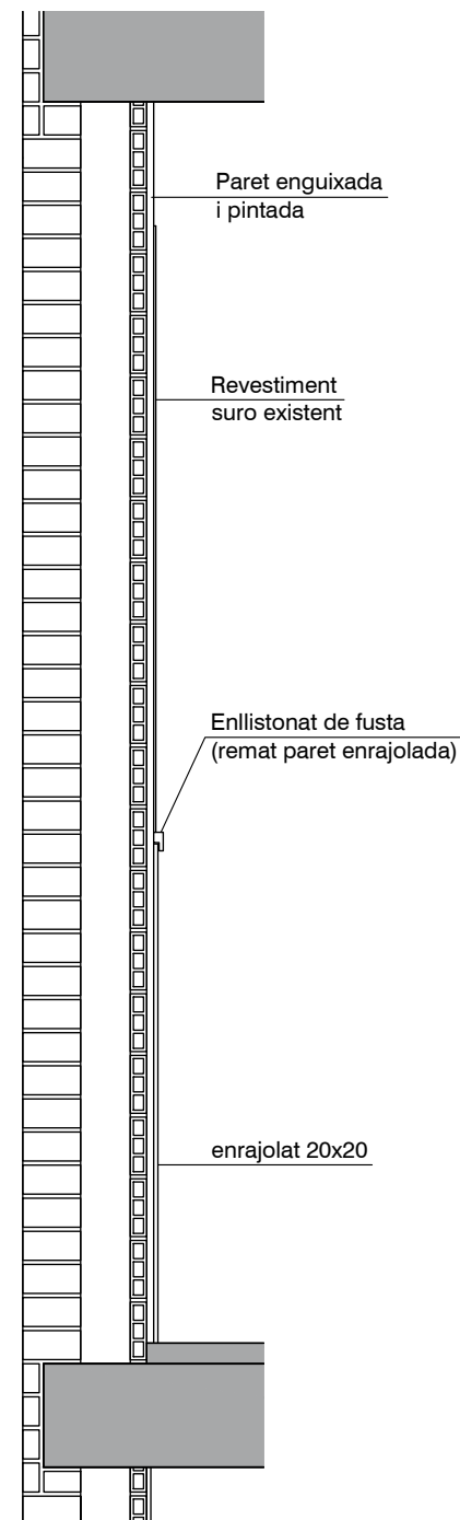
SECCIÓ TIPUS PARET CEGA ESTAT ACTUAL E. 1/20
