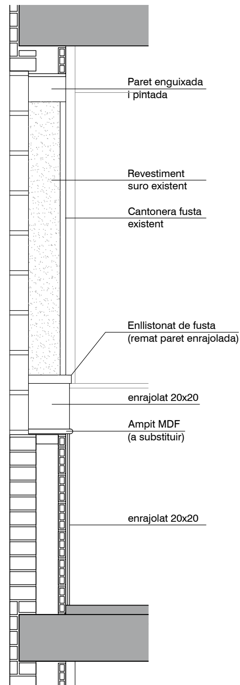
SECCIÓ TIPUS FINESTRA ESTAT ACTUAL E. 1/20
