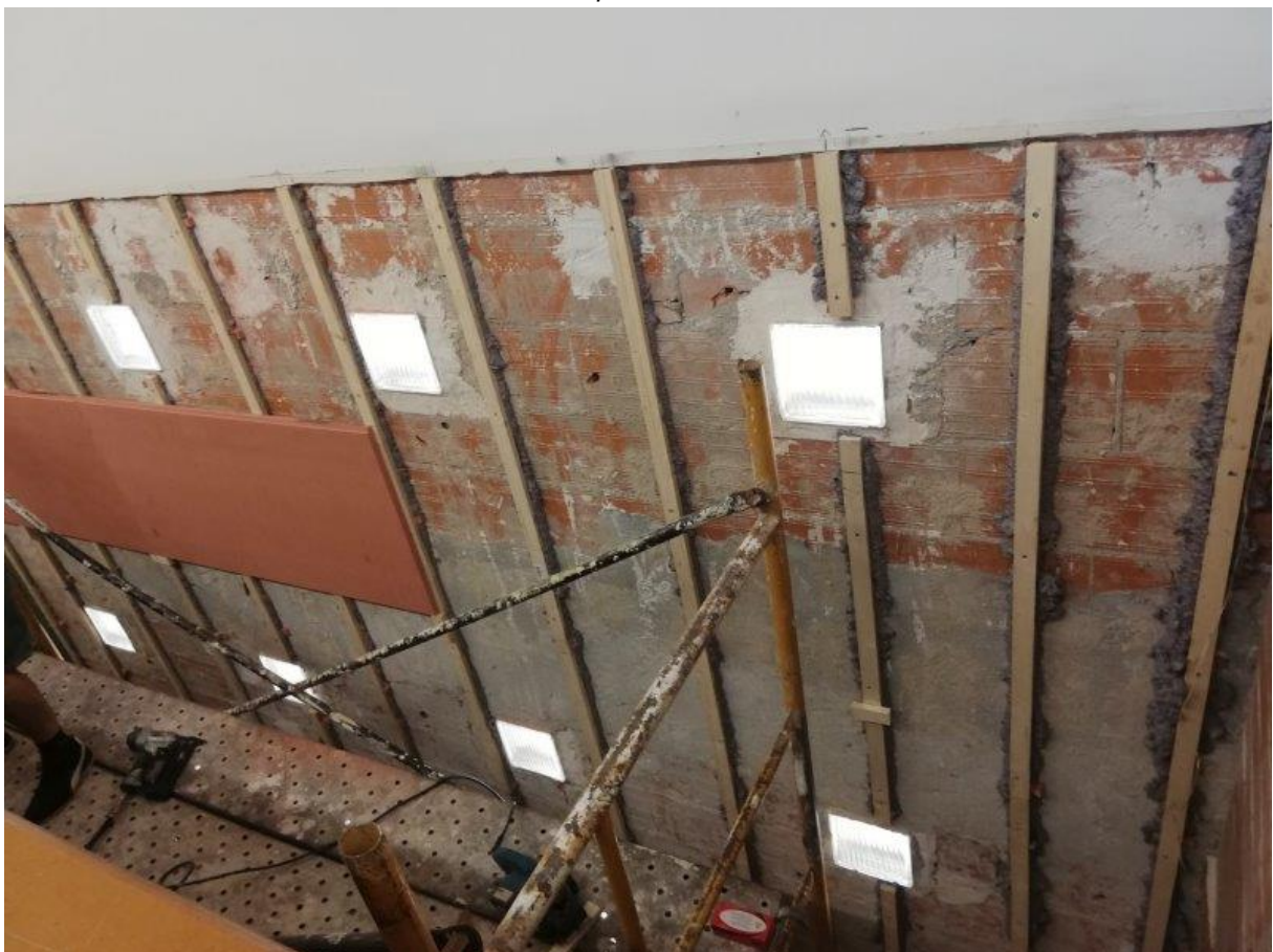
Vista col·locació de llistons de fusta i nous panells de MDF ignífug per arrambadors en zona d'escala.
