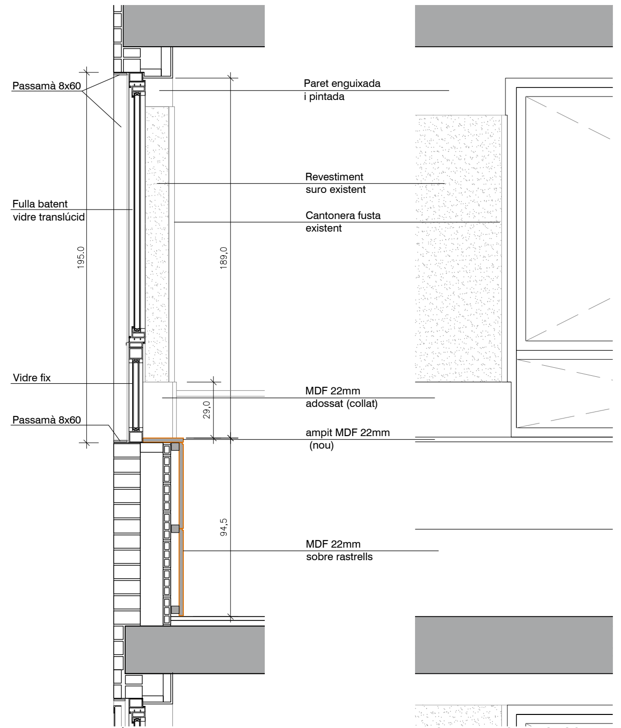
SECCIÓ PROPOSTA PLANTA SUPERIOR E. 1/20
