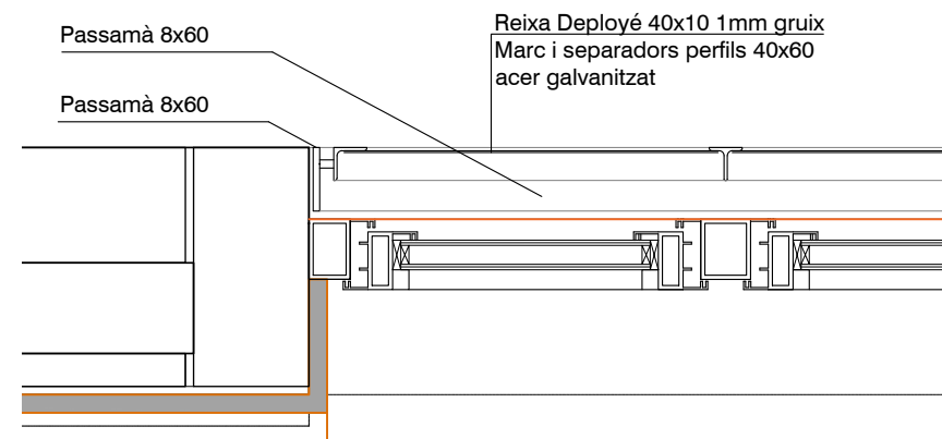
PLANTA PROPOSTA PLANTA BAIXA E. 1/10
