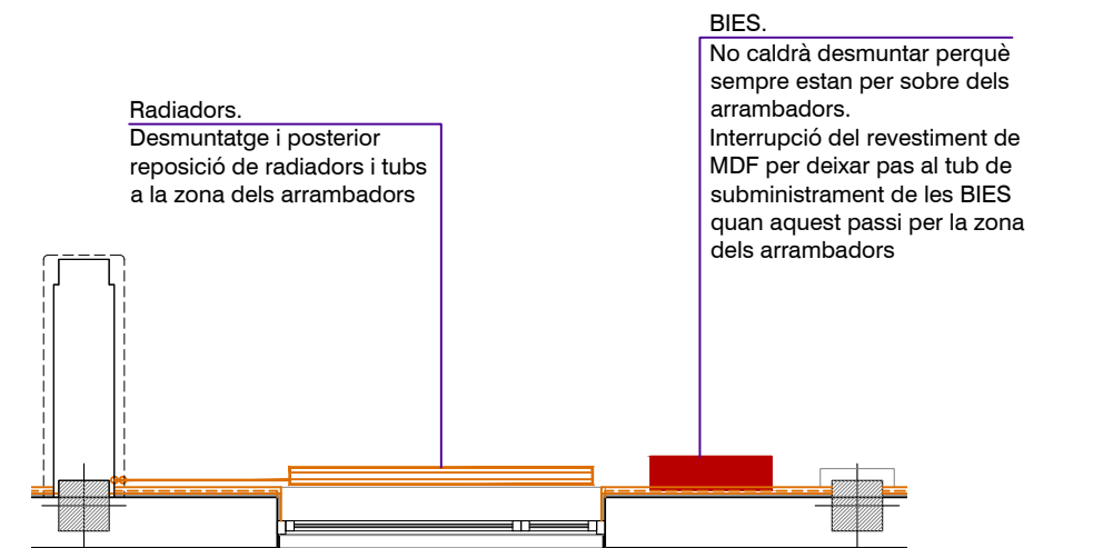
PLANTA MÒDUL-ADEQUACIÓ INSTAL·LACIONS e. 1:50
