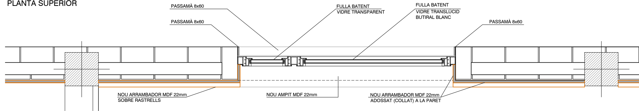
PLANTA MÒDUL PLANTA SUPERIOR e. 1:20
