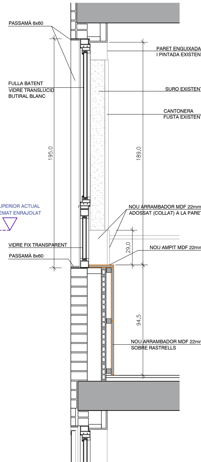
SECCIÓ FINESTRA PLANTA SUPERIOR e. 1:20
