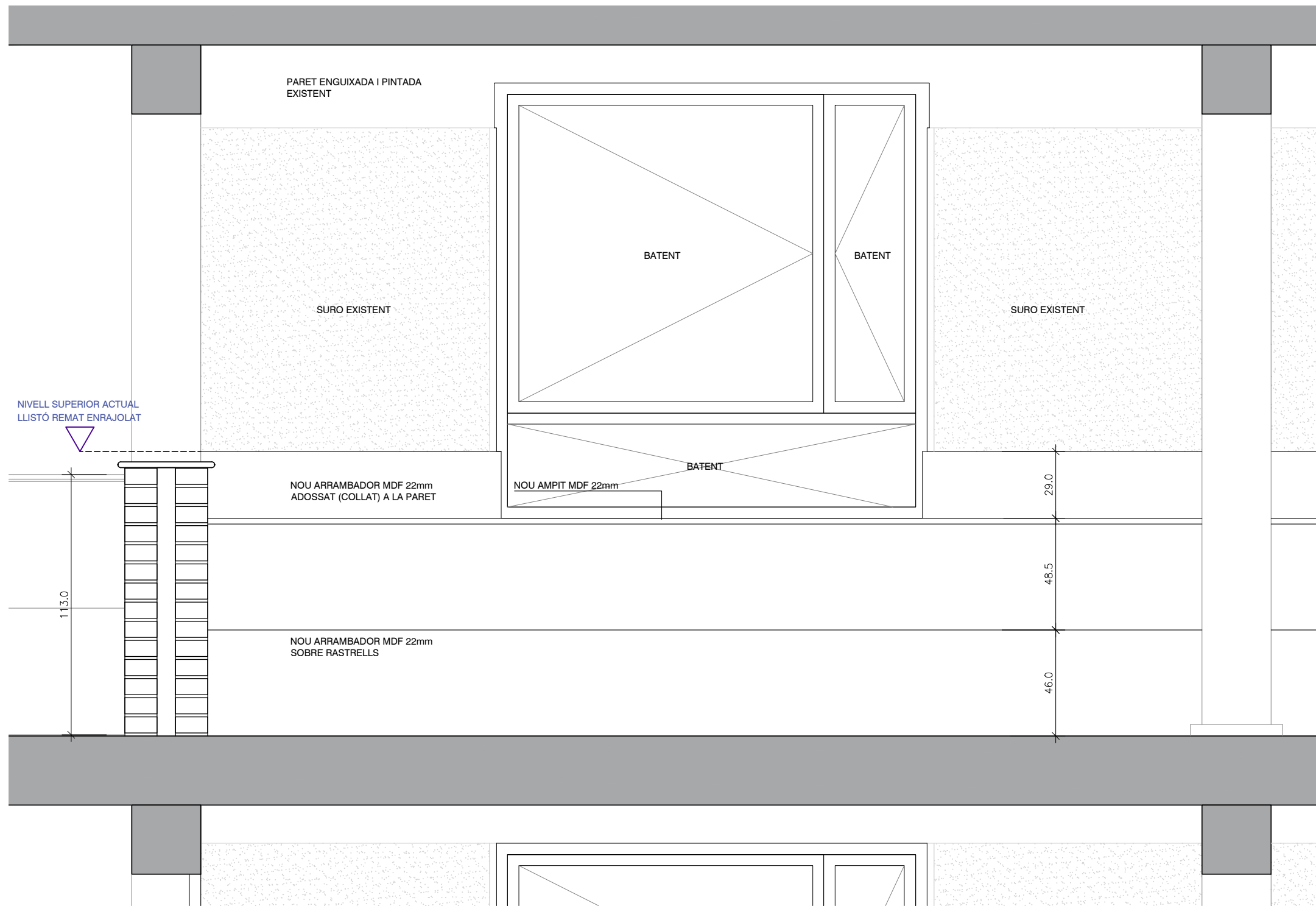
ALÇAT INTERIOR MÒDUL PLANTA SUPERIOR e. 1:20
