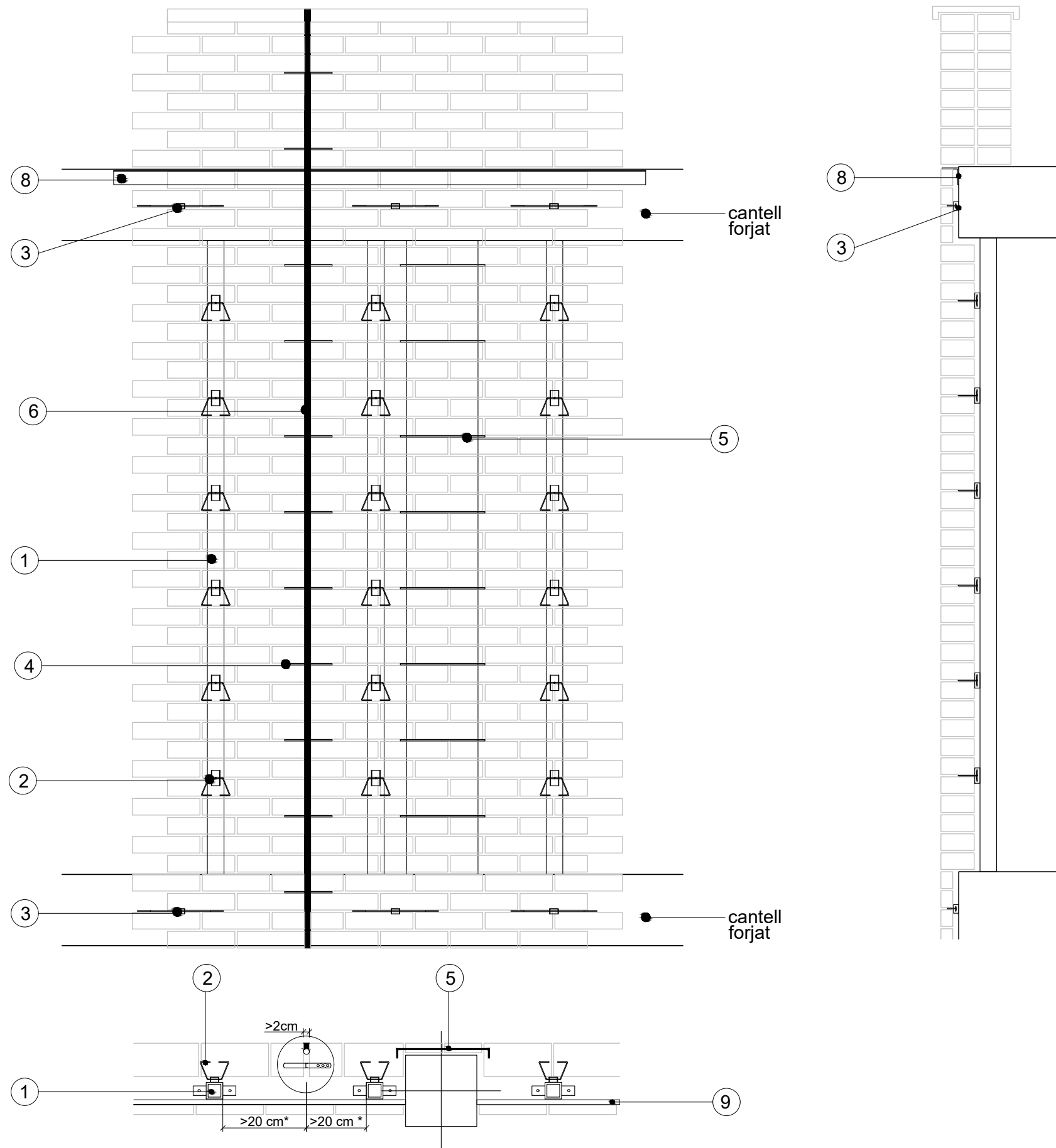
Detall formació noves juntes
