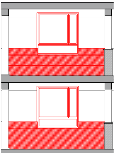
MÒDUL TIPUS: ALÇAT INTERIOR OBRA NOVA e. 1:100
