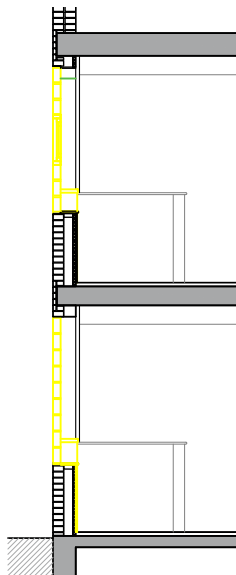
MÒDUL TIPUS: SECCIÓ ENDERROC e. 1:100
