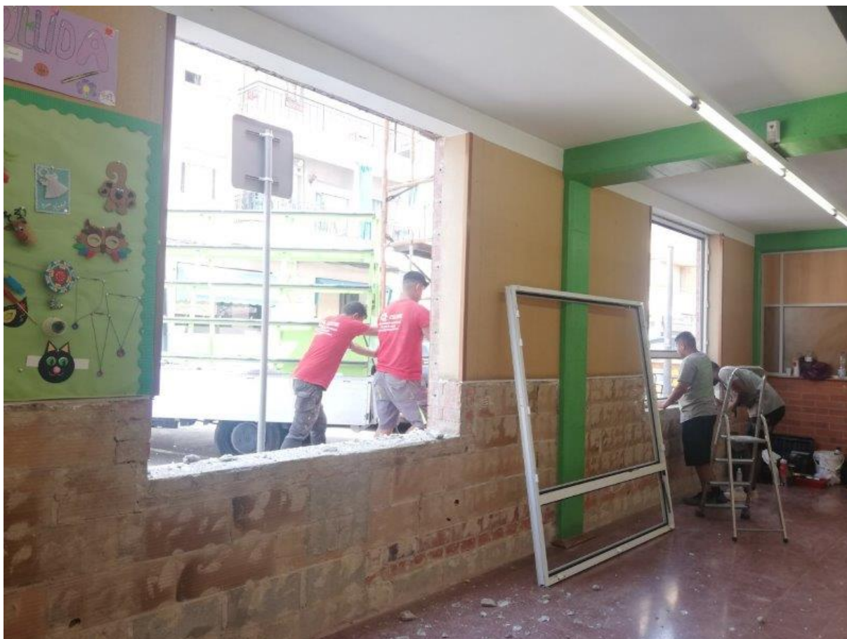
Enderroc dels arrambadors ceràmics interiors. Es manté el revestiment de suro superior
