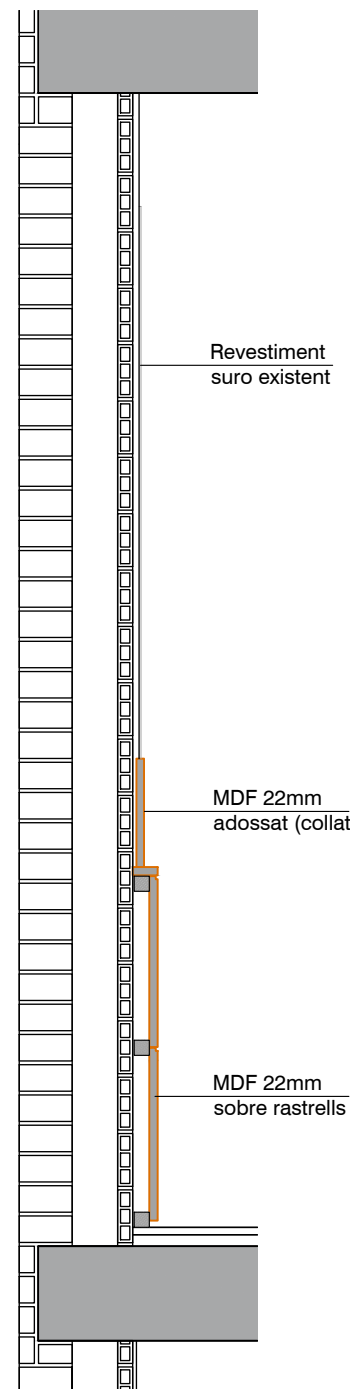
SECCIÓ PROPOSTA PARET CEGA E. 1/20
