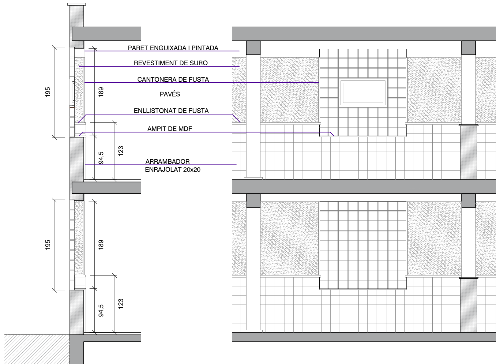
MÒDUL: SECCIÓ ESTAT ACTUAL e. 1:50
