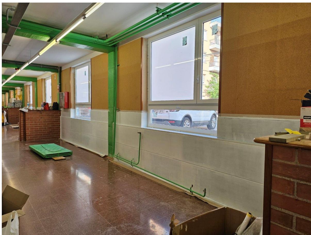
Fusteries noves muntades i arrambadors col·locats amb primera capa d'imprimació a planta baixa
