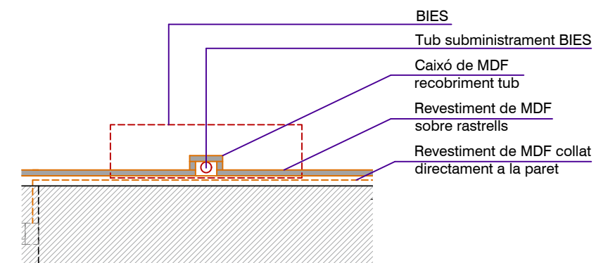
D1- PLANTA DETALL e. 1:20 CAIXÓ PAS TUB BIES
