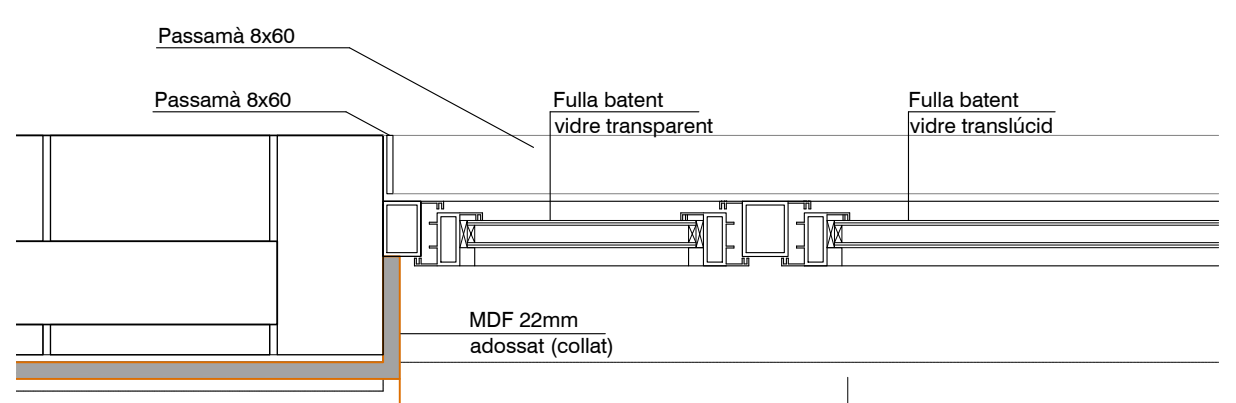
PLANTA PROPOSTA PLANTA SUPERIOR E. 1/10
