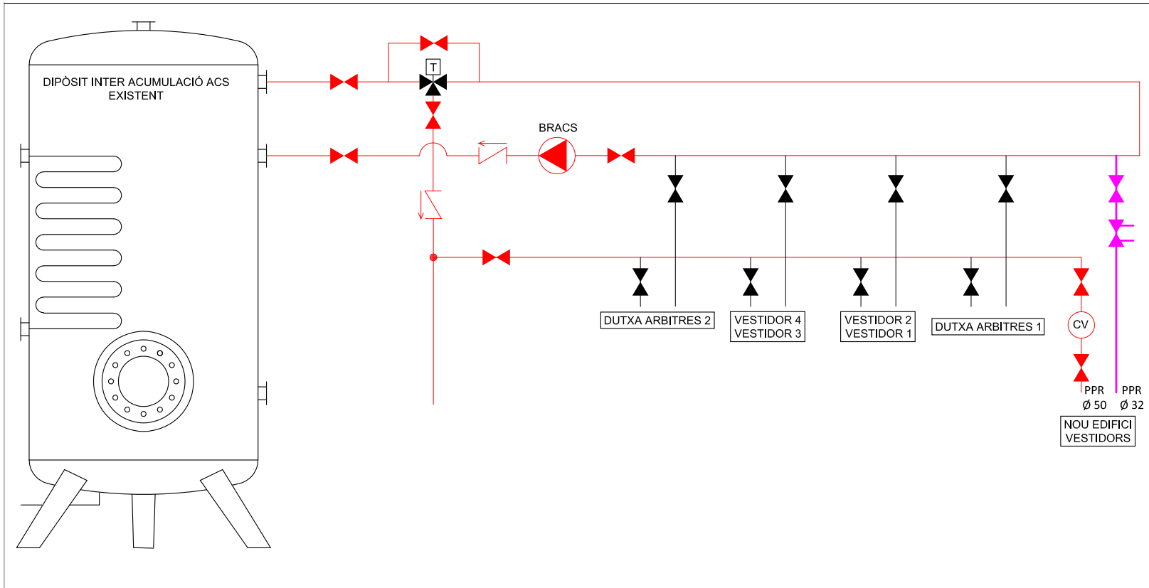
ESQUEMA DE PRINCIPI CONNEXIÓ AIGUA CALENTA SANITÀRIA I RETORN ACS - NOUS VESTIDORS
