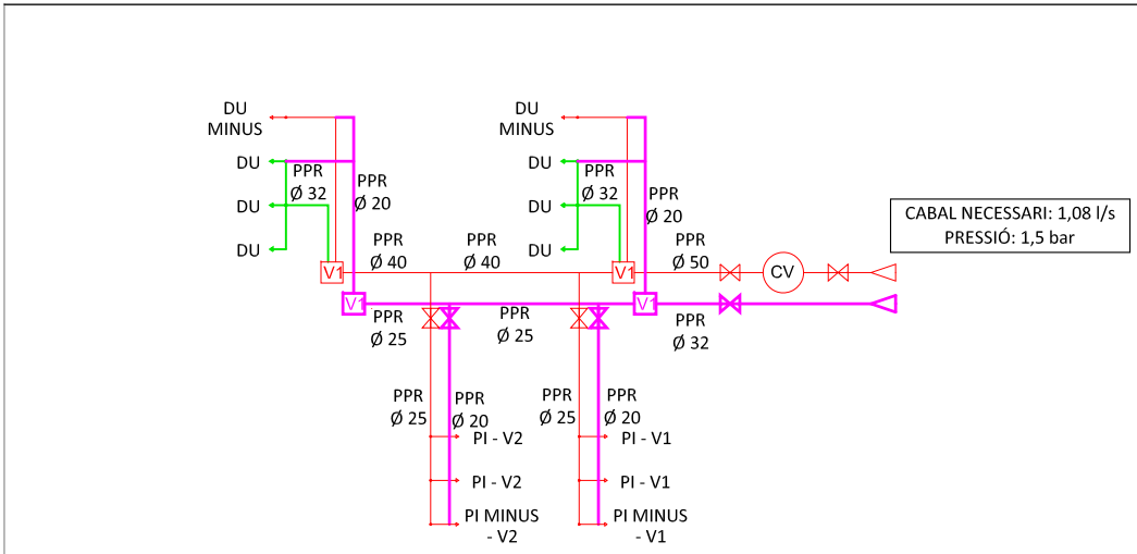
ESQUEMA DE PRINCIPI CONNEXIÓ AIGUA CALENTA SANITÀRIA I RETORN ACS - NOUS VESTIDORS
