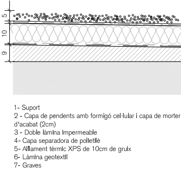
C1- Coberta plana invertida
