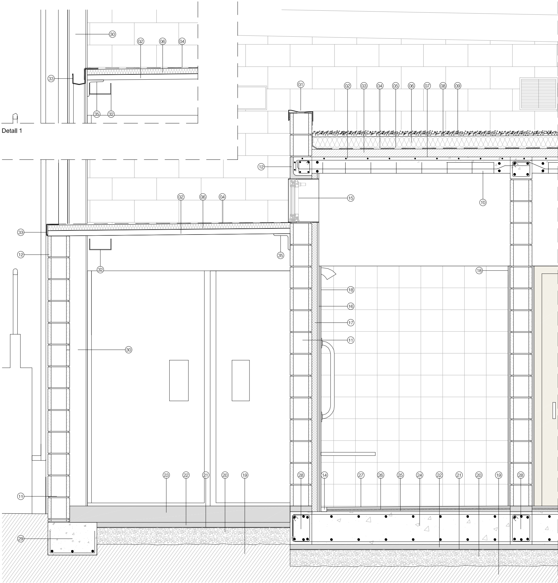
Detall 2
