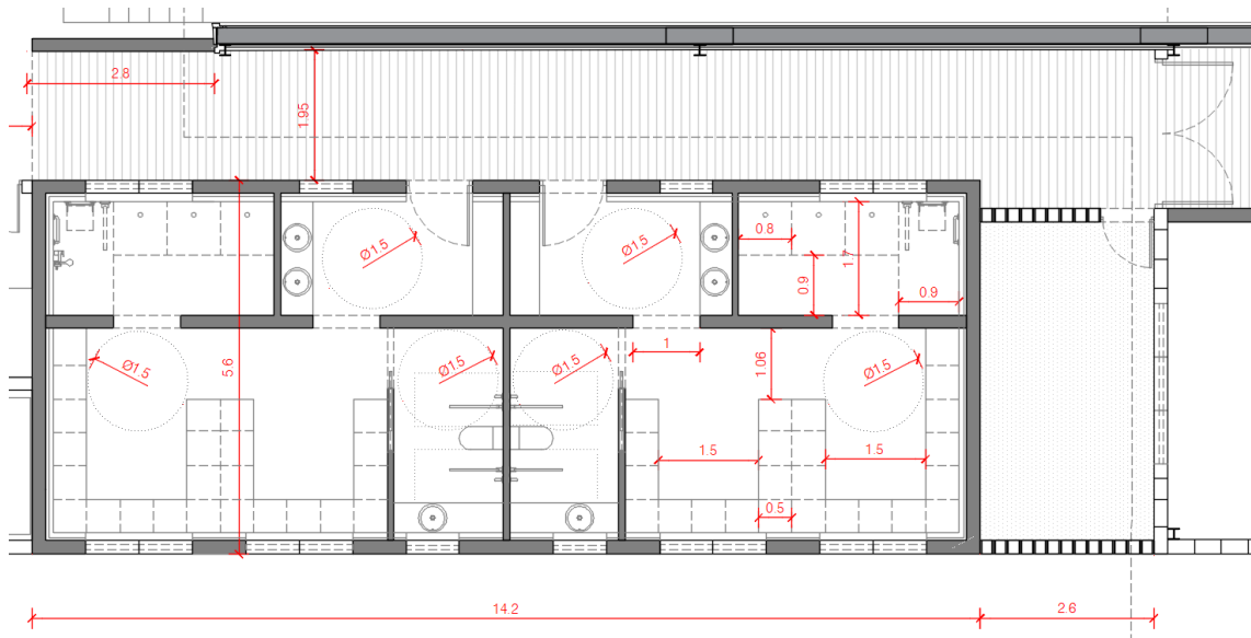
Planta general de l'Estructura del Vestuari de la Llagosta
