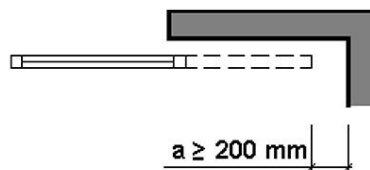
Figura 2.1 Holgura per evitar atrapaments
