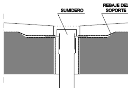
Figura 2.14 Rebañe del soporte alrededor de los sumideros
