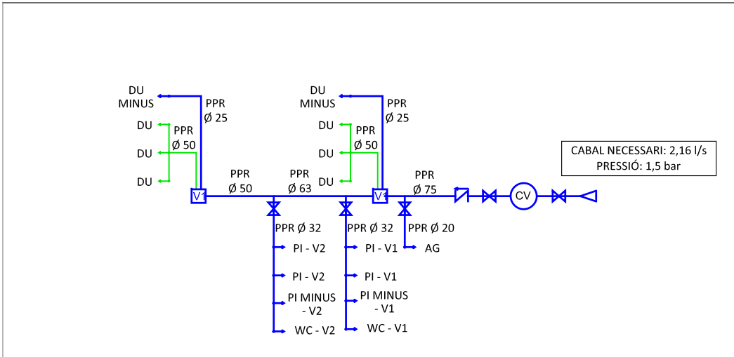
ESQUEMA DE PRINCIPI AIGUA CALENTA SANITÀRIA I RETORN ACS - NOUS VESTIDORS
