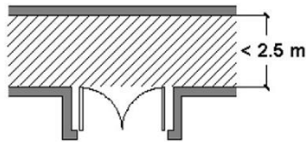
Figura 1.1 Disposició de portes laterals a vies d'evacuació
