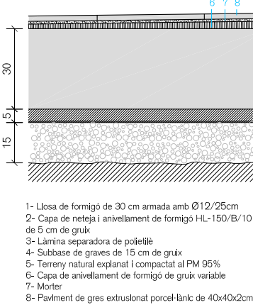
S2. Llosa de fonamentació 30cm
