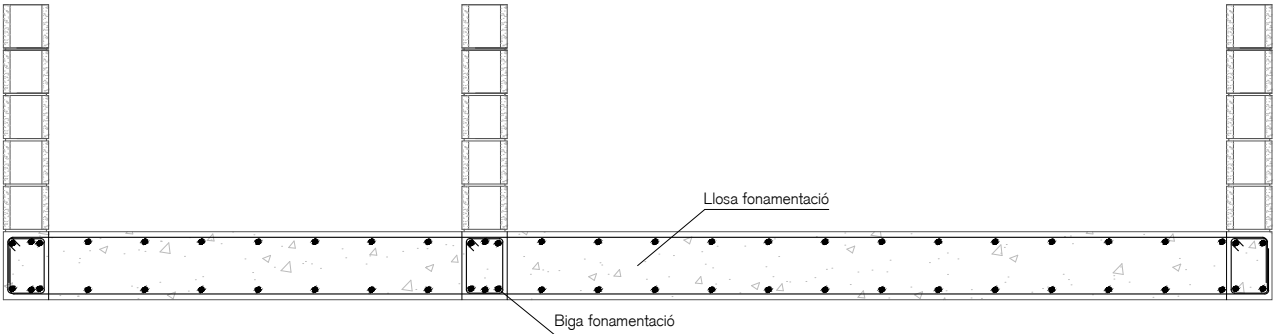
SECCIÓ A-A
