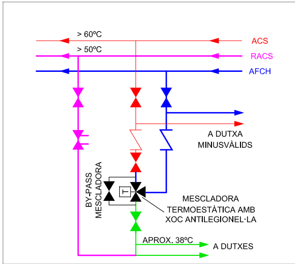
ESQUEMA TIPUS DE VALVULERIA V1
