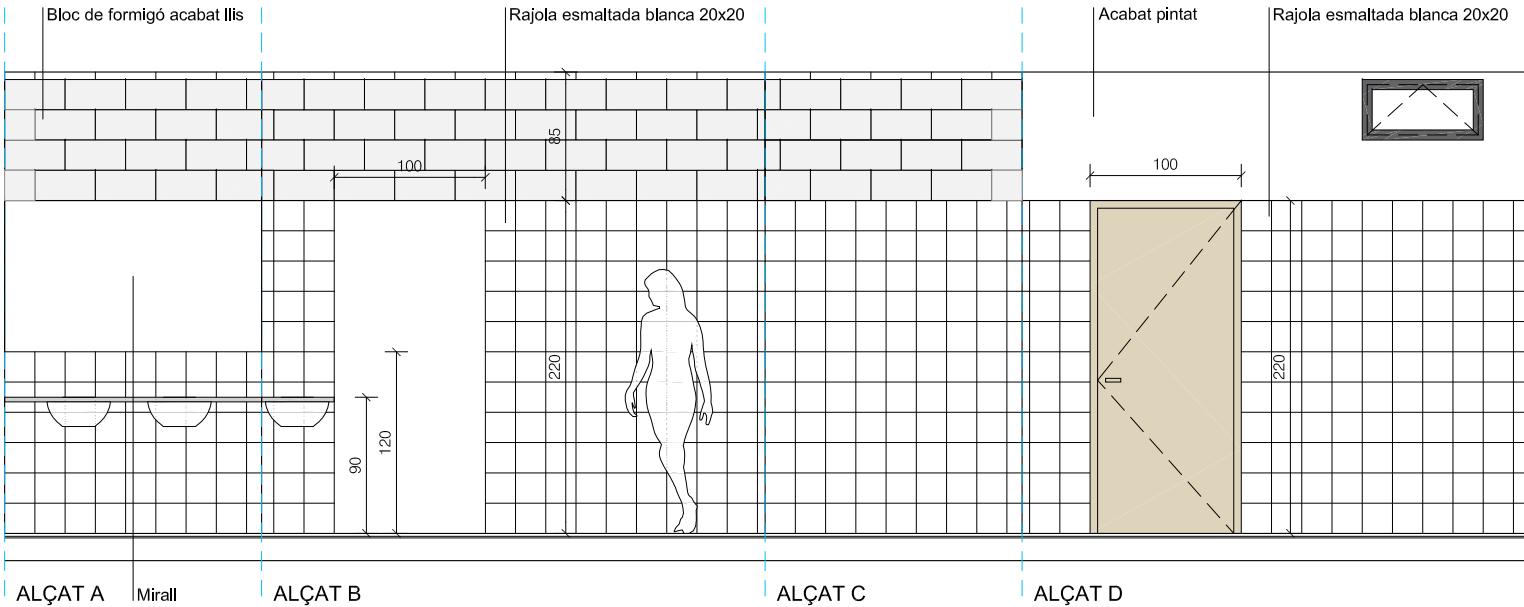
ALÇAT INTERIOR ZONA ACCÉS
