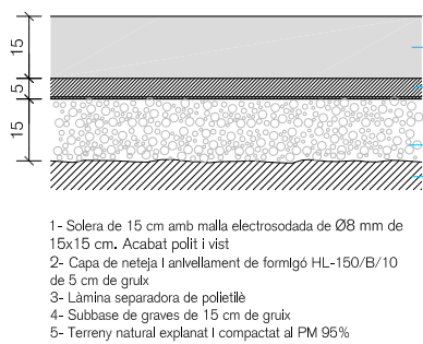
S1. Solera 15cm
