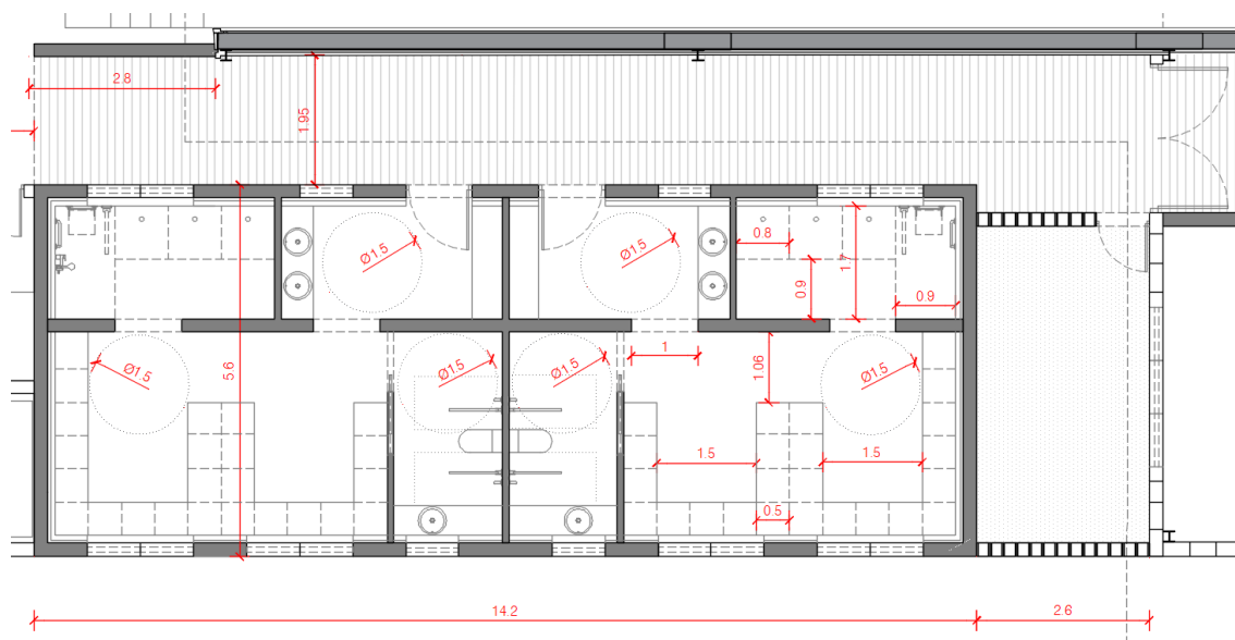
Planta general d' Instal·lacions del Vestuari de la Llagosta
