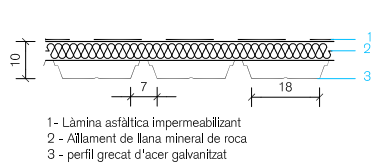
C2- Coberta Deck amb Aïllament i Impermeabilitzant
