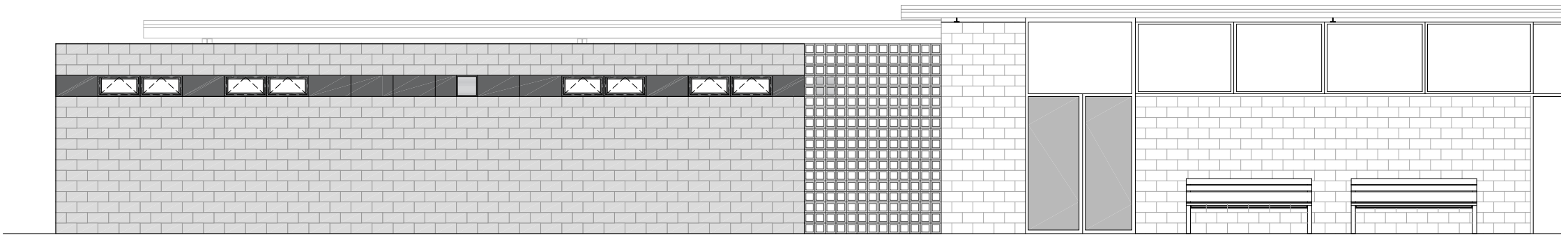
Alçat frontal
