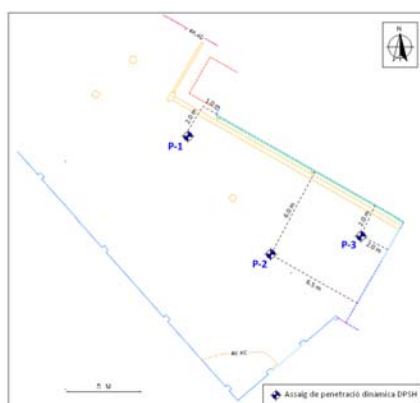
Figura 2. Situació dels assaigs realitzats.
