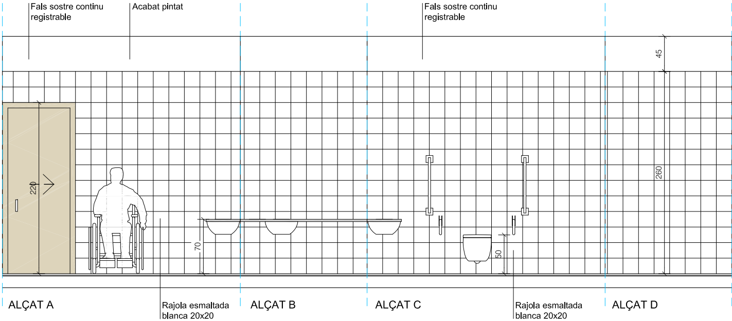
ALÇAT INTERIOR BANY ADAPTAT
