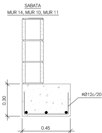
SECCIÓ A-A
