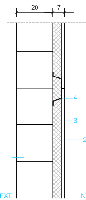
F1 - Mur de blocs de formigó amb aïllament interior
