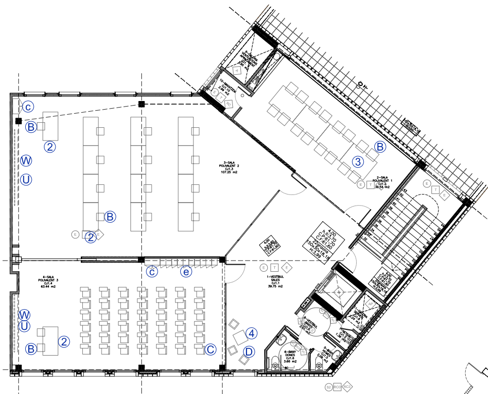
PLANTA P1 C.F: 61,60
