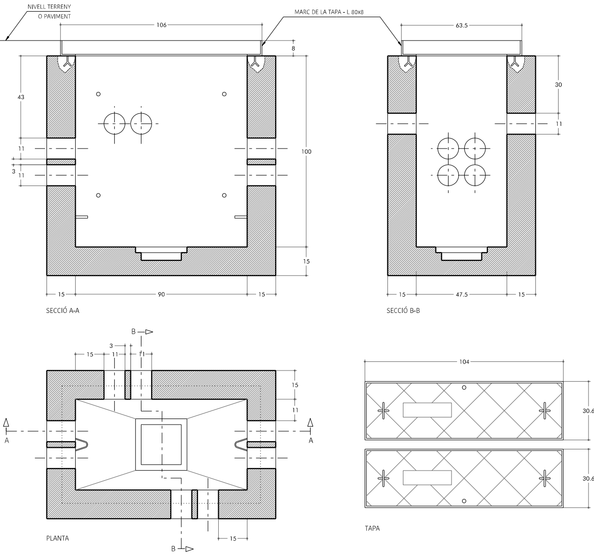
ARQUETA TIPUS "MD" - TELEFONIA
