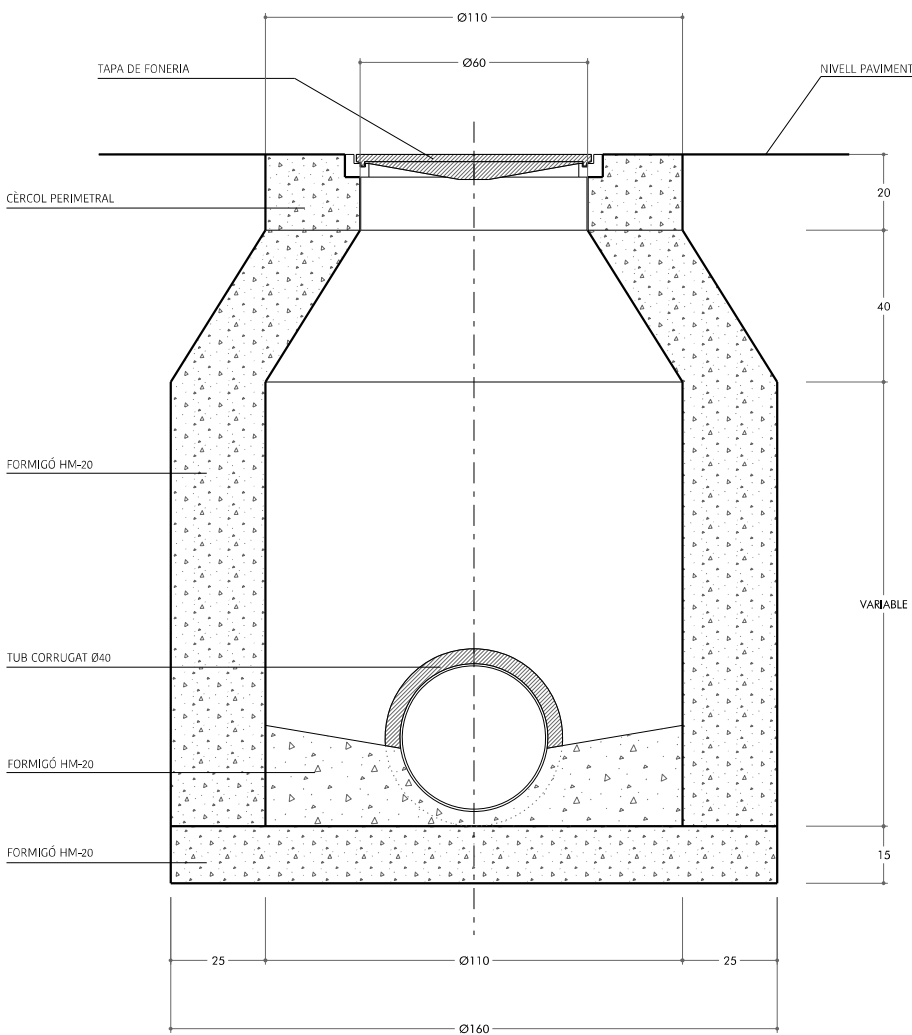
POU DE REGISTRE - SANEJAMENT I PLUJANES
