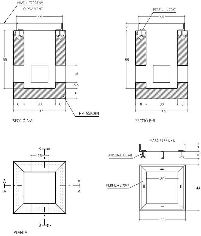
ARQUETA TIPUS "M" - TELEFONIA
