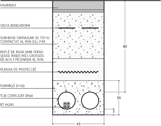
DETALL RASA UN CIRCUIT CREUAMENT CARRER - BAIXA TENSIÓ
