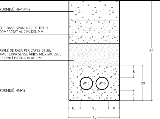
SECCIÓ CANALITZACIÓ - 2 CONDUCTES DE PVC Ø110 - TELEFONIA
