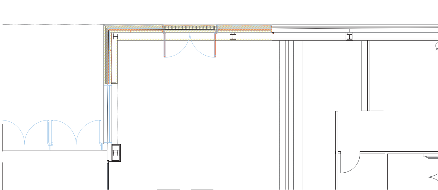
PLANTA BAIXA
