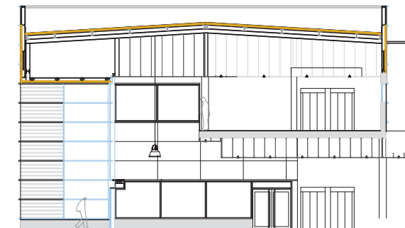
FAÇANA OEST
