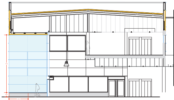
FAÇANA OEST
