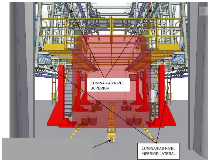
Figura 16 (ejemplo luminarias en cochera Triangle)
