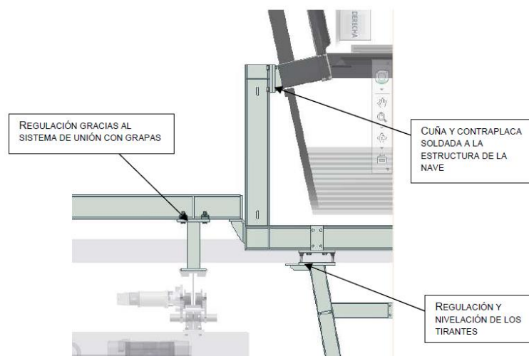
Figura 2 (ejemplo fijación estructura cochera Triangle)
