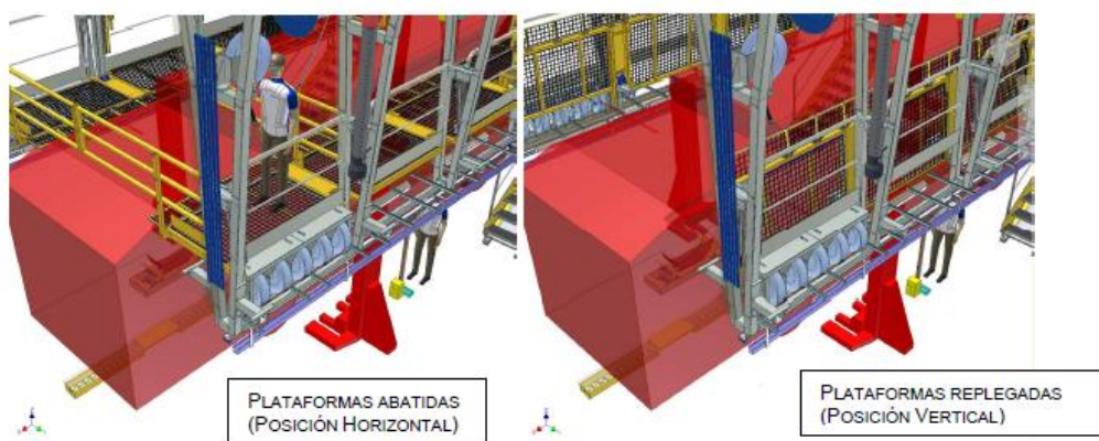
Figura 3 (ejemplo pasarelas abatidas y recogidas cochera Triangle)
