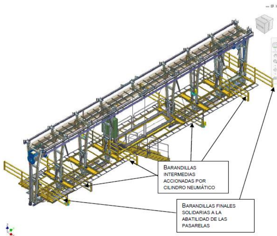
Figura 7 (ejemplo barandillas cochera Triangle)
