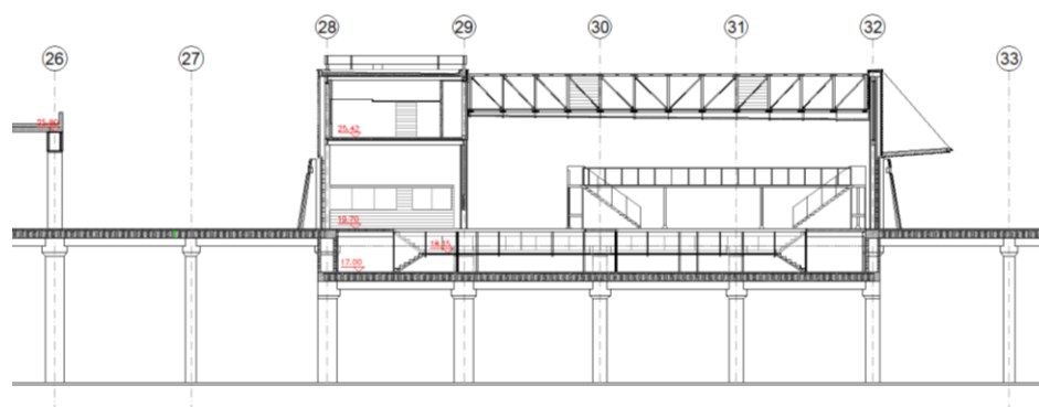
Sección transversal
