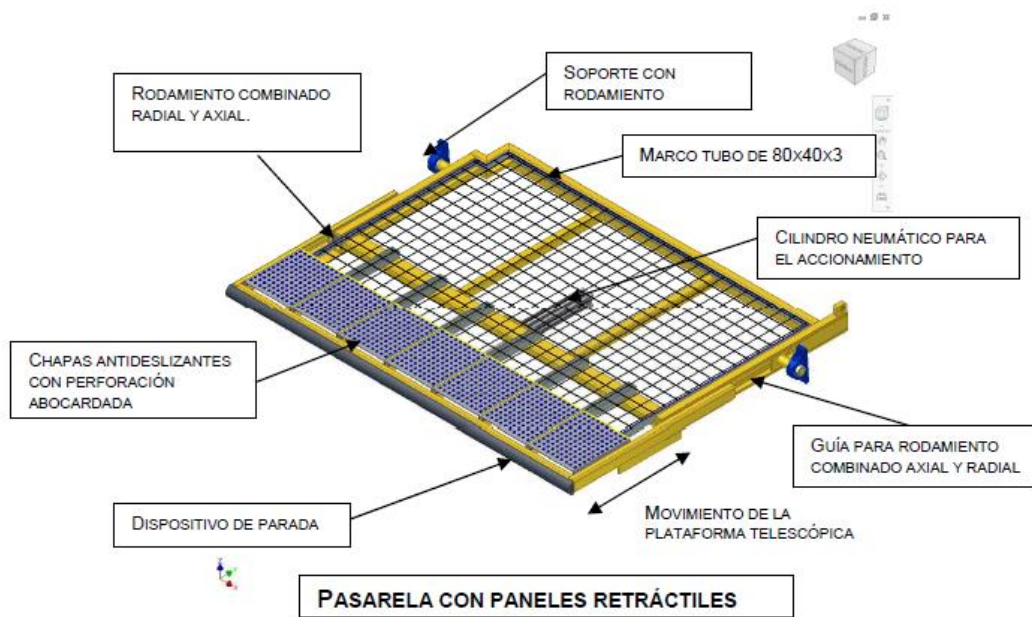
Figura 8 (ejemplo pasarela con panel retráctil cochera Triangle)
