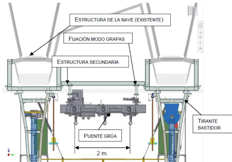
Figura 15 (ejemplo puente grúa en cochera Triangle)
