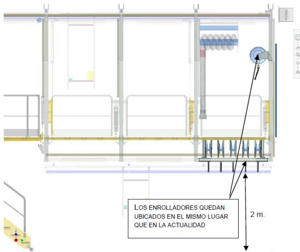
Figura 13 (ejemplo enrollador en cochera Triangle)
