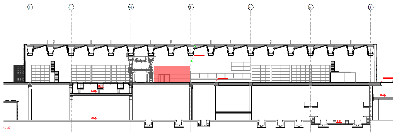
Sección longitudinal
