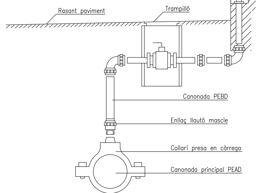
FORMACIÓ D'ESCOMESA
