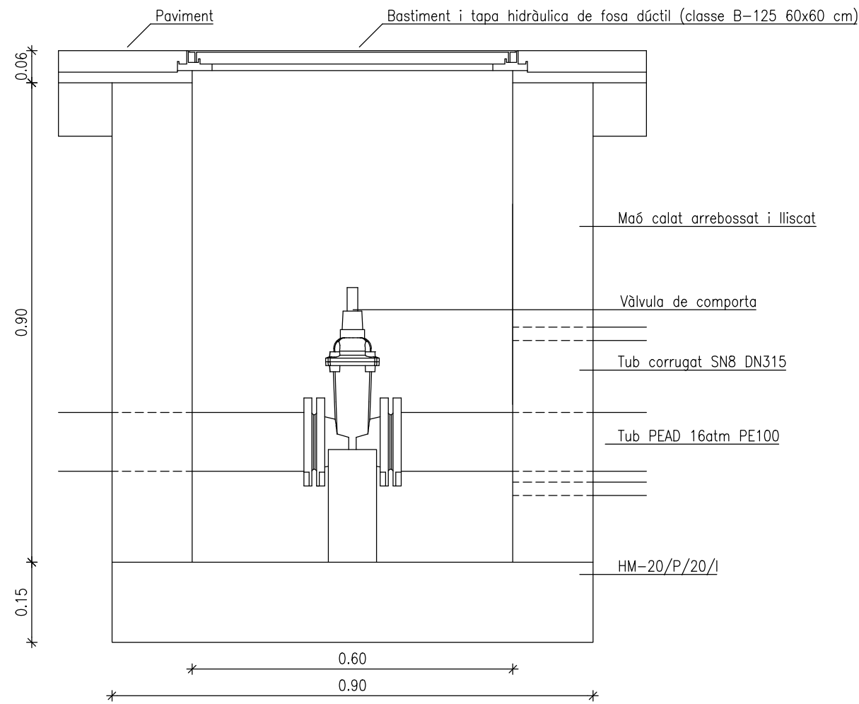
SECCIÓ
