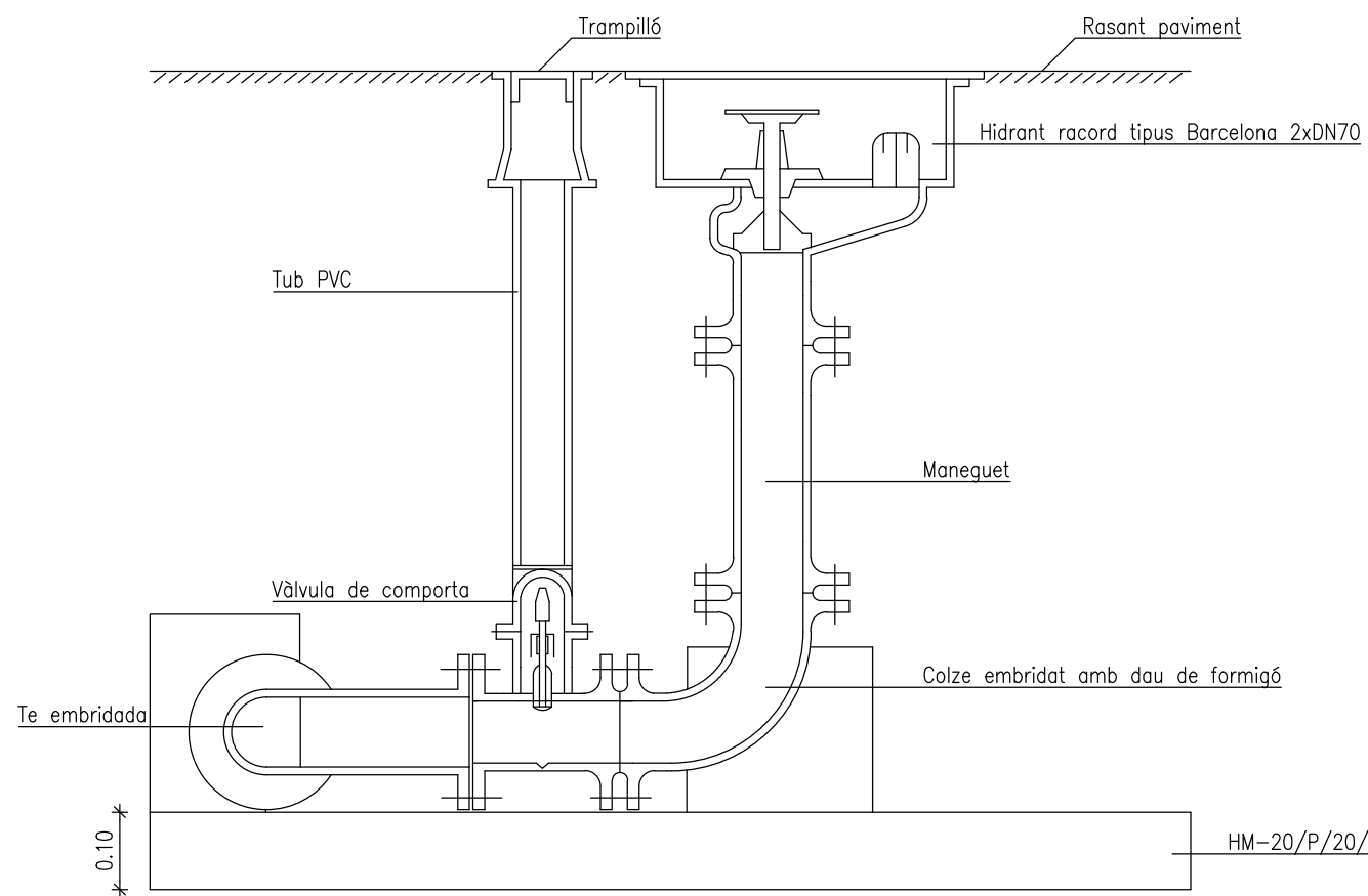
HIDRANT SOTERRAT AMB VÀLVULA
