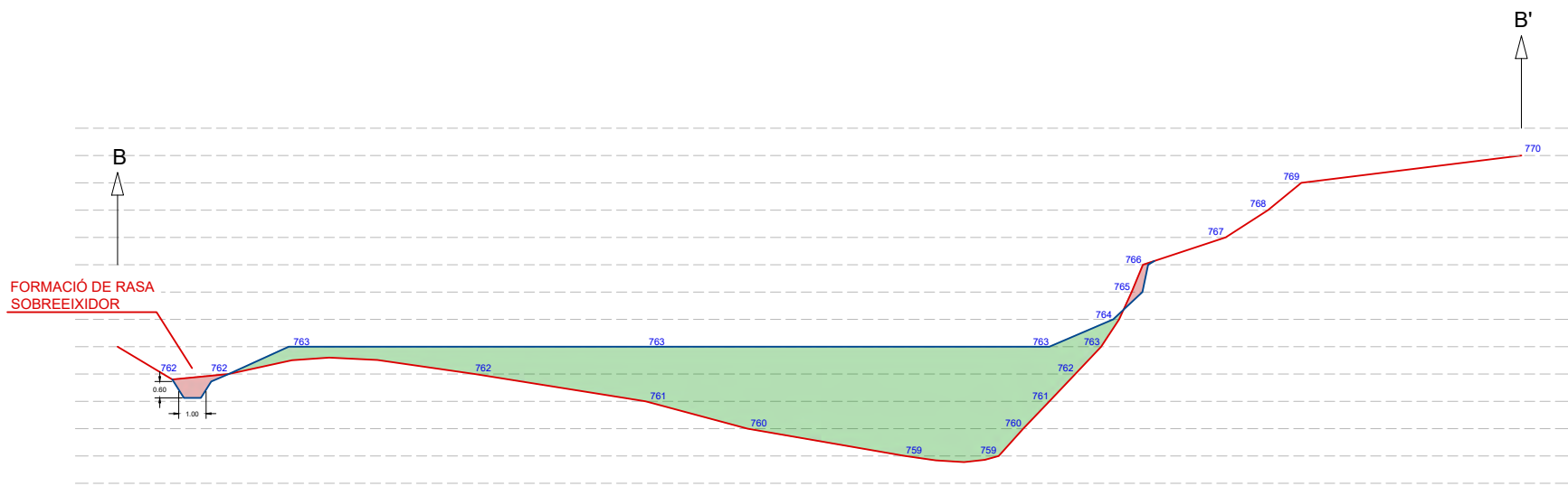
TALL TOPOGRÀFIC B-B' 1:250
