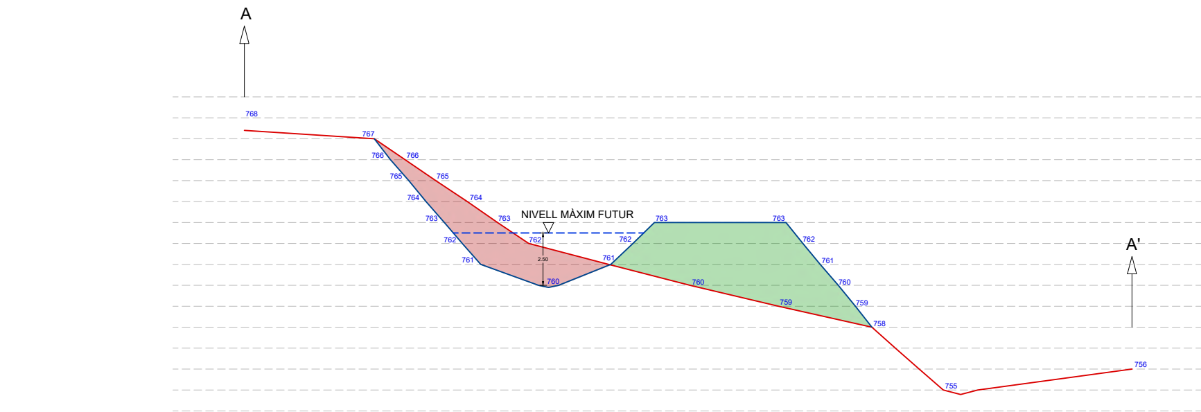
TALL TOPOGRÀFIC A-A' 1:250
