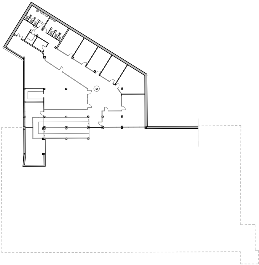
Planta primera
