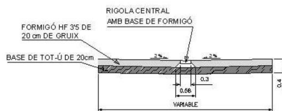
Secció tipus paviment de formigó
