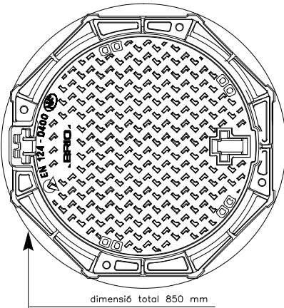
PLANTA TAPA
