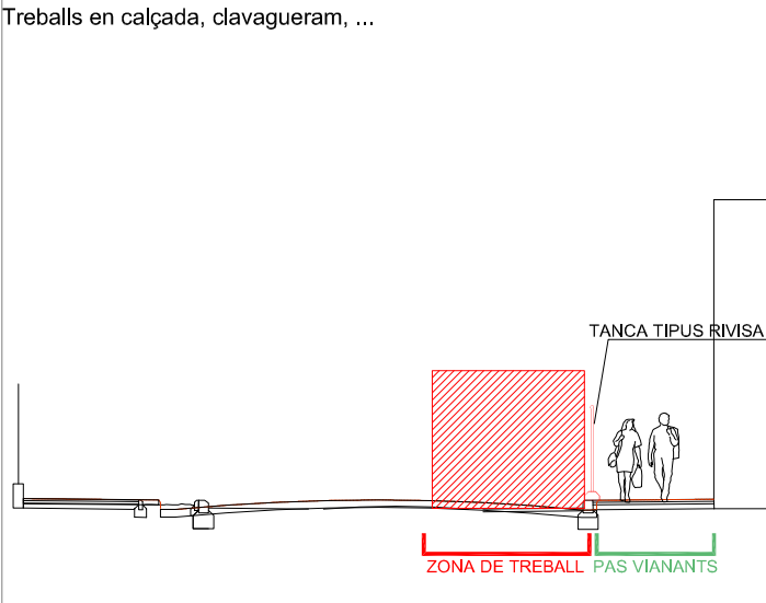
SECCIÓ TIPUS IMPLANTACIÓ. PAS VIANANTS ZONA TREBALLS. FASE 1
