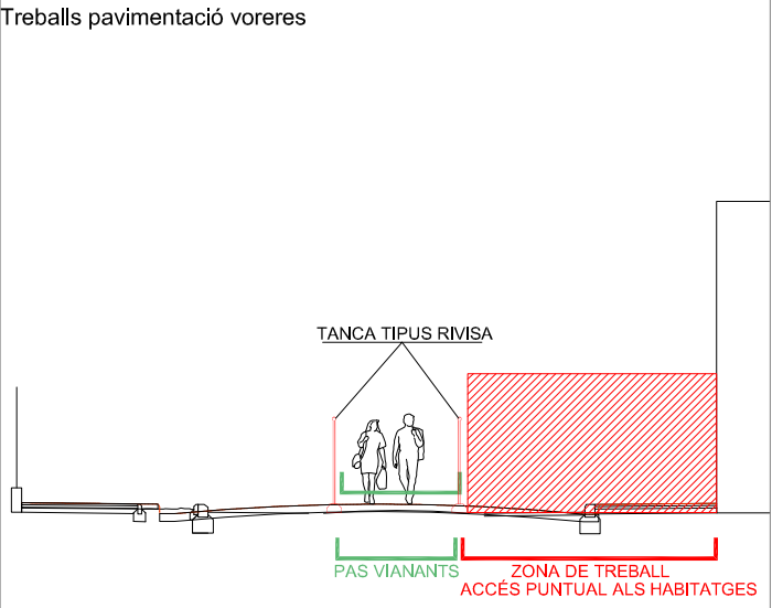
SECCIÓ TIPUS IMPLANTACIÓ. PAS VIANANTS ZONA TREBALLS. FASE 2
