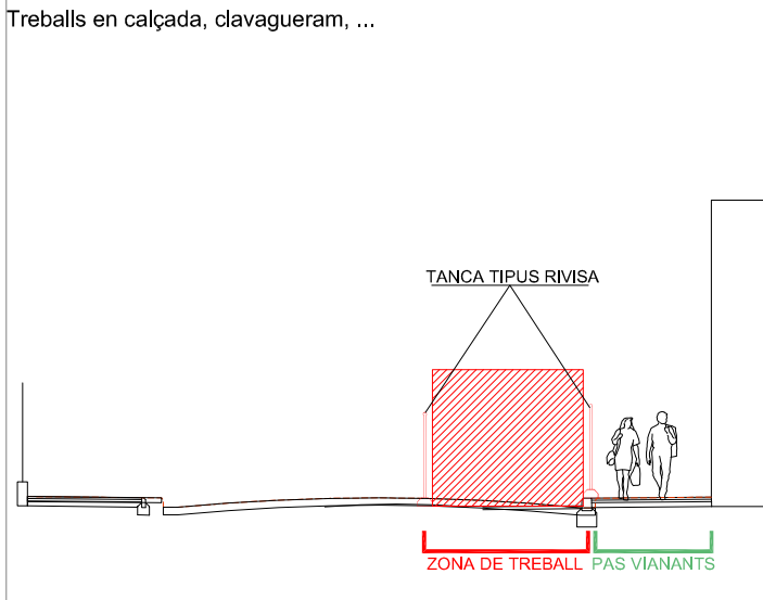
SECCIÓ TIPUS IMPLANTACIÓ. PAS VIANANTS ZONA TREBALLS. FASE 1 Treballs en calçada, clavagueram, ...
