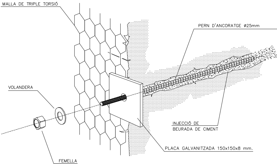
DETALL D'ANCORATGE AMB PLACA SENSE ESCALA
