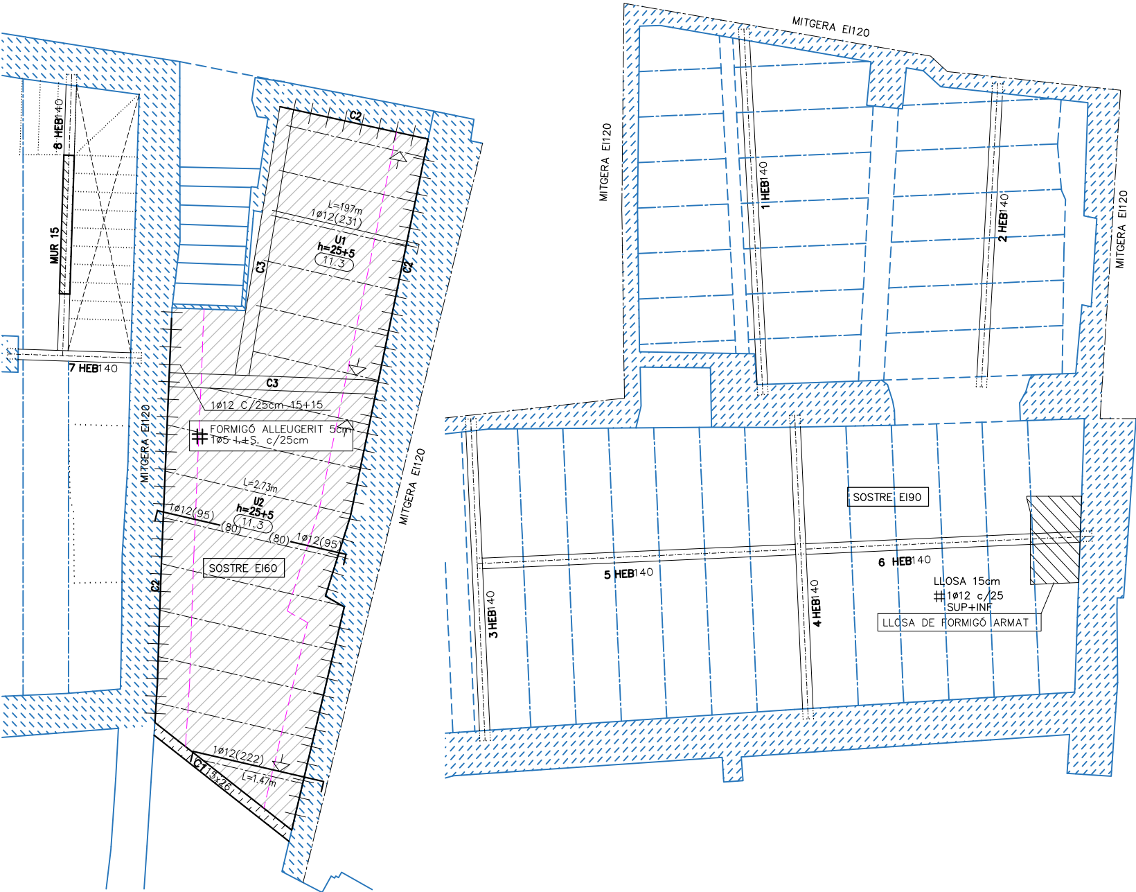
SOSTRE PLANTA BAIXA
