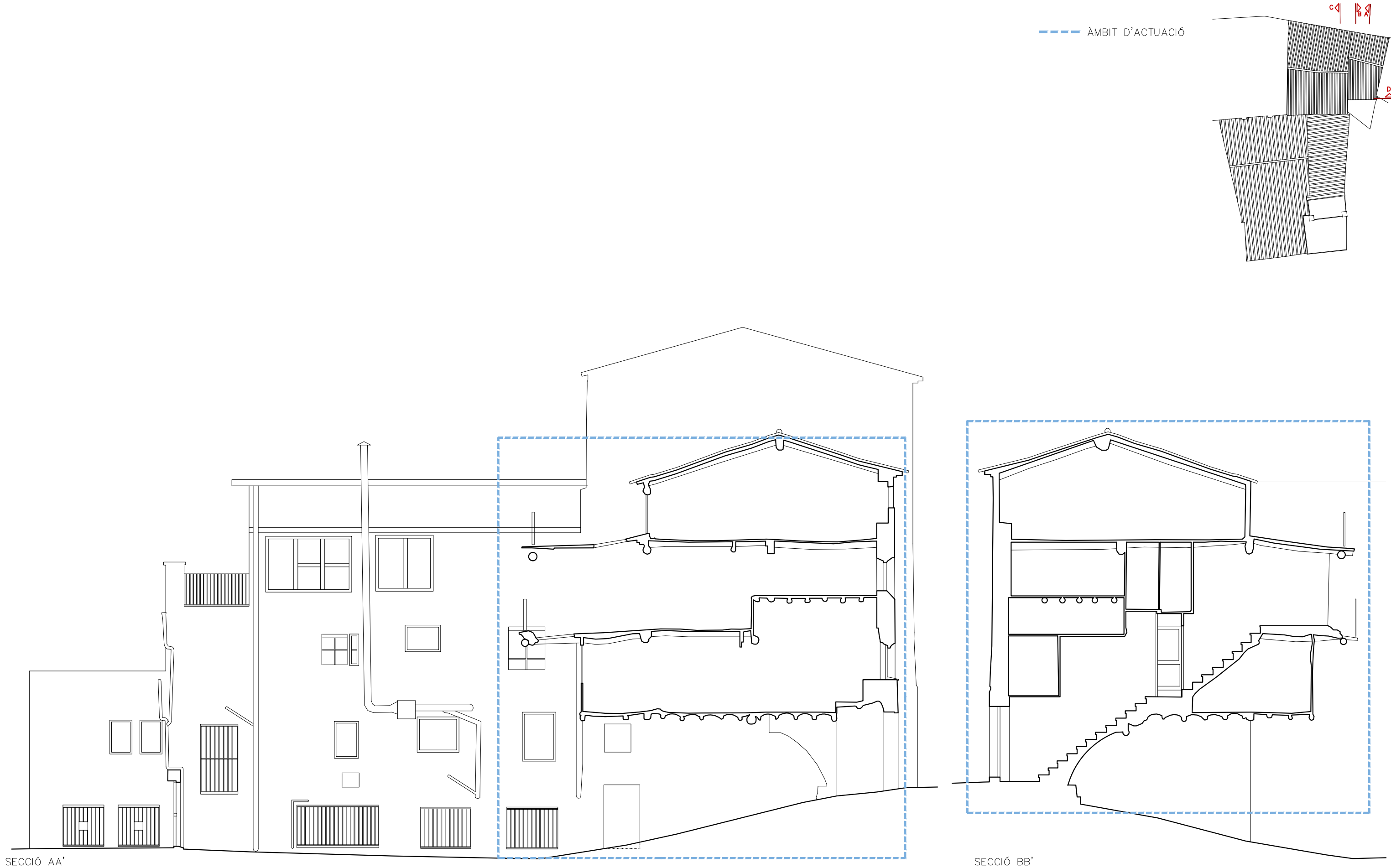
SECCIÓ AA'
