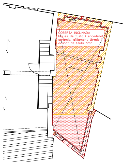
PLANTA TERCERA
