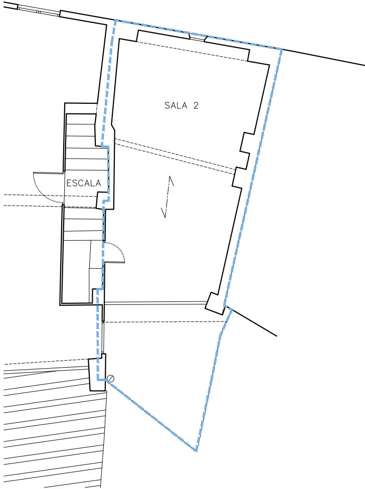
PLANTA GOLFES
