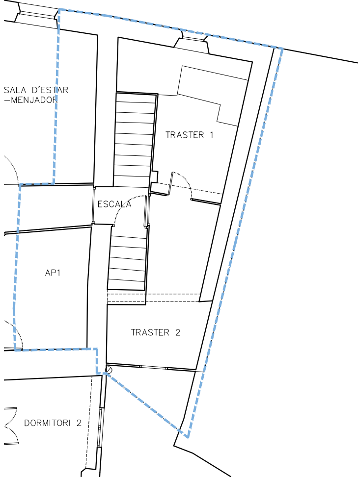
PLANTA PRIMERA
