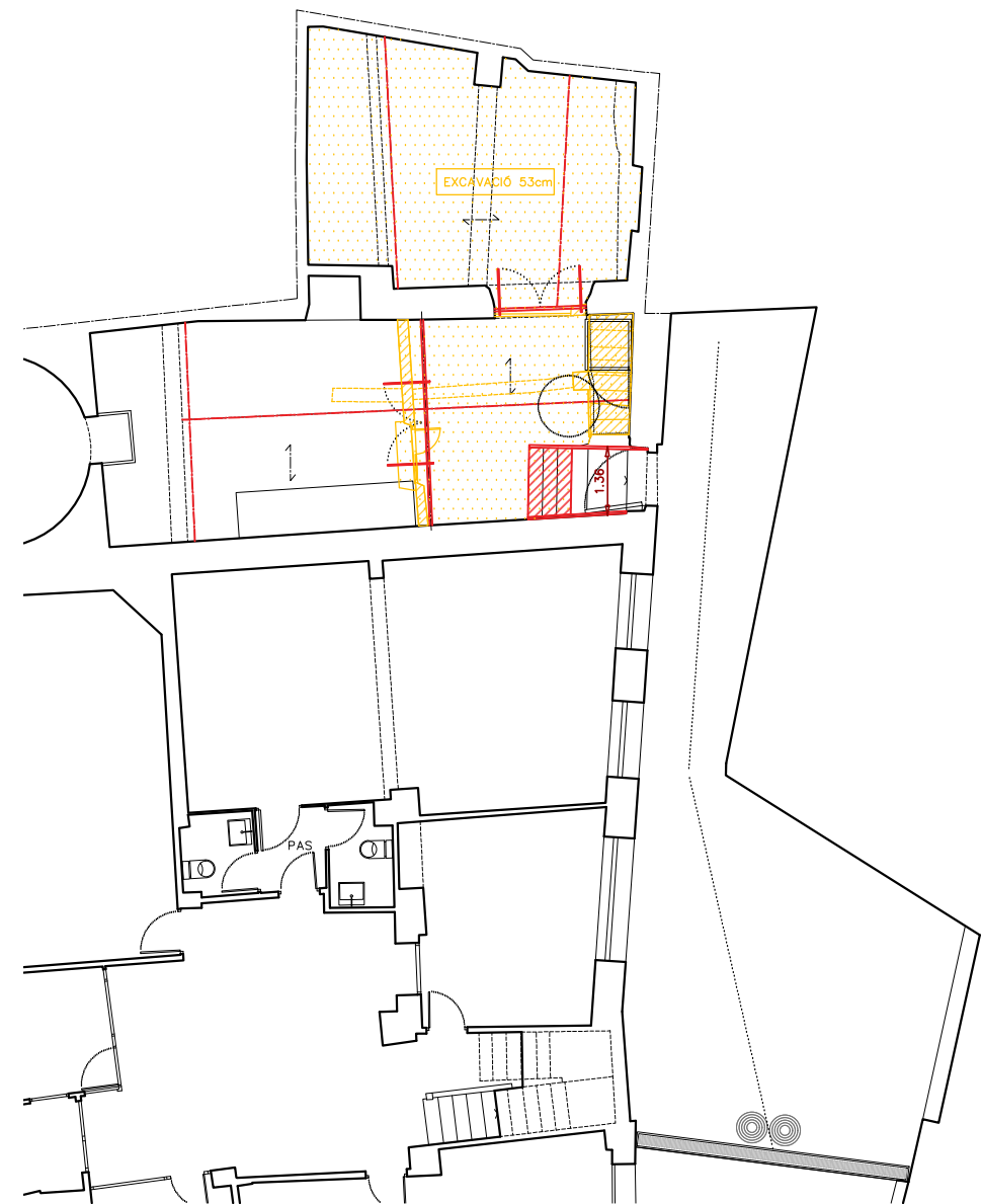
PLANTA SEMI SOTERRANI
