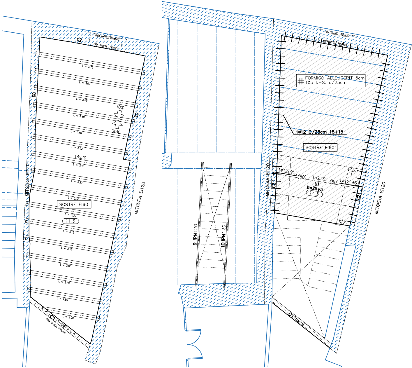
SOSTRE PLANTA SEGONA
