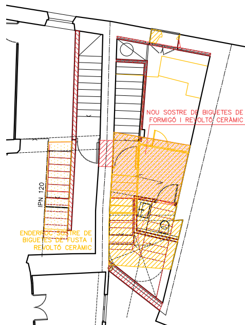
PLANTA PRIMERA
