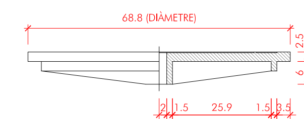
SECCIÓ B-B
