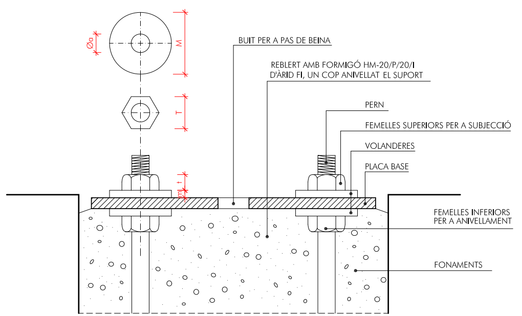
DETALL FONAMENT BÀCUL TIPUS I PRESA DE TERRA
