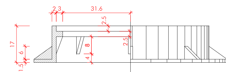
SECCIÓ A-A
