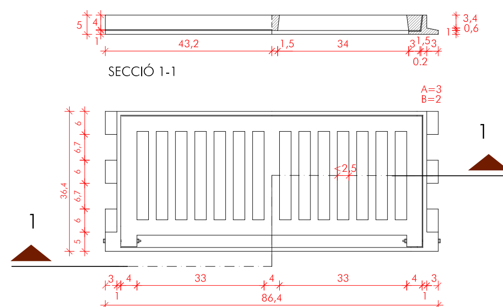
PLANTA
