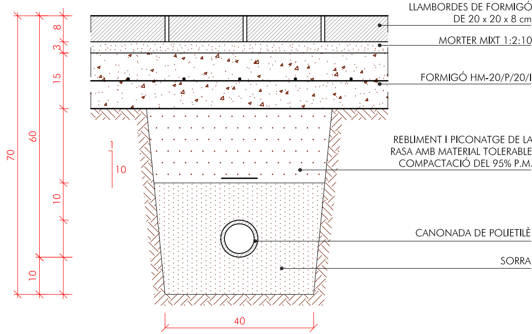
RASA TIPUS CANALITZACIÓ D'AIGUA
