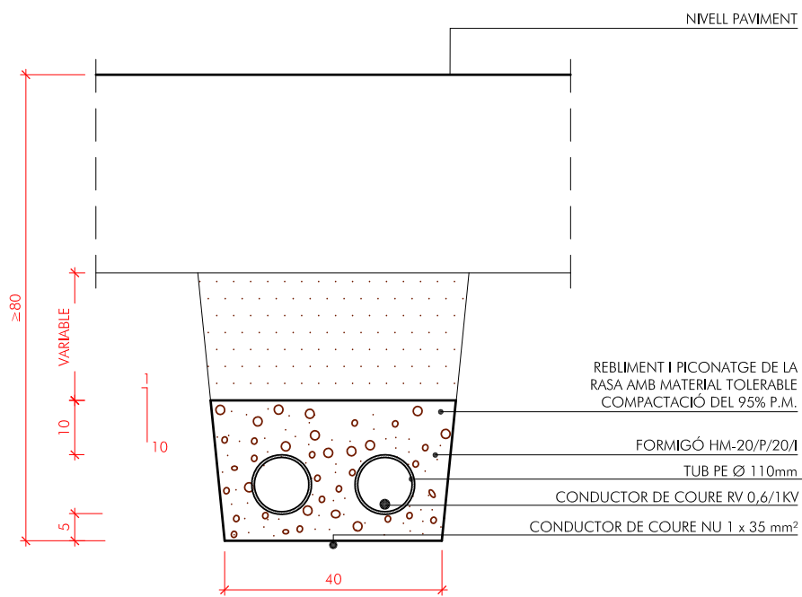
RASA TIPUS PER A ENCANONAR CABLES SOTA CALÇADA
