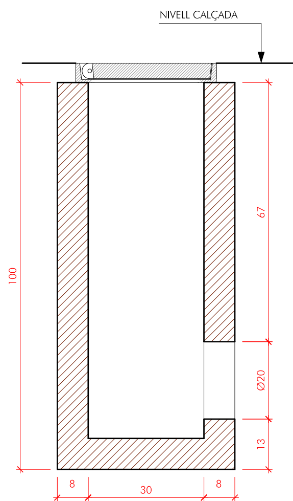
SECCIÓ A-A
