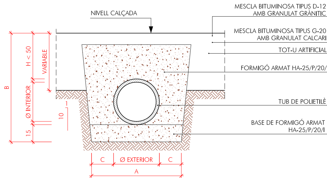
RASA TIPUS H < 50 E: 1/20
