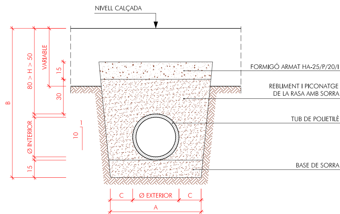
RASA TIPUS H > 50 i H < 80 E: 1/20
