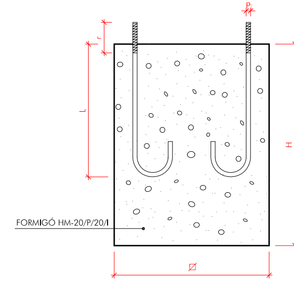
FONAMENTS I PERNS
