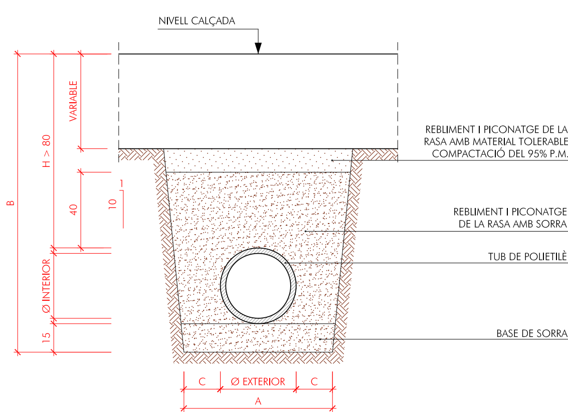
RASA TIPUS H > 80 E: 1/20
