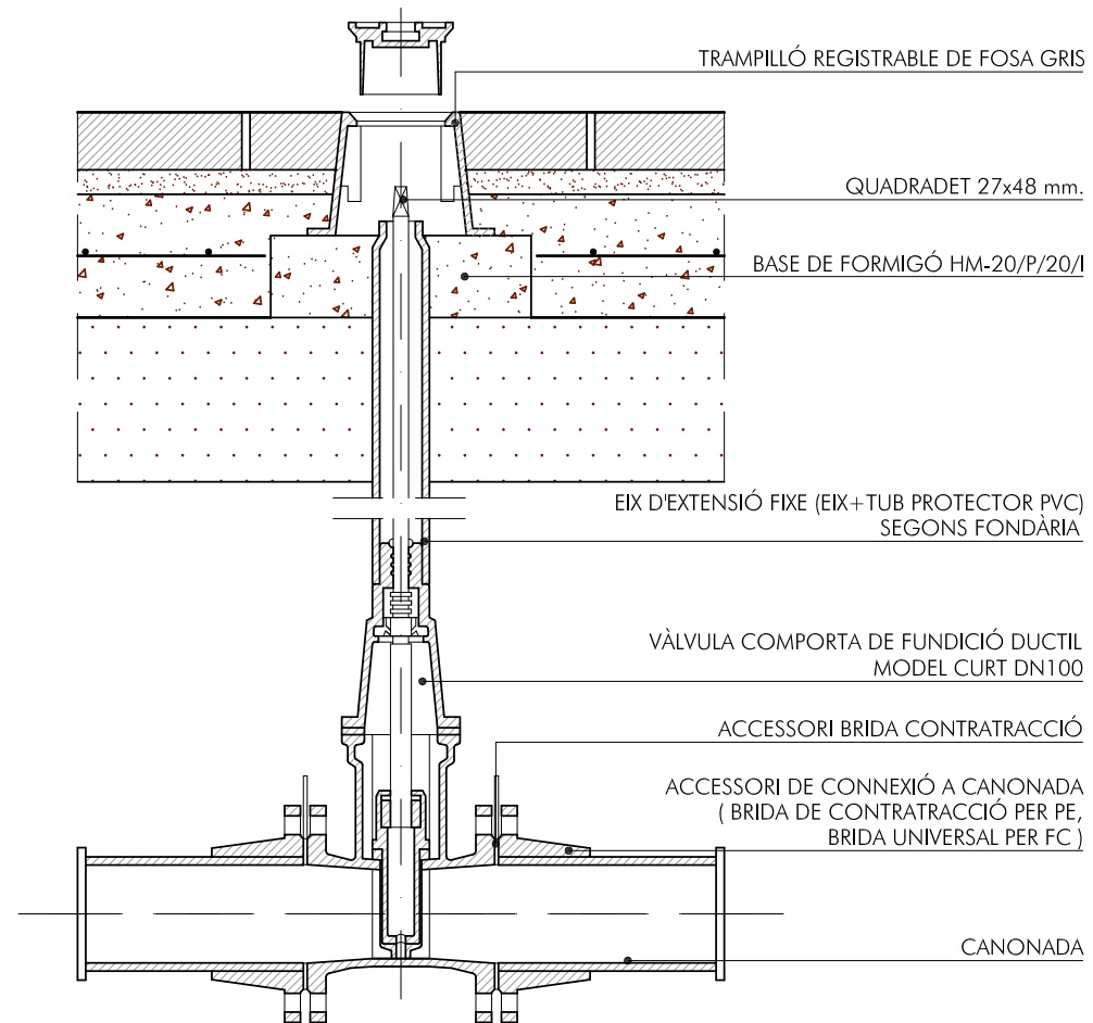
VÀLVULA PER A CANONADES DE POLIETILÈ I FIBROCIMENT
