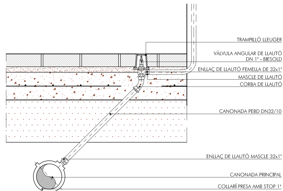
ESCOMESA D'AIGUA D'1" ( 3/4" - 1.1/2" )
