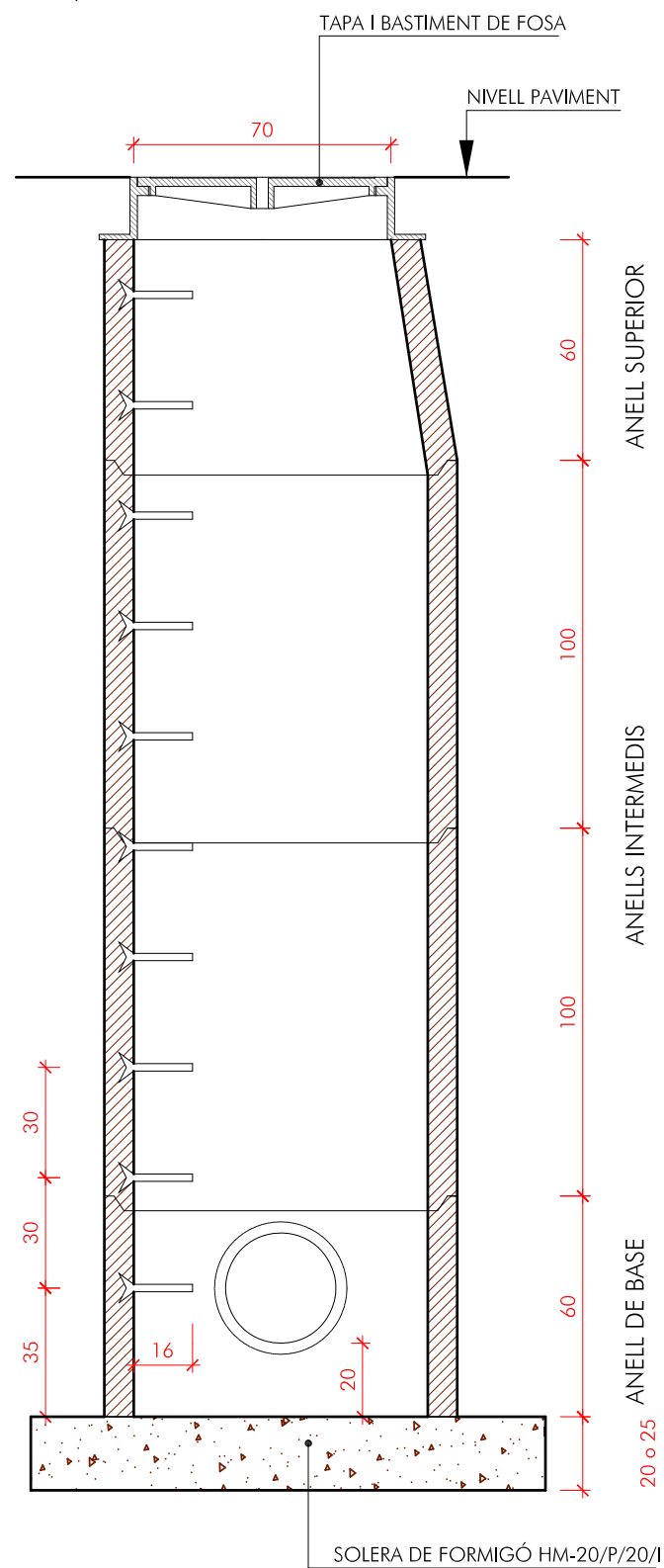
SECCIÓ A-A
