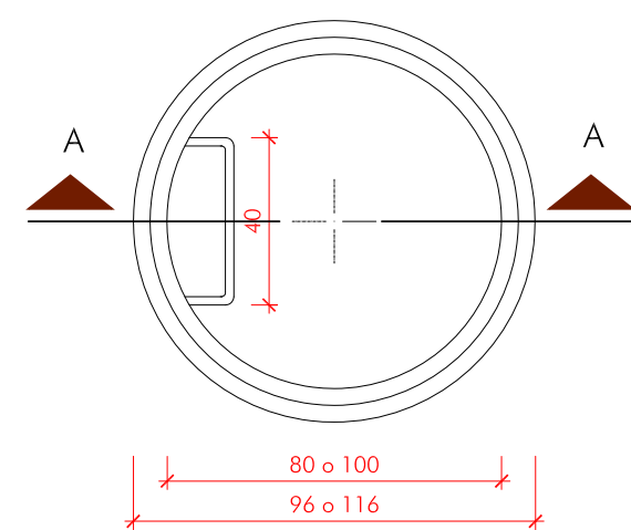
PLANTA ANELL INTERMEDIS
