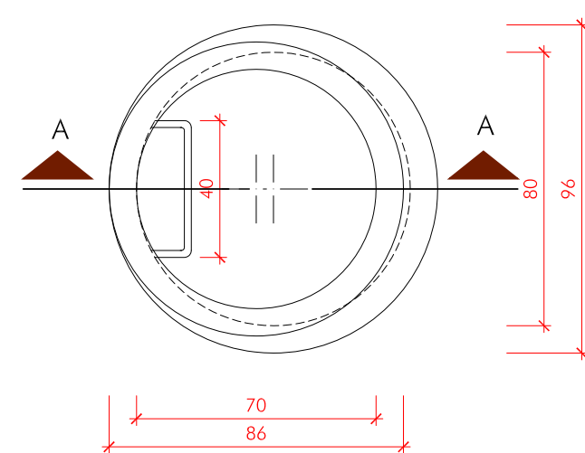
PLANTA ANELL SUPERIOR
