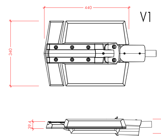
LLUMENERA V-MAX DE CARANDINI O SIMILAR
