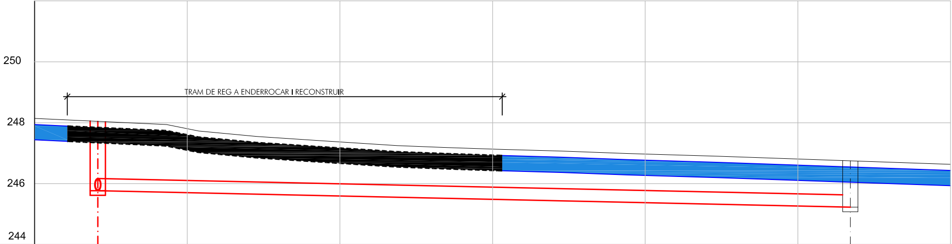
Perfil Longitudinal: Carrer Montseny Escala - V: 250 H:100
