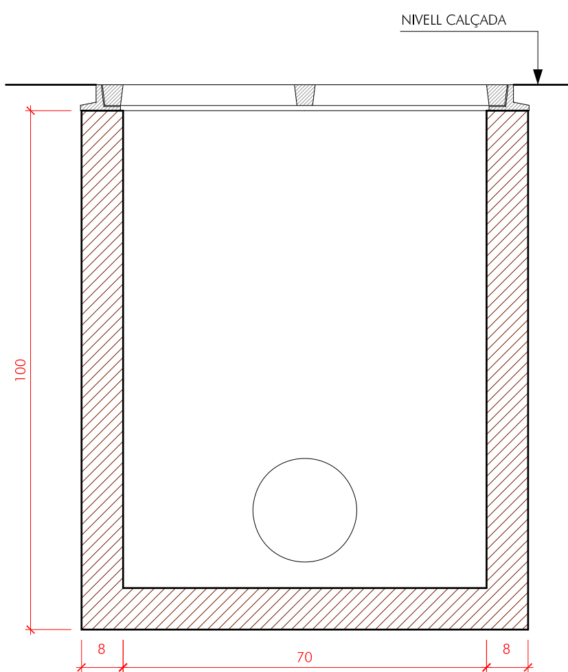
SECCIÓ B-B
