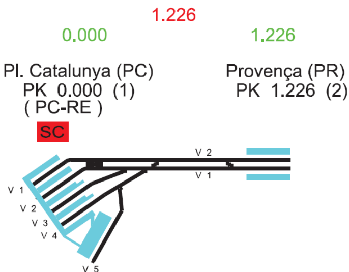
Fig 1. Esquema túnel PC-PR.
