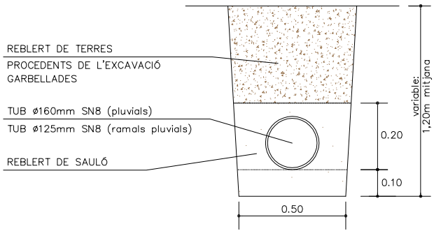
SECCIÓ TIPUS RASA SISTEMA DE PLUVIALS
