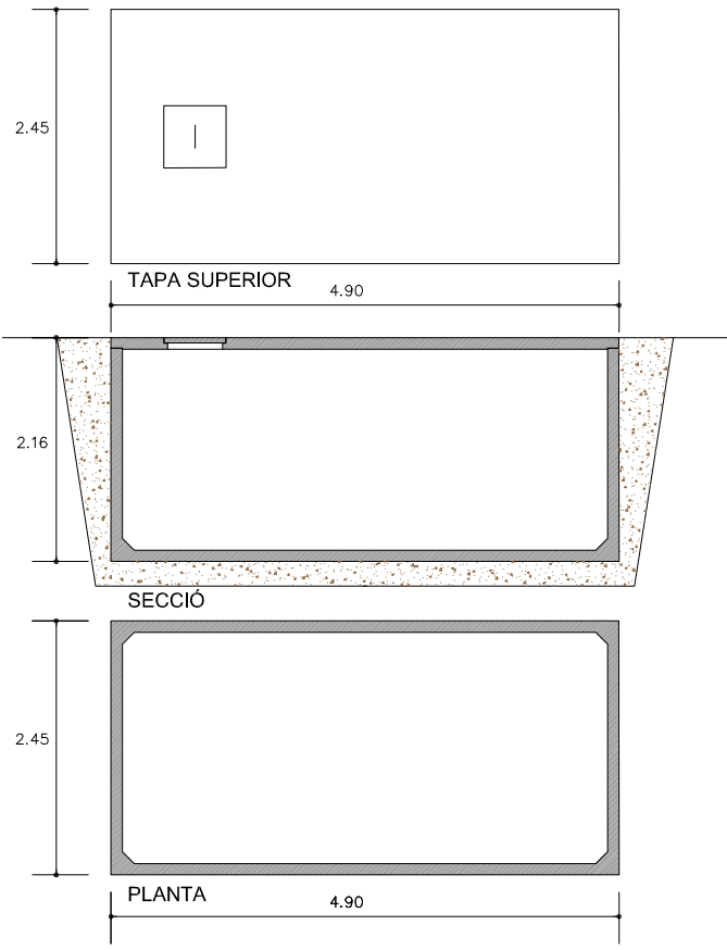
DIPÒSIT PREFABRICAT DE FORMIGÓ 20m 3 disposició horitzontal
