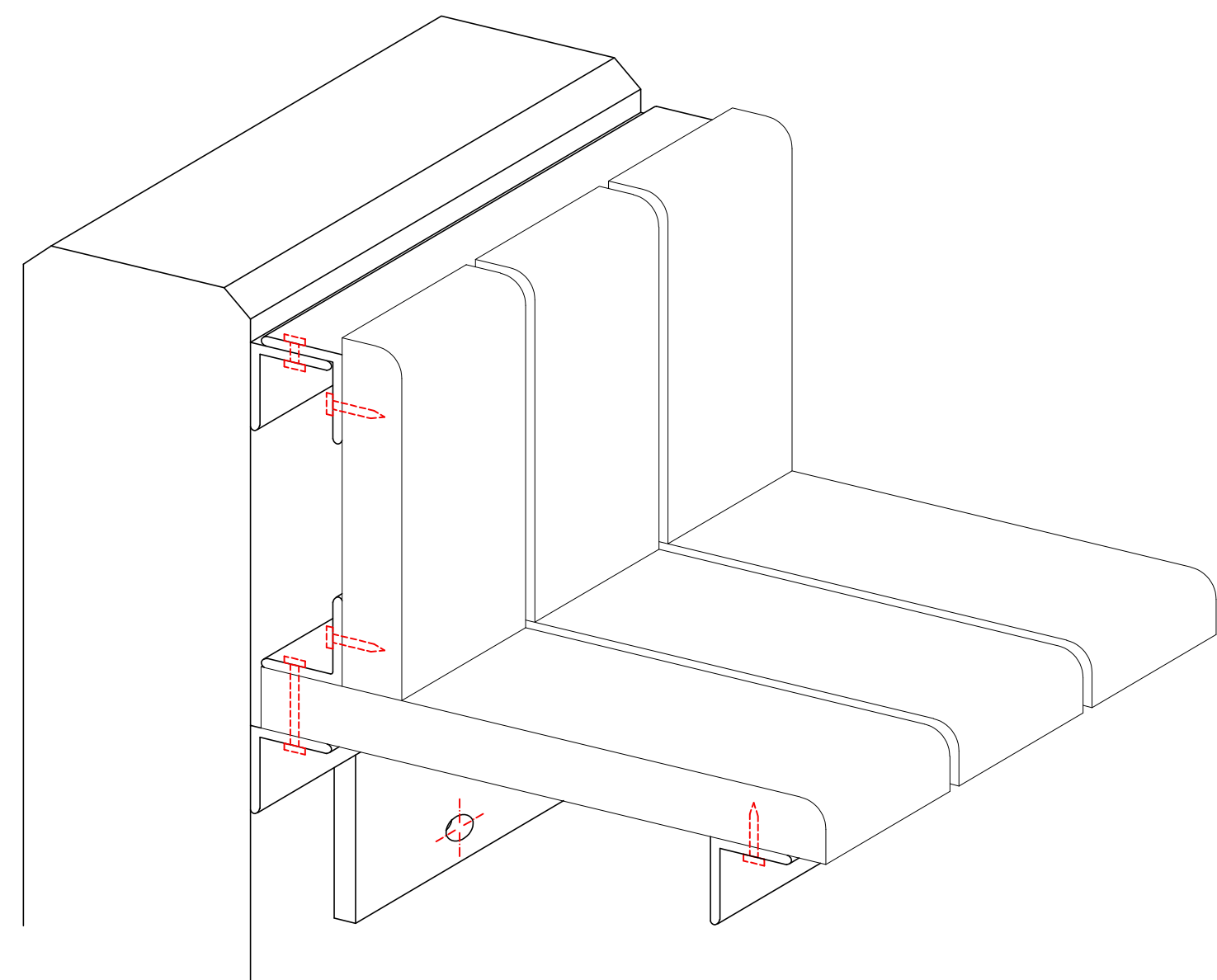
DETALL SEIENT AMB RESPATLLER
