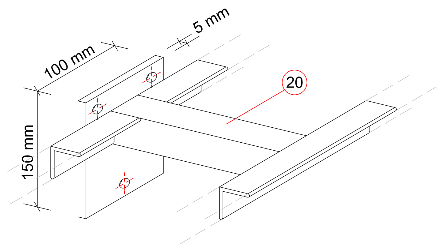
DETALL ANCLATGE
