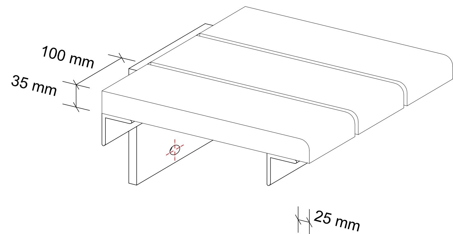
DETALL SEIENT SENSE RESPATLLER
