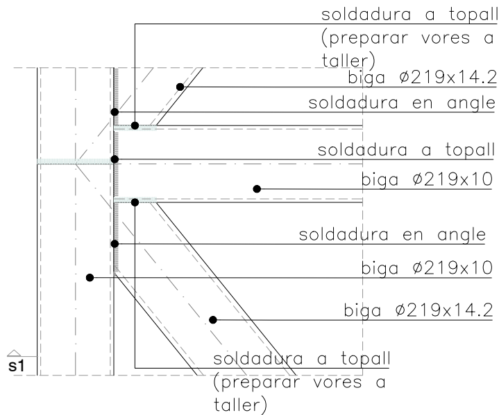
PLANTA DET S.02 Detall unió entre bigues i diagonals
