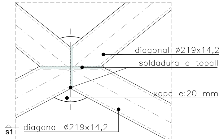
PLANTA DET S.01 Detall realzament bigues sobre pilars
