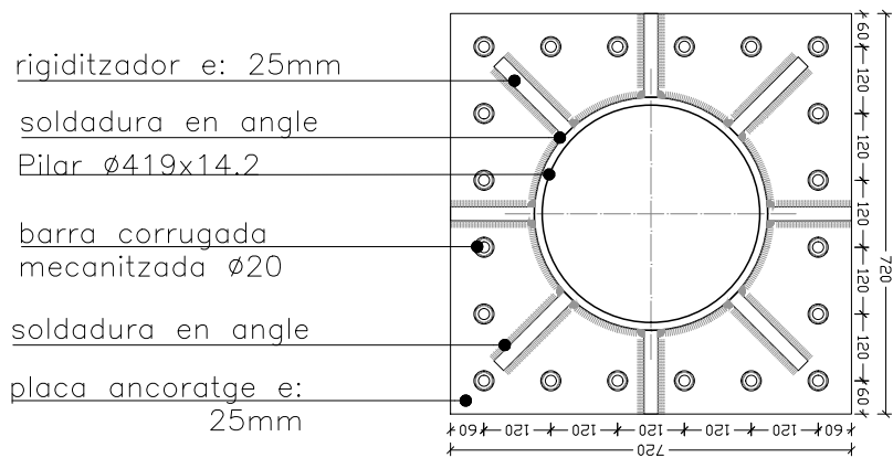
PLANTA DET F.01 Detall placa ancoratge nous pilars
