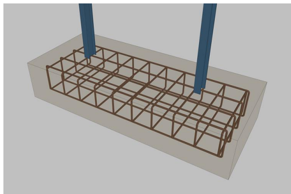
Figura 4. Fonamentació tipus (Cybe 3D)
