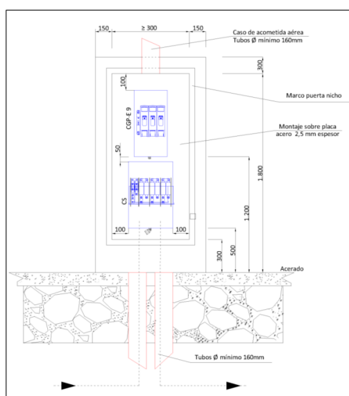
Figura 3. Instal·lació CGP y CS montaje vertical. Alzado.
