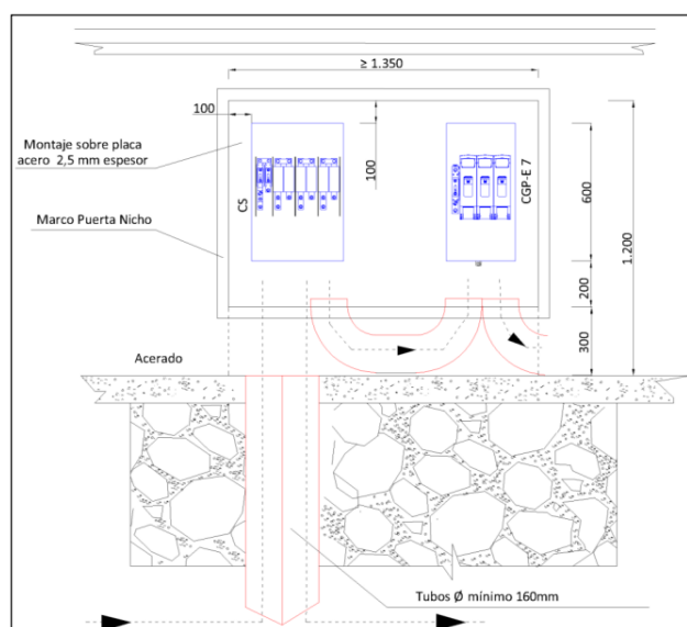
Figura 6. Instal·lació CGP y CS montaje horizontal. Alzado.
