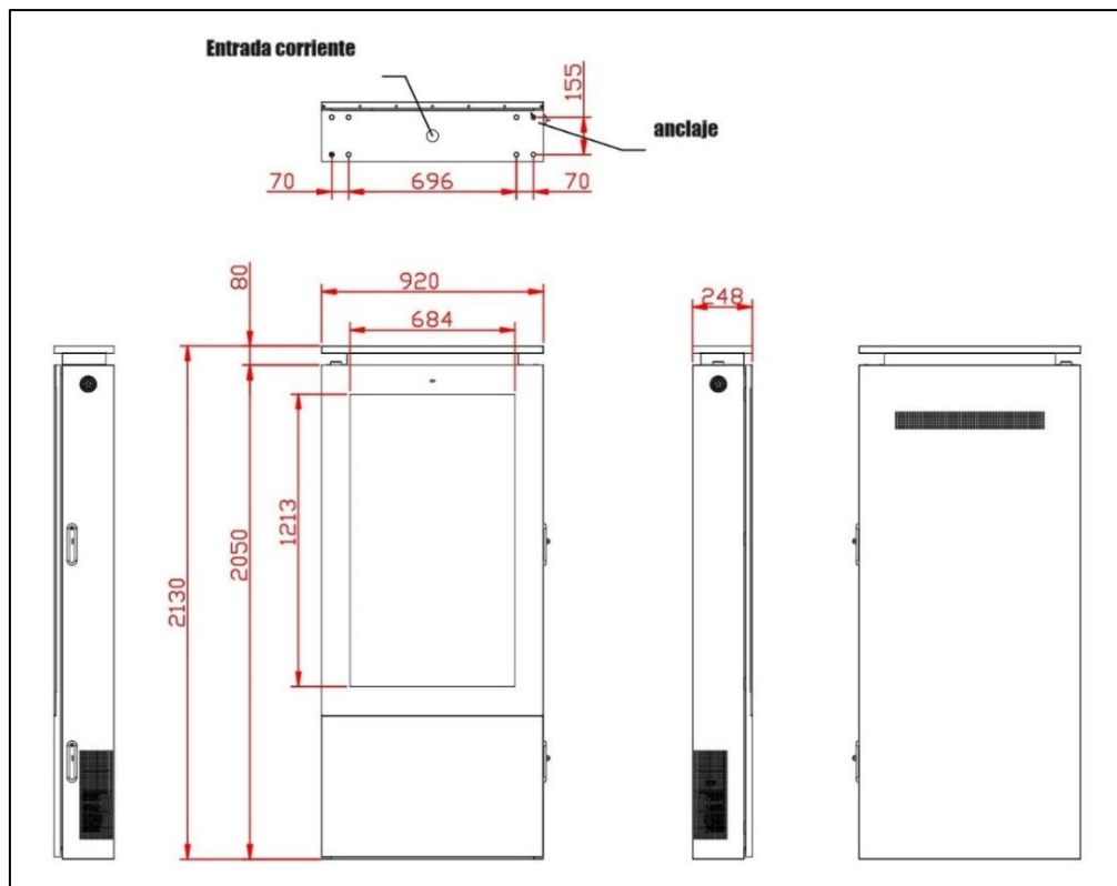
Figura 2. Esquema tòtem, model EC-OK-55
