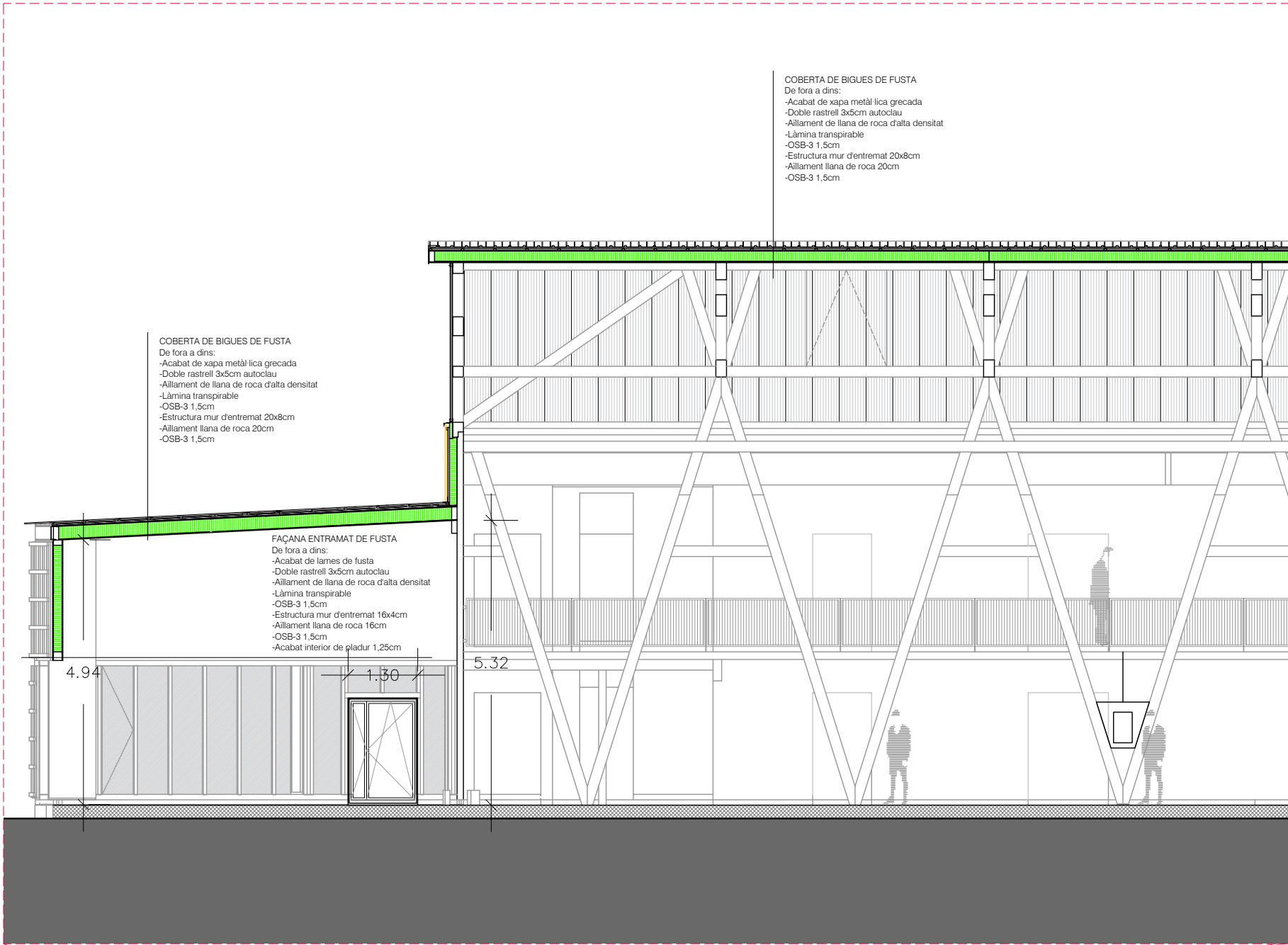
SECCIÓ DETALL ESCALA 1.50
