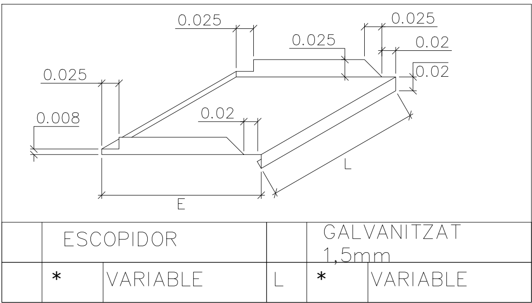
DETALL GENÈRIC ESCUPIDOR
