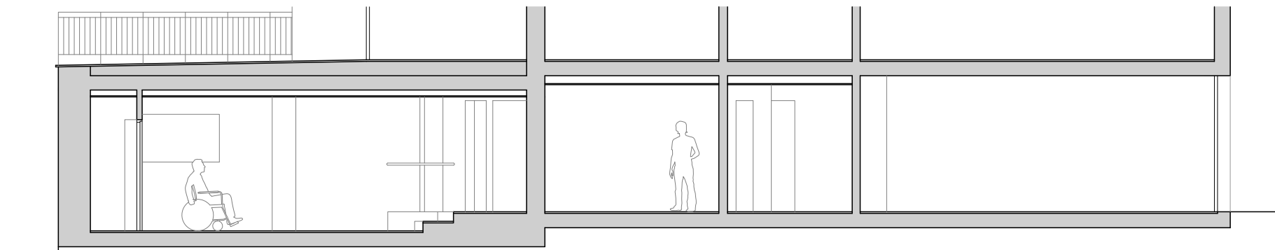
SECCIO LONGITUDINAL SL3
