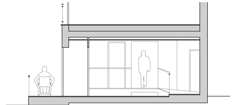
SECCIO TRANSVERSAL ST1
